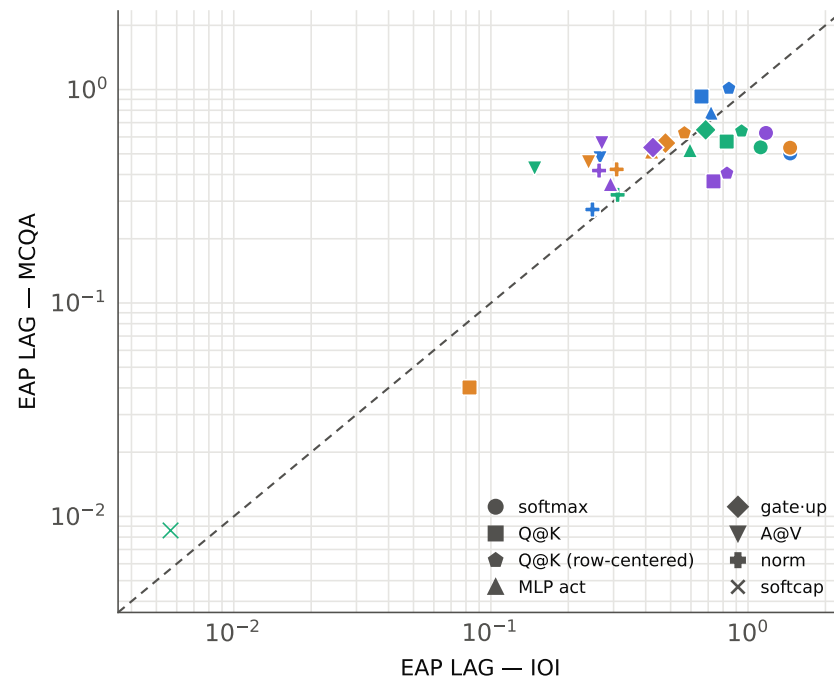
(d) task effect: same op, MCQA vs IOI (marker = op, color = model)
