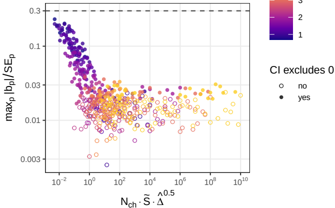
D bias per parameter, worst
