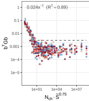
A bias: b^T G b
