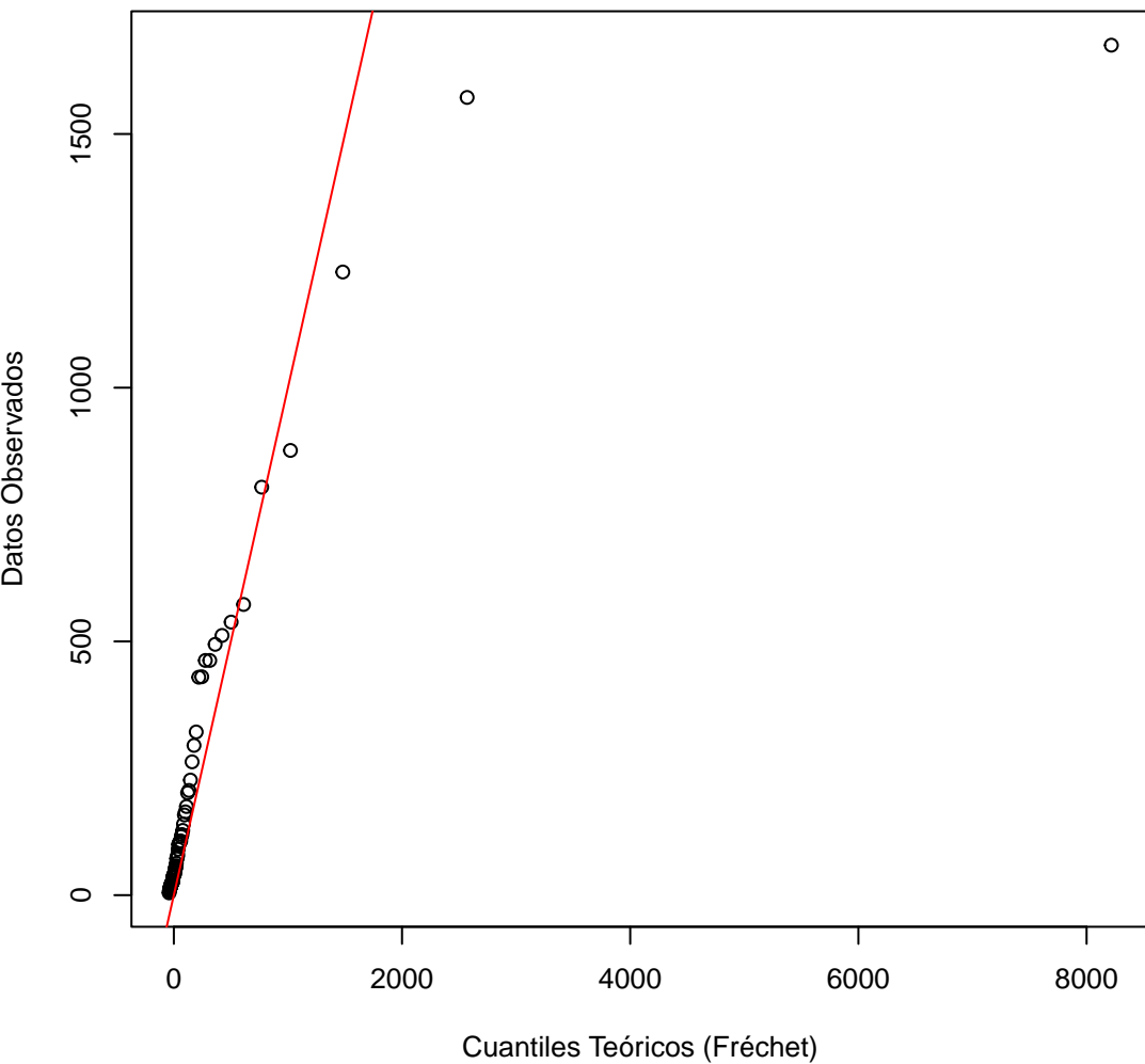
Q-Q Plot para la Distribución Fréchet Ajustada
