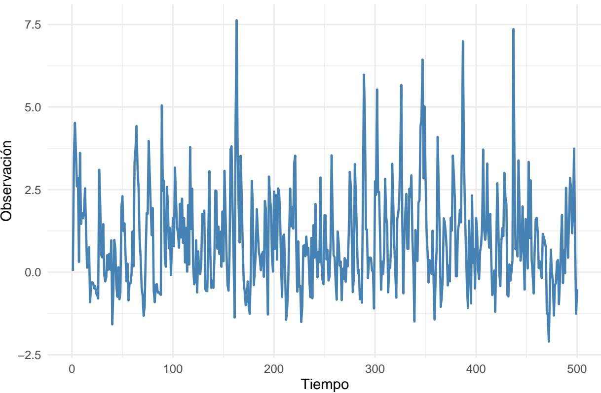
Proceso 2-dependiente estacionario con datos Gumbel
