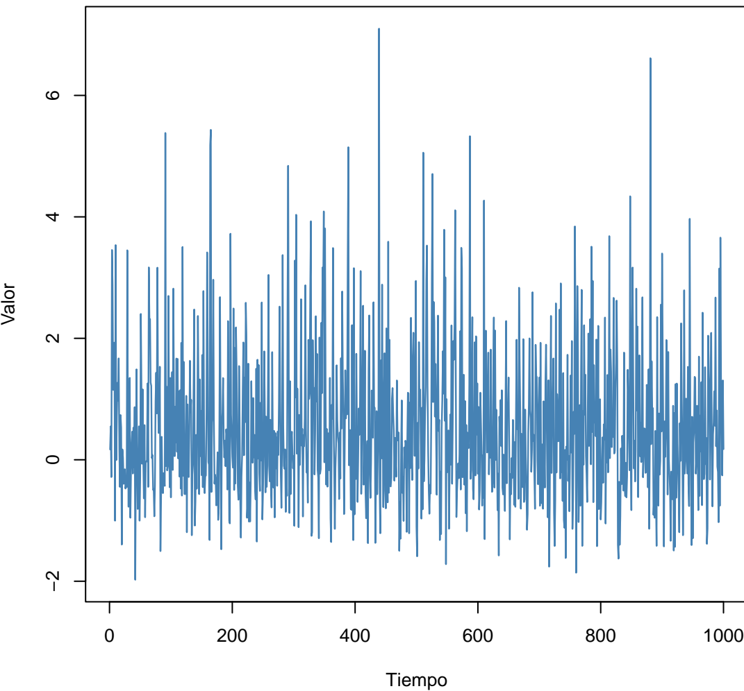
Datos iid con distribución Gumbel simulados como serie temporal
