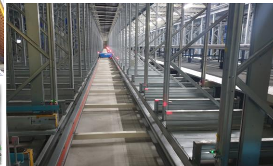
보관 Rack
