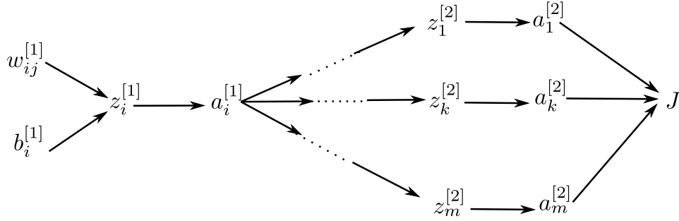
Figura 6.18: Graf computațional pentru neuronul i din stratul ascuns. Ponderile instruibile w_{ij}^{[1]} și b_i^{[1]} contribuie la valoarea funcției de eroare prin mai multe căi, via z_1^{[2]}, \dots, z_m^{[2]} . Situația e similară cu cea din figura 6.10.
