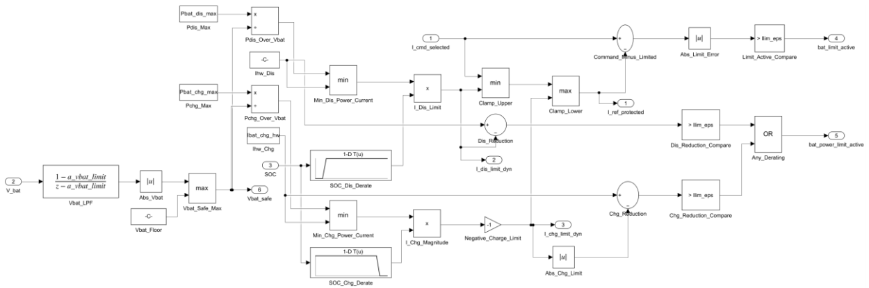
图1 Battery_Reference_Protection 自动布局后的标准块接线
