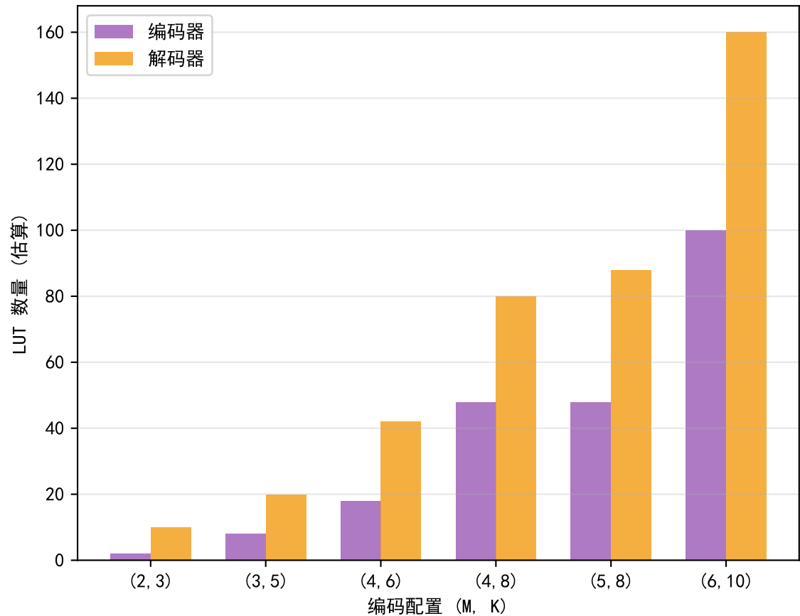
CS-FEC 编解码器资源分布
