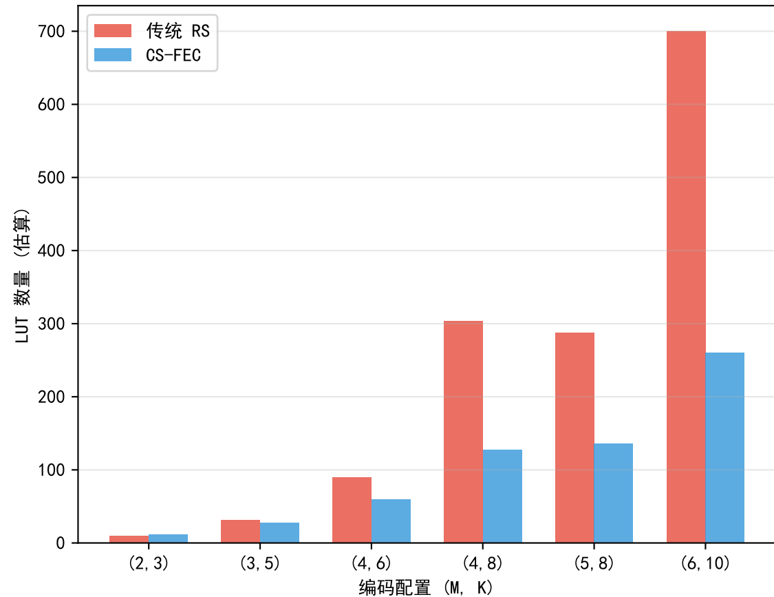
FPGA LUT 资源对比
