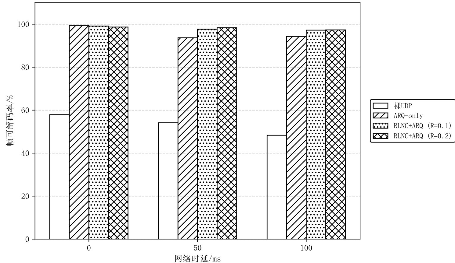
(c) 不同时延下的帧可解码率（丢包率=10%）
