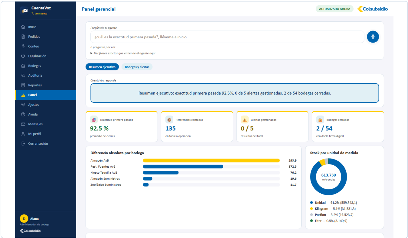
FIGURA 16 Panel · Resumen ejecutivo.
