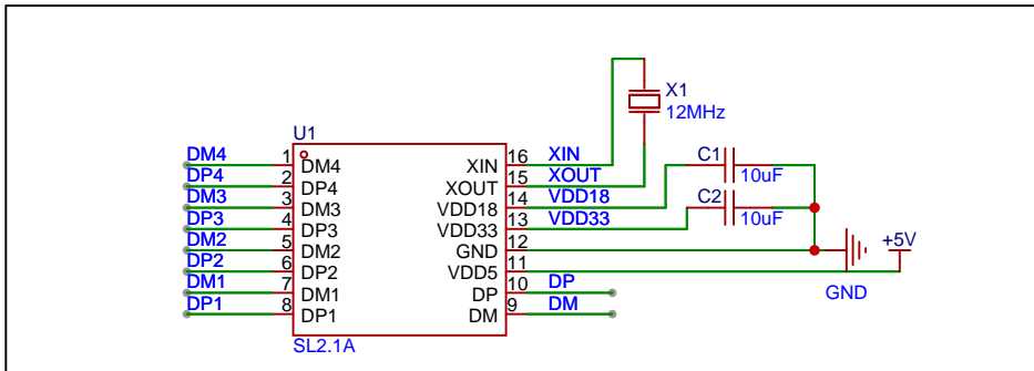
拓展电路
