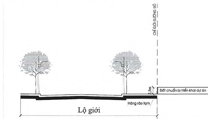
Hình 14: Tường rào xây dựng tạm cho dự án chuẩn bị triển khai
