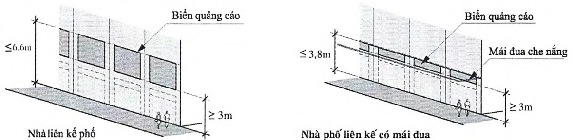
Hình 12: Quy định quảng cáo đối với nhà liên kế phố
