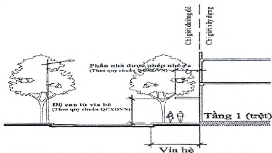
Hình 16: Hình minh họa mái đón, mái hè phố
