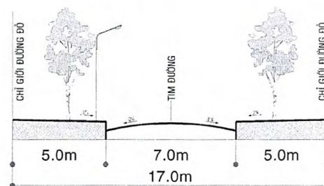
MẶT CẮT 4-4, LG: 17M
