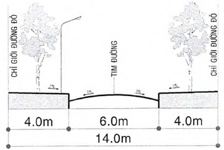
MẶT CẮT 6-6, LG: 14M
