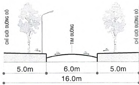
MẶT CẮT 5-5, LG: 16M
