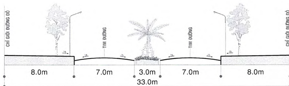
MẶT CẮT 1-1, LG:33M
