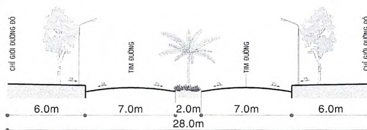
MẶT CẮT 2-2, LG:28M
