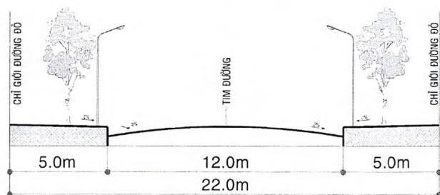
MẶT CẮT 3-3, LG: 22M
