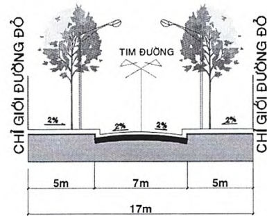
MẶT CẮT 4-4
