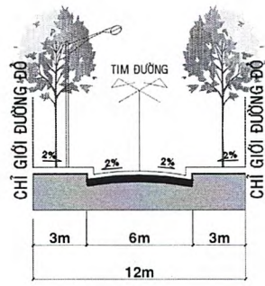
MẶT CẮT 7-7
