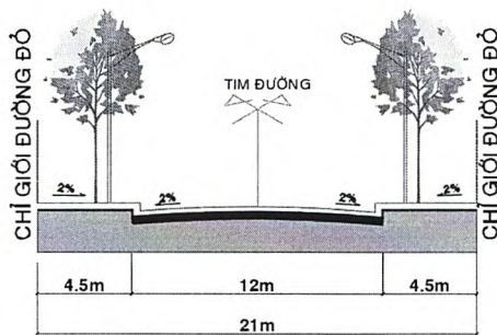
MẶT CẮT 3-3
