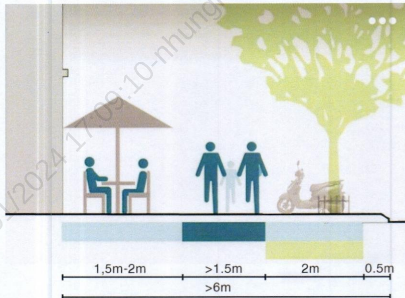
Minh họa mặt cắt không gian vỉa hè
