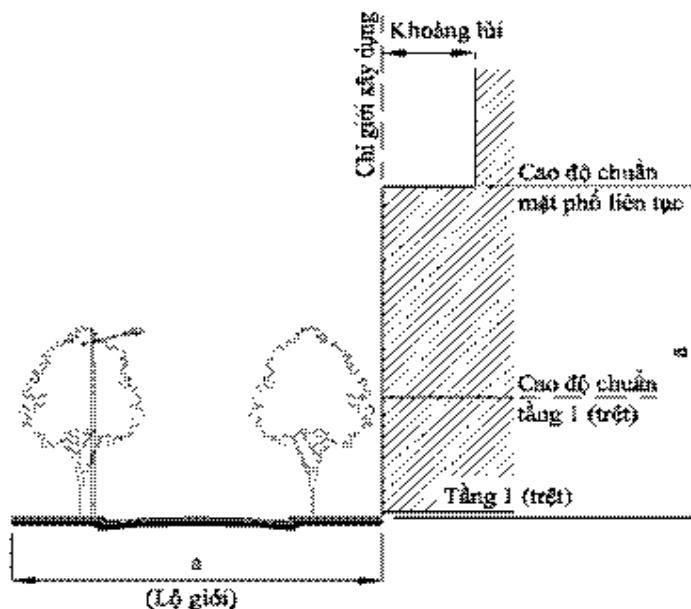
Hình 2.2. Minh họa về khoảng lùi xây dựng công trình
