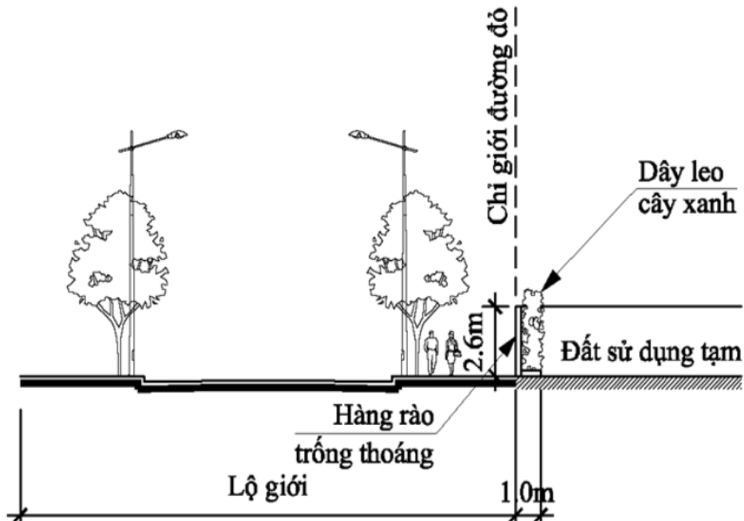
Hình 2.8: Sơ đồ minh họa hàng rào dự án, công trình chưa triển khai
