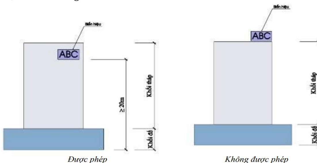
Hình 2.7: Minh họa quy định về biển hiệu
