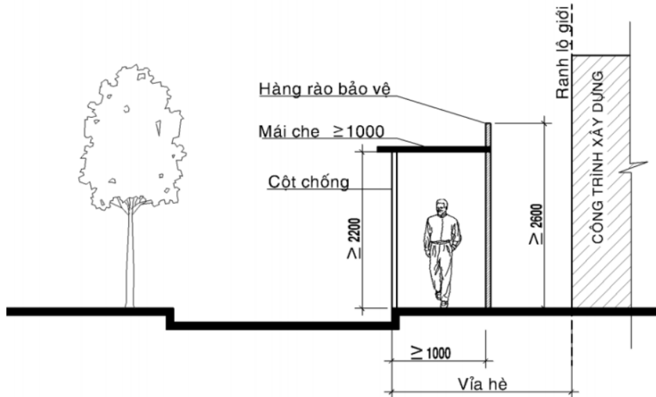
Hình 2.10: Sơ đồ minh họa hàng rào của công trình xây dựng sát ranh lộ giới
