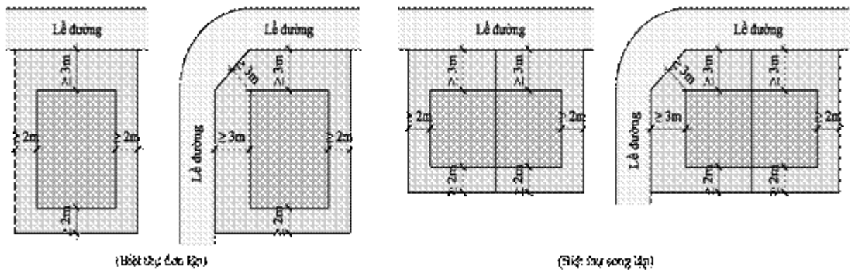
Hình 2.5. Minh họa quy định về khoảng lùi tối thiểu của công trình biệt thự
