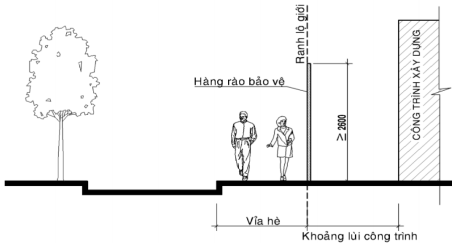
Hình 2.9: Sơ đồ minh họa hàng rào của công trình xây dựng có khoảng lùi
