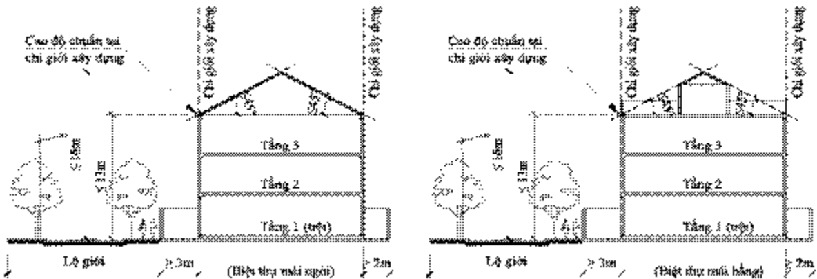
Hình 2.6: Minh họa quy định về số tầng nhà và chiều cao công trình
