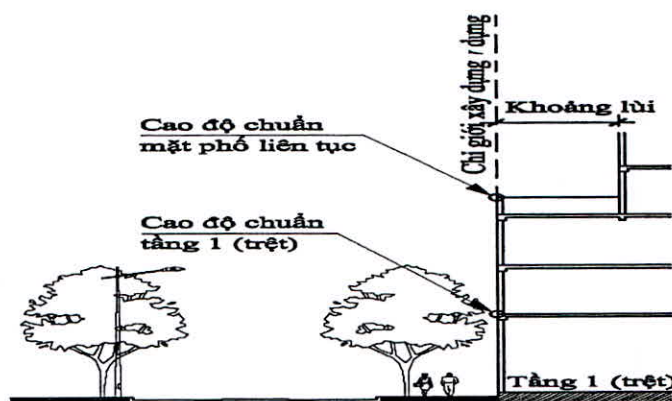
Chiều cao nhà mặt phố liên tục
