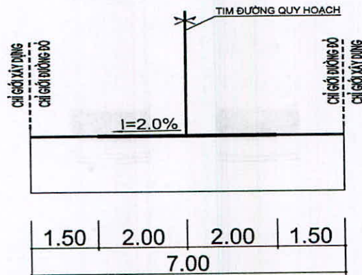
MẶT CẮT 5-5-MẶT CẮT NGANG ĐIỂN HÌNH ĐƯỜNG LIÊN XÃ
