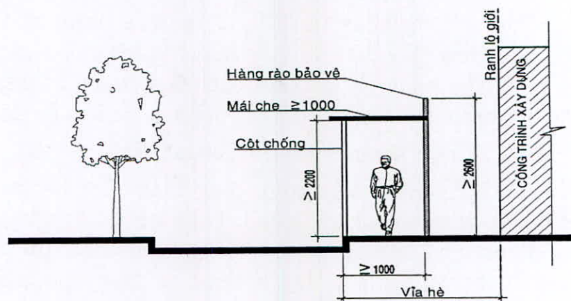
Hàng rào của công trình xây dựng sát ranh lộ giới
