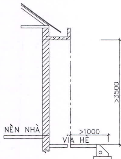
b) Trường hợp phần đua ra là sê nô, ô văng và mái dốc
