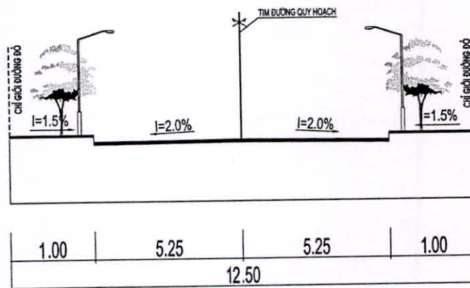
MẶT CẮT 1-1 : MẶT CẮT NGANG ĐIỂN HÌNH ĐOẠN KHÔNG QUA ĐÔ THỊ
