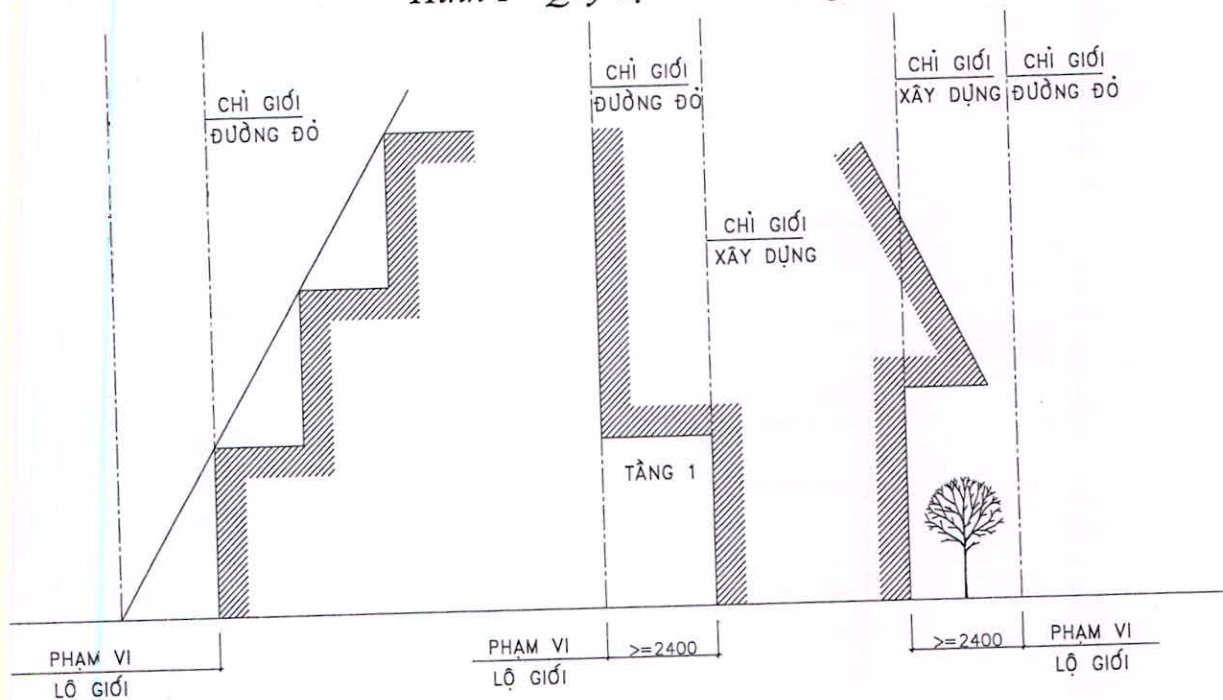
Hình 1 - Quy định về khoảng lùi
