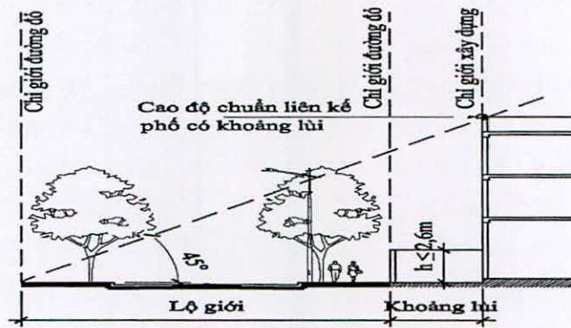
Cao độ chuẩn nhà liên kế phố có khoảng lùi
