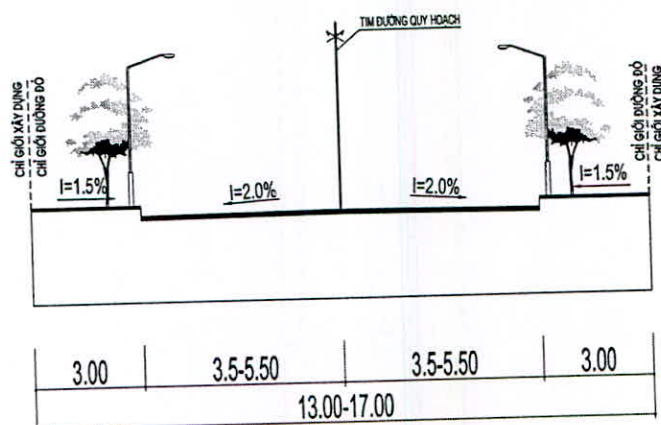
MẶT CẮT 2*2*-MẶT CẮT NGANG ĐIỂN HÌNH ĐƯỜNG LIÊN KHU VỰC
