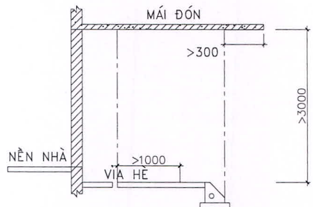
a) Phần đua ra của mái đón
