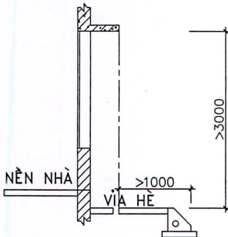
c) Trường hợp phần đua ra là ô văng của sổ
