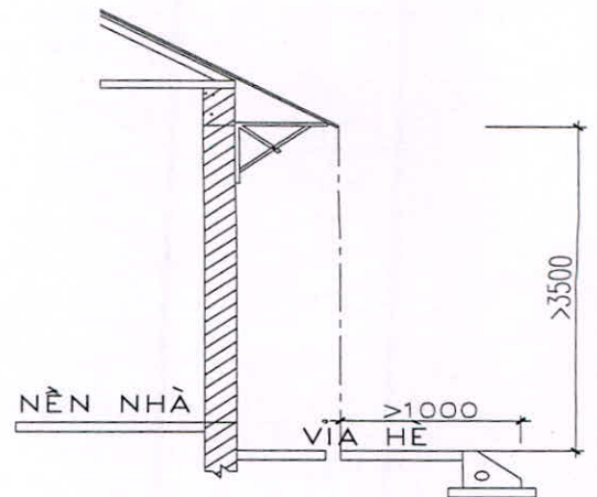
d) Trường hợp phần đua ra là con sơn mái dốc
