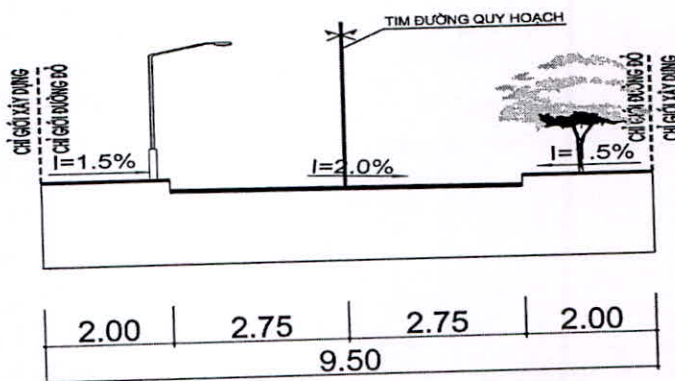
MẶT CẮT 4-4-MẶT CẮT NGANG ĐIỂN HÌNH ĐƯỜNG KHU VỰC
