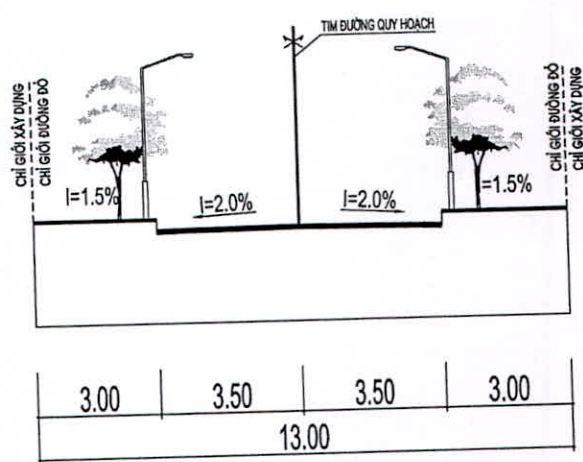
MẶT CẮT 3-3-MẶT CẮT NGANG ĐIỂN HÌNH ĐƯỜNG CHÍNH KHU VỰC
