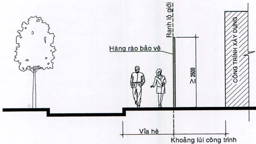
Hàng rào của công trình xây dựng có khoảng lùi
