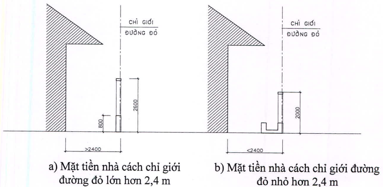
Hình 6 - Quy định cổng, hàng rào
