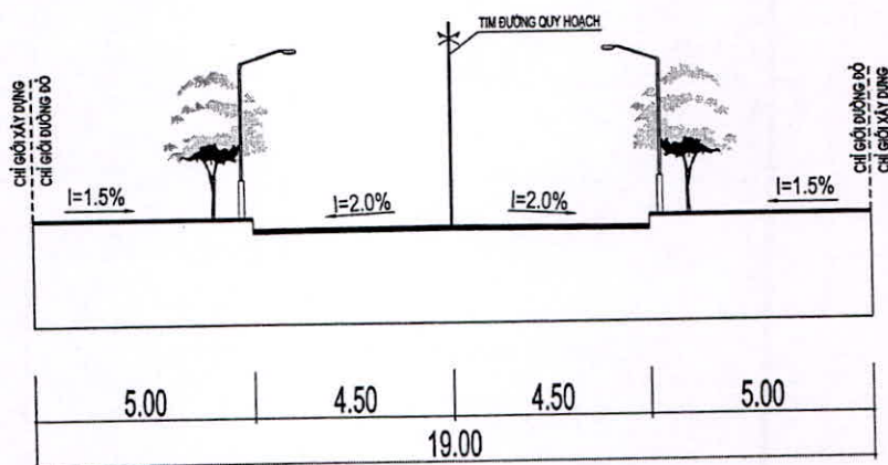
MẶT CẮT 6-6-MẶT CẮT NGANG ĐIỂN HÌNH ĐƯỜNG TRÁNH QUỐC LỘ 4C QUY HOẠCH
