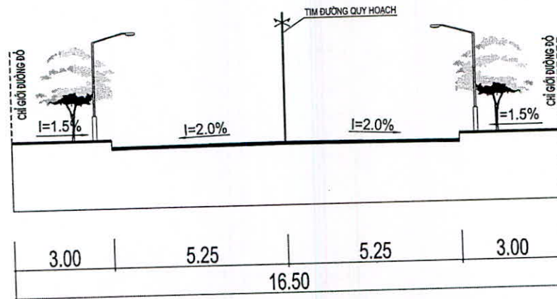
MẶT CẮT 1*1*-MẶT CẮT NGANG ĐIỂN HÌNH ĐƯỜNG CHÍNH ĐÔ THỊ ĐOẠN ĐI QUA ĐÔ THỊ
