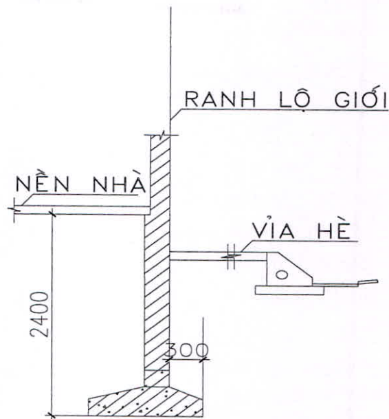
Hình 5 - Quy định về móng nhà giáp tường
