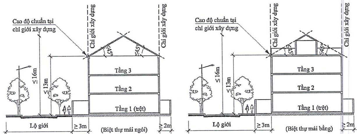
Hình 9. Minh họa tầng cao, chiều cao và mái biệt thự
