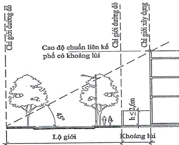
Hình 8. Minh họa cao độ chuẩn nhà liền kề phố có khoảng lùi
