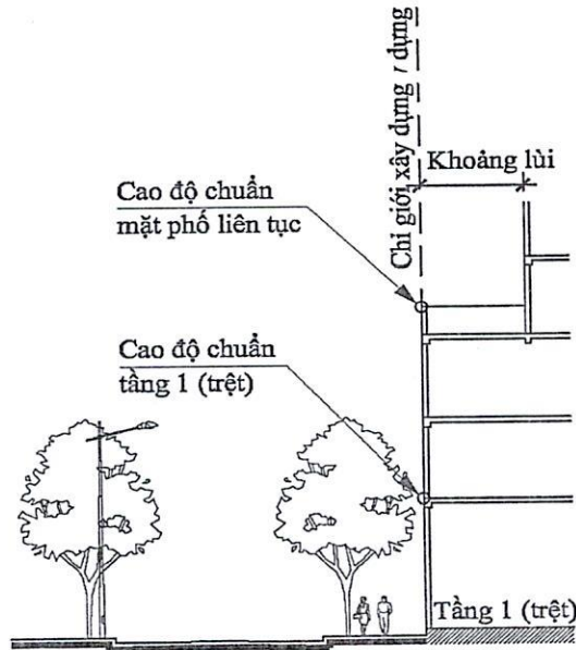
Hình 7. Minh họa chiều cao nhà mặt phố liên tục
