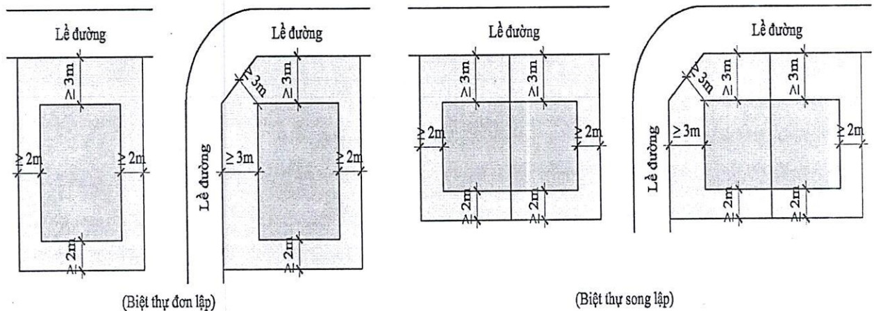
Hình 10. Chỉ giới xây dựng biệt thự
