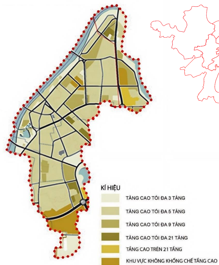
SƠ ĐỒ PHÂN BỐ TẦNG CAO XÂY DỰNG
