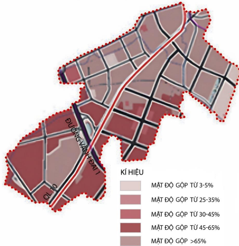
SƠ ĐỒ PHÂN BỐ MẬT ĐỘ XÂY DỰNG GỘP
