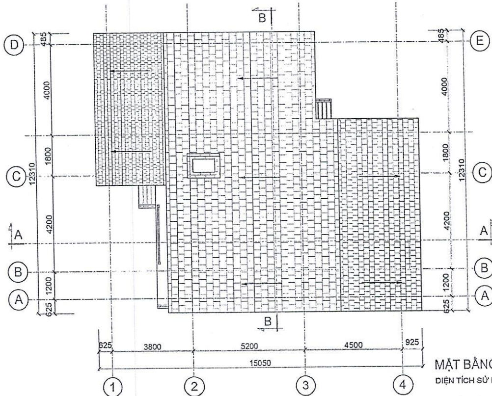
MẶT BẰNG DIỆN TÍCH SỬ DỤNG: 72m²
