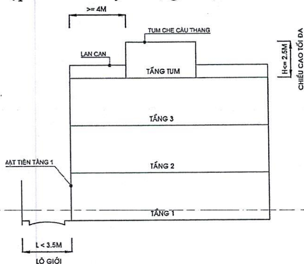
Hình 27: Quy định nhà ở trong ngõ nhỏ hơn 3,5m (trường hợp 4)
