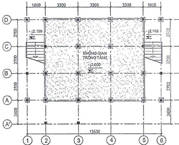
MẶT BẰNG TRỐNG TẦNG 1
