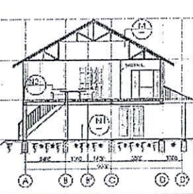
MẶT CẮT A-A
