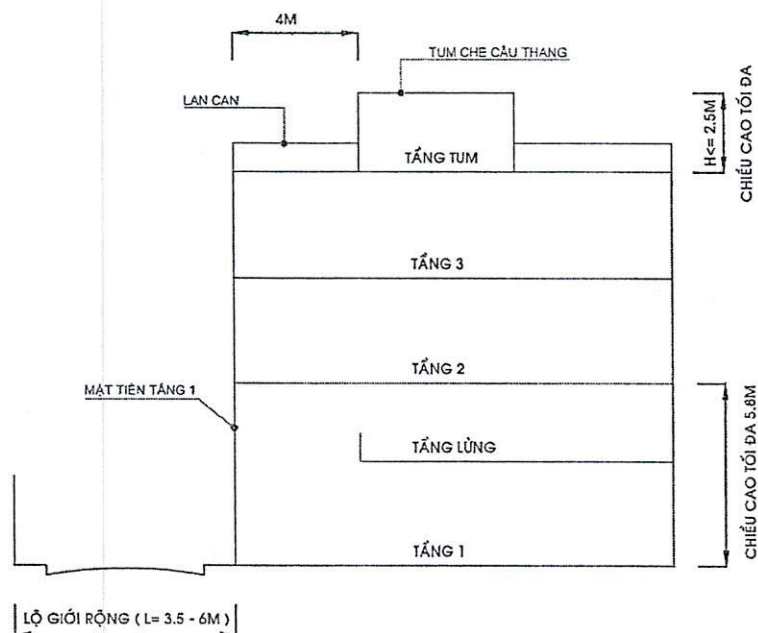
Hình 24: Quy định nhà ở trong ngõ 3,5 đến 6m (trường hợp 1)
