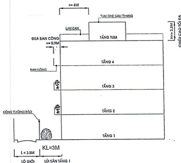
Hình 28: Quy định nhà ở trong ngõ nhỏ hơn 3,5m (trường hợp 5)
