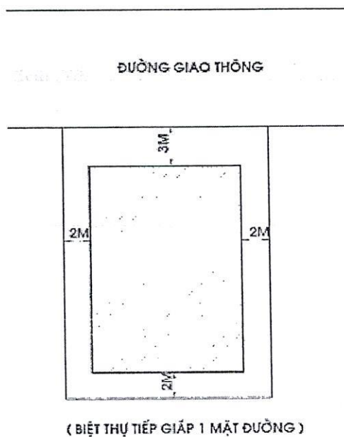
Hình 16: Minh họa quy định về khoảng lùi của biệt thự
