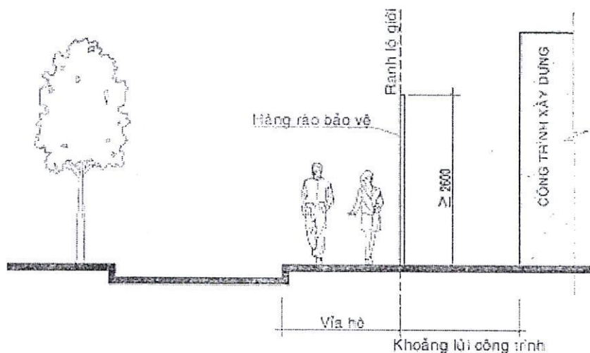
Hình 21: Hàng rào của công trình đang triển khai có khoảng lùi
