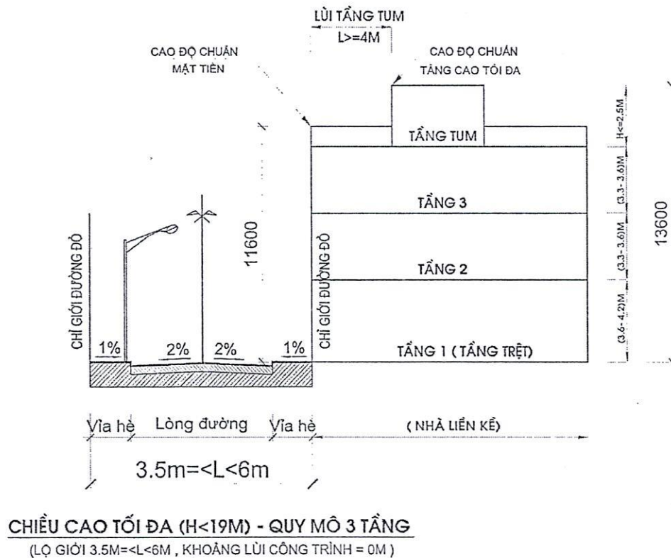
Hình 14: Minh họa khoảng tầng cao, khoảng lùi đối với lộ giới từ 3,5m đến 6m
