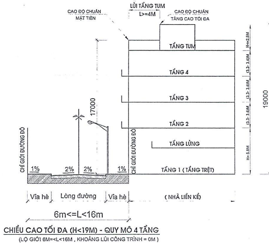
Hình 13: Minh họa khoảng tầng cao, khoảng lùi đối với lộ giới từ 6m đến 16m
