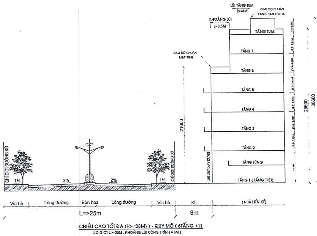
Hình 11: Minh họa khoảng tầng cao, khoảng lùi đối với lộ giới từ 25m trở lên
