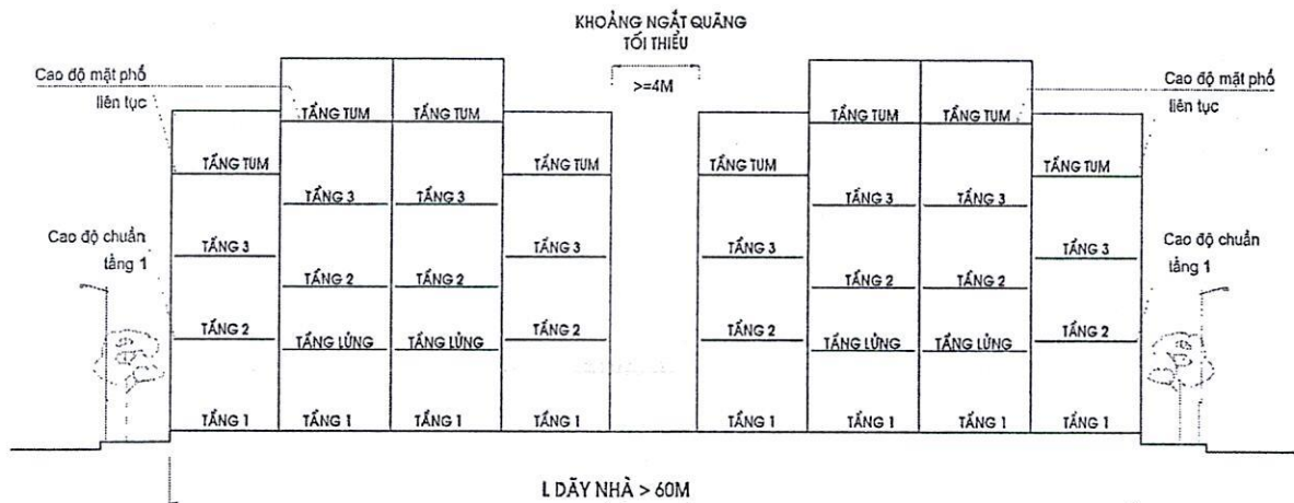
Hình 9: Quy định khoảng ngắt quãng tối thiểu với dãy nhà liên kế L > 60m
