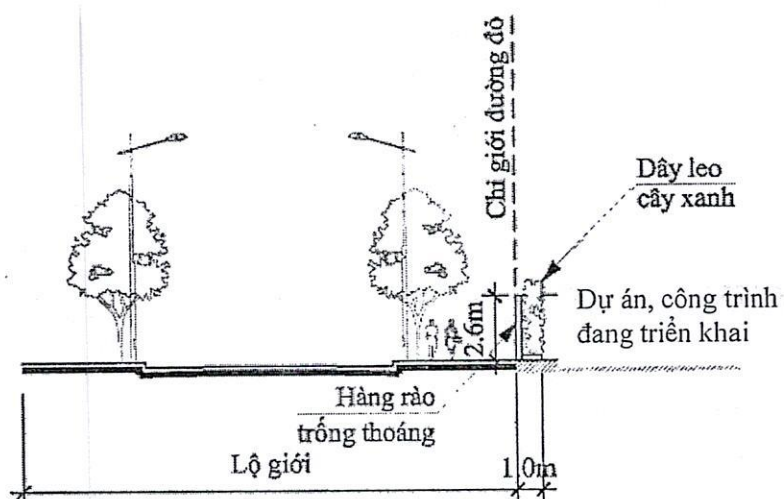
Hình 22: Hàng rào dự án, công trình đang triển khai sát chỉ giới đường đỏ
