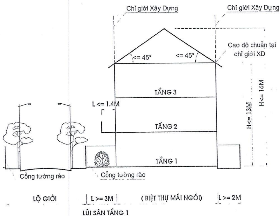
Hình 17: Minh họa quy định về số tầng nhà và chiều cao của biệt thự
