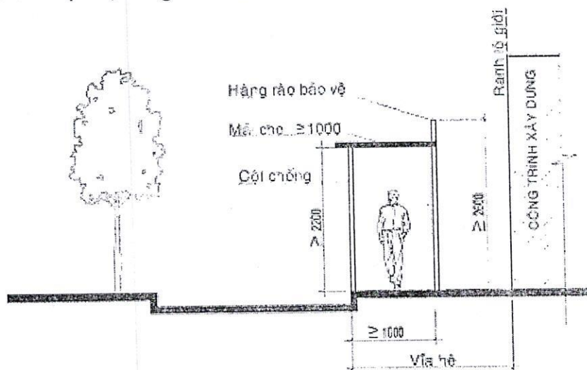
Hình 20: Hàng rào của dự án, công trình chưa triển khai sát ranh lộ giới
