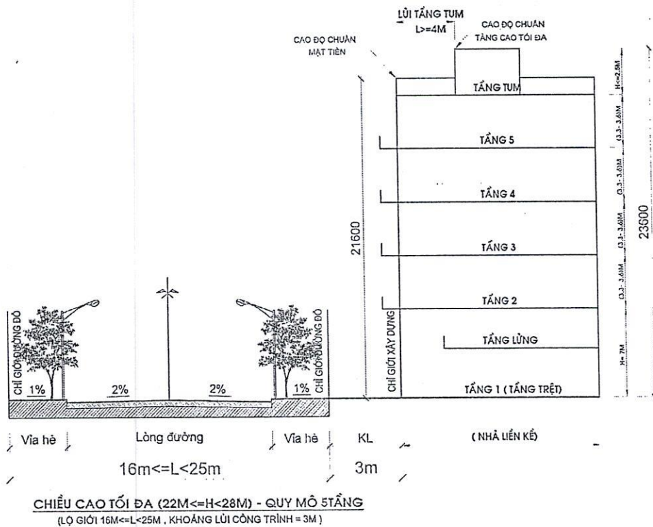
Hình 12: Minh họa khoảng tầng cao, khoảng lùi đối với lộ giới từ 16m đến dưới 25m
