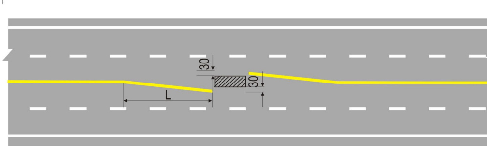
Hình G.70 - Vạch số 63: Đường 4 làn xe ở giữa có chướng ngại vật, đơn vị cm
