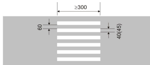
Hình G. 9 -Vạch số 9: Vạch đi bộ qua đường vuông góc, đơn vị cm
