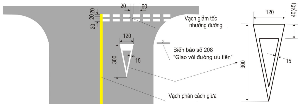
Hình G.48 - Vạch số 41: Vạch giảm tốc nhường đường, đơn vị cm
