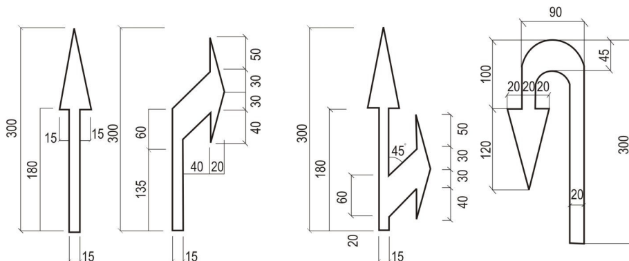
Hình G.31 - Vạch số 25 - Kích thước mũi tên chỉ đường áp dụng cho loại đường có tốc độ xe \leq 40\text{km/h} , đơn vị cm
