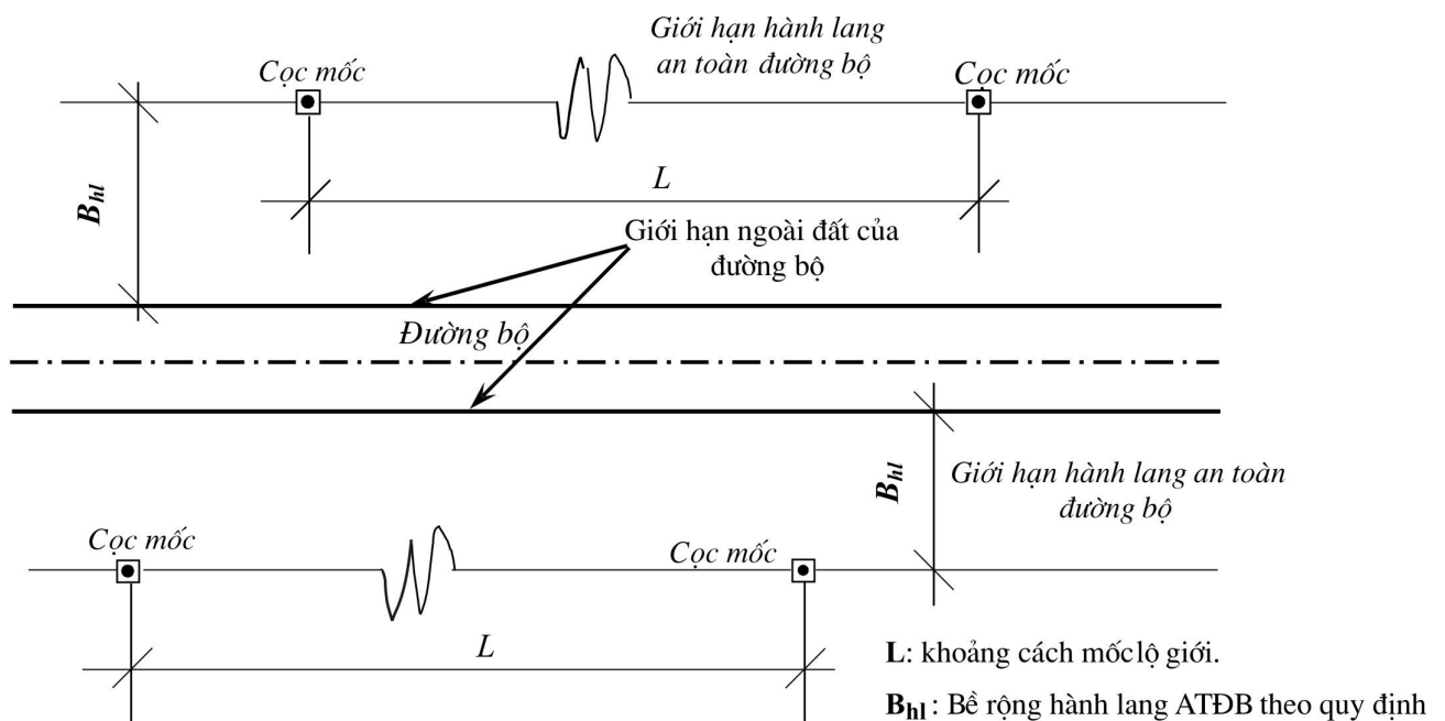
Hình I.4 - Mặt bằng bố trí mốc lộ giới
