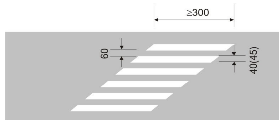
Hình G.10 - Vạch số 10: Vạch đi bộ qua đường cắt chéo, đơn vị cm
