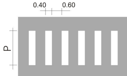
Hình H.14 - Vạch số 1.14, đơn vị m
