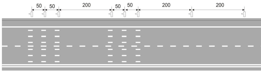
Hình G.13 - Vạch số 13: Vạch xác định khoảng cách xe, đơn vị m
