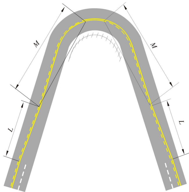
Hình G.36 - Vạch số 29: Bố trí vạch từ hai làn xe về một làn xe và ngược lại
