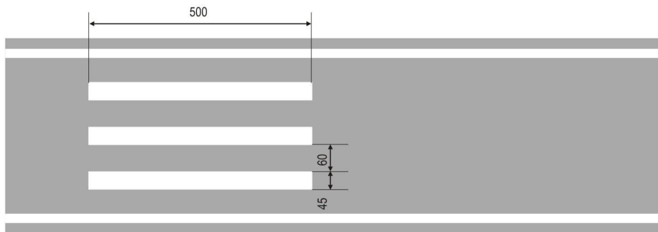
Hình G.14 - Vạch số 14: Kích thước vạch xác định khoảng cách xe, đơn vị cm
