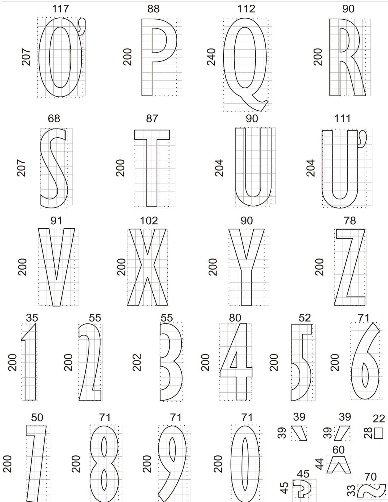
Hình K.4 - Chi tiết chữ viết và con số nét gầy, đơn vị mm
