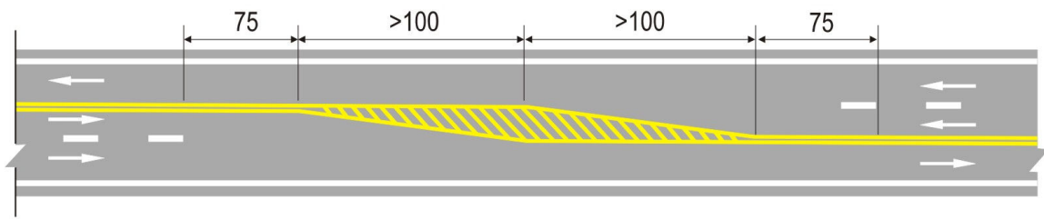
Hình G.67 - Vạch số 60: Đường 3 làn xe đoạn đảo làn xe giữa
