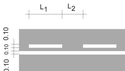
Hình H.11 - Vạch số 1.11, đơn vị m
