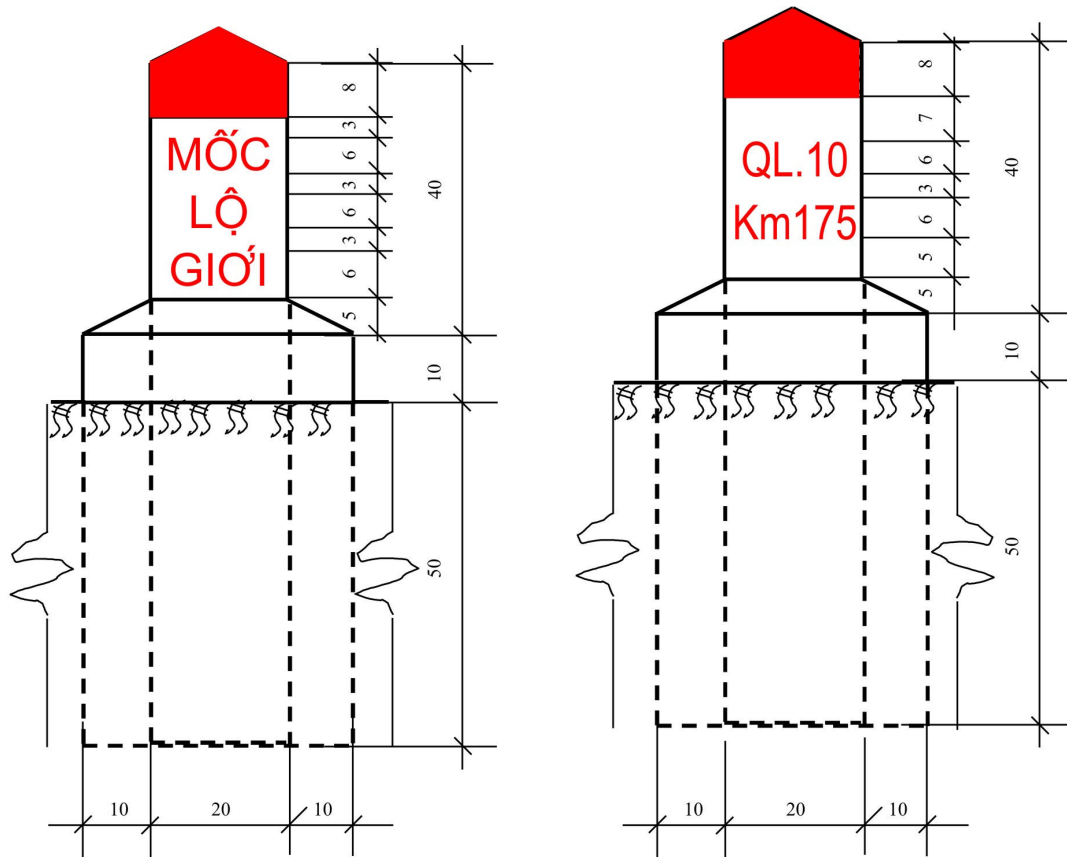
a) Mặt chính (nhìn ra phía đường) b) Hai mặt bên (hướng xe chạy)
