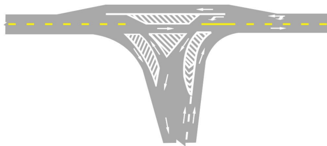
Hình G.51 - Vạch số 44: Vạch phân làn xe ở ngã ba đi lại phức tạp
