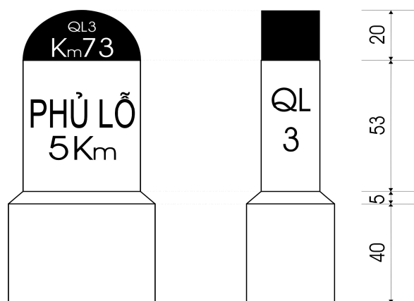
Hình I.1 - Cột Ki-lô-mét đặt ở lề đường, đơn vị cm
