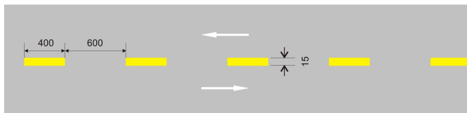
Hình G.1 - Vạch số 1: Đường tim trên mặt đường hai luồng xe ngược chiều, đơn vị cm
