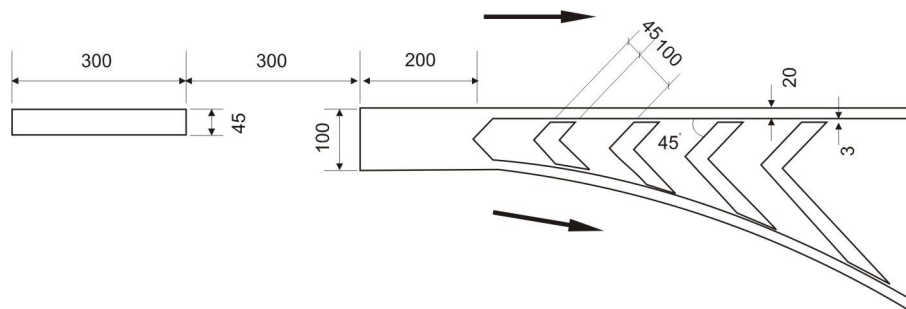
Hình G.15 - Bố trí tổng thể vạch tách làn, đơn vị cm
