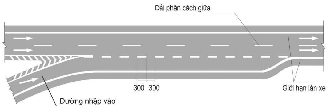
Hình G.19 - Vạch số 17: Vạch nhập làn kiểu trực tiếp, đơn vị cm
