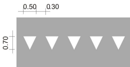
Hình H.13 - Vạch số 1.13, đơn vị m
