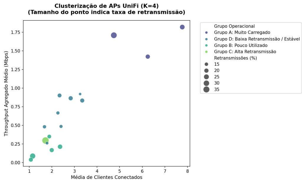
Figura 31 – Clusterização UniFi
