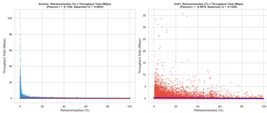
Figura 17 – Retransmissões x Throughput
