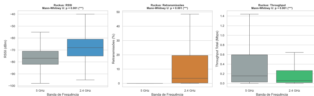
Figura 24 – Comparação de Bandas Ruckus
