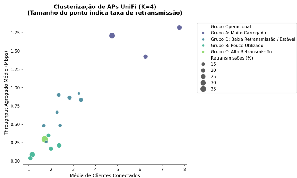
Figura 31 – Clusterização UniFi
