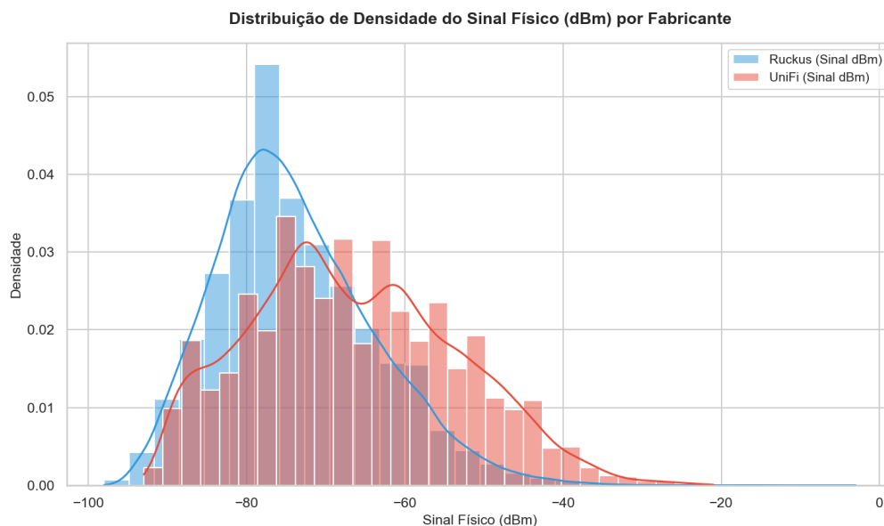
Figura 7 – Histograma RSSI
