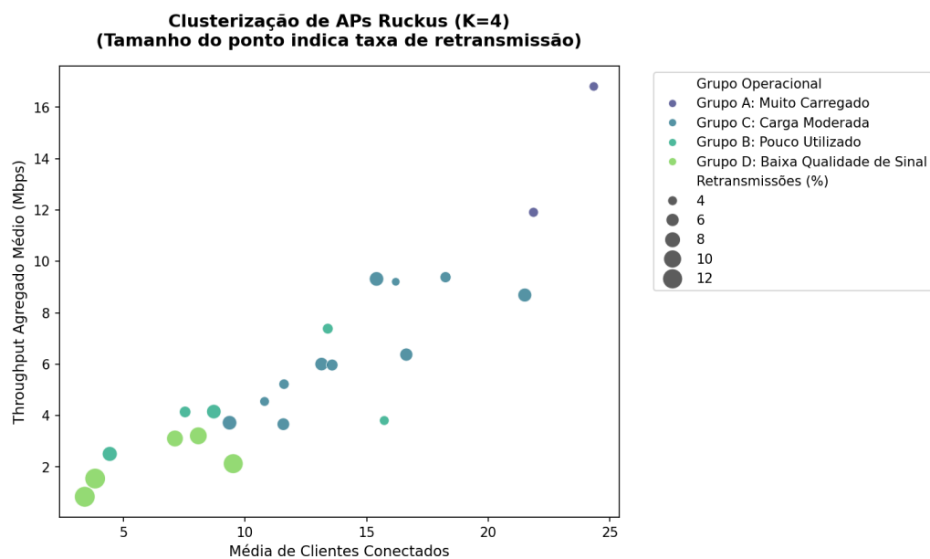
Figura 30 – Clusterização Ruckus
