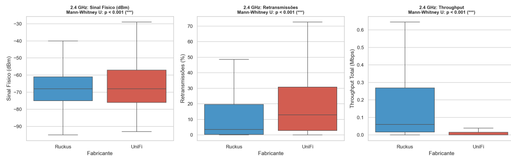
Figura 26 – Comparação de Fabricantes 2.4 GHz
