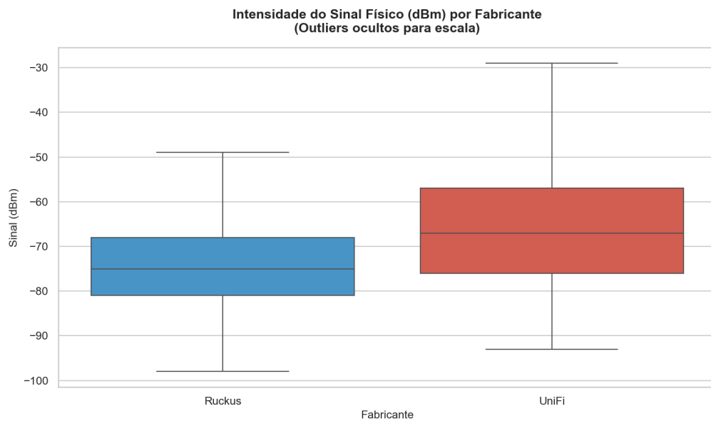
Figura 3 – Boxplot RSSI por Fabricante
