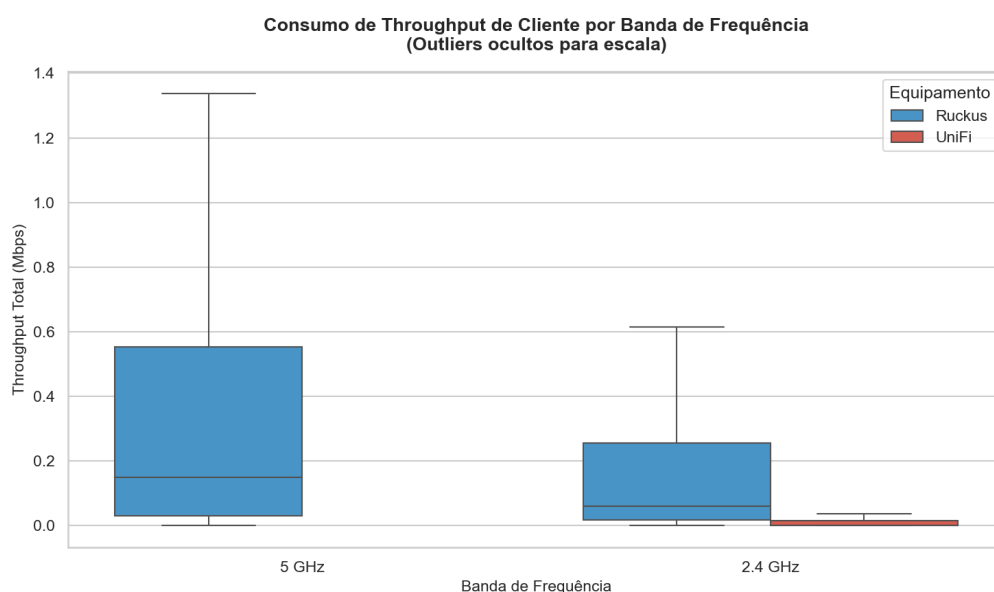
Figura 7 – Boxplot Throughput por Banda
