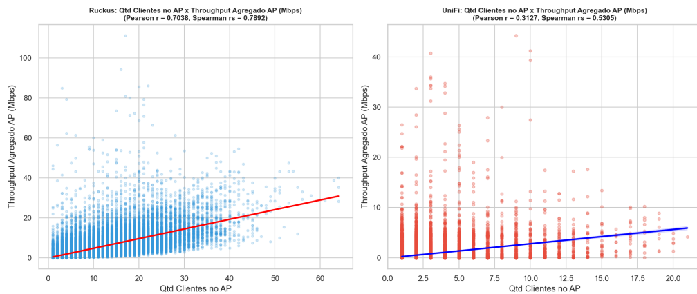
Figura 15 – Clientes x Throughput Agregado
