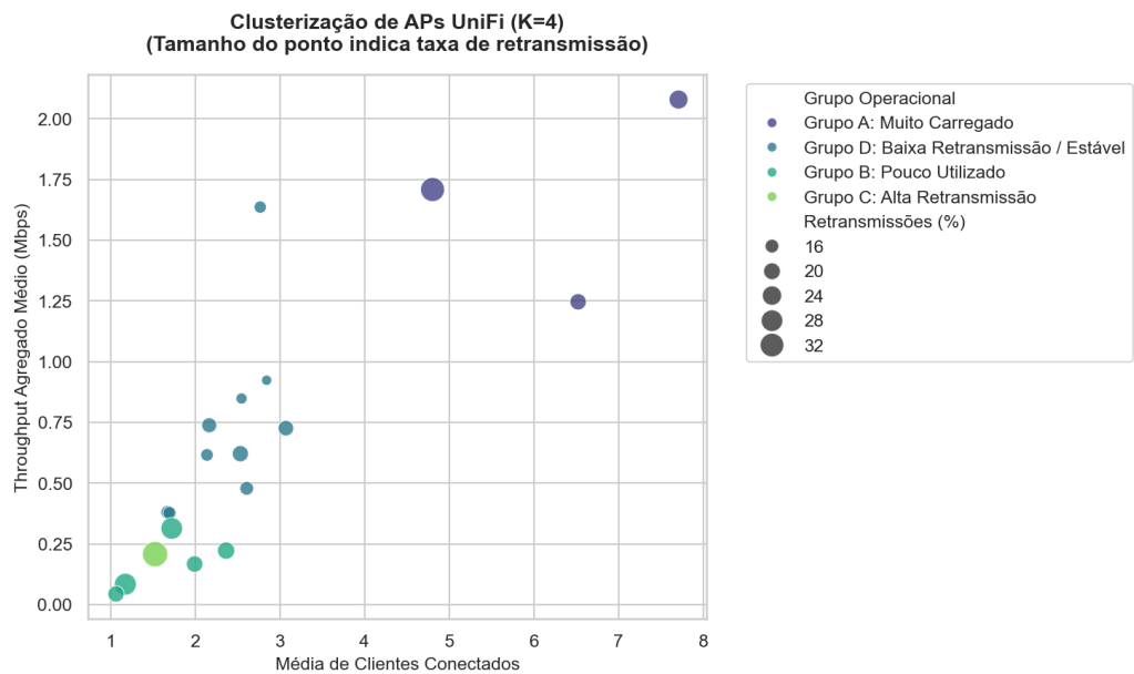
Figura 25 – Clusterização UniFi
