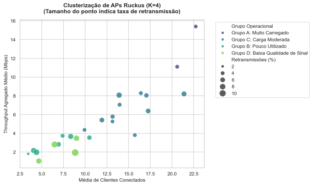
Figura 24 – Clusterização Ruckus
