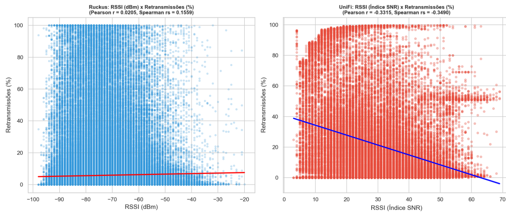
Figura 13 – RSSI x Retransmissões
