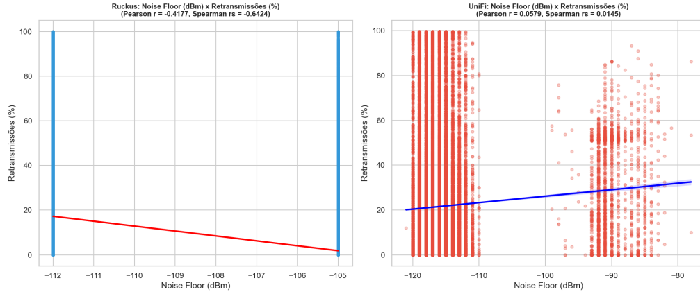
Figura 17 – Noise x Retransmissões
