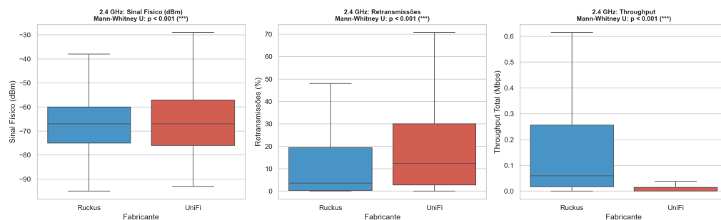
Figura 23 – Comparação de Fabricantes 2.4 GHz
