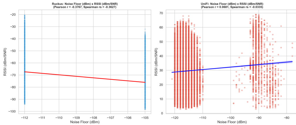
Figura 18 – Noise x RSSI
