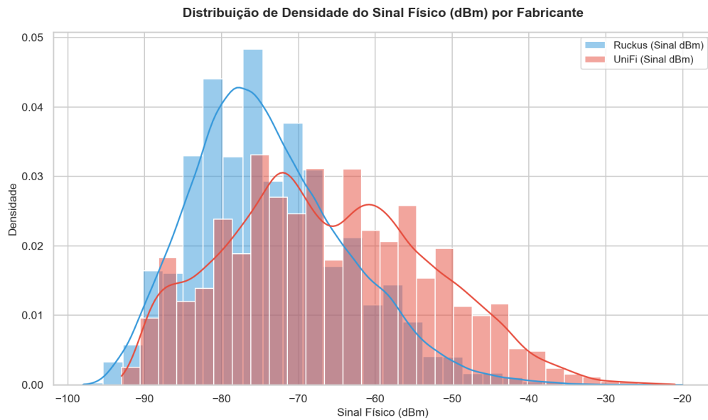
Figura 4 – Histograma RSSI
