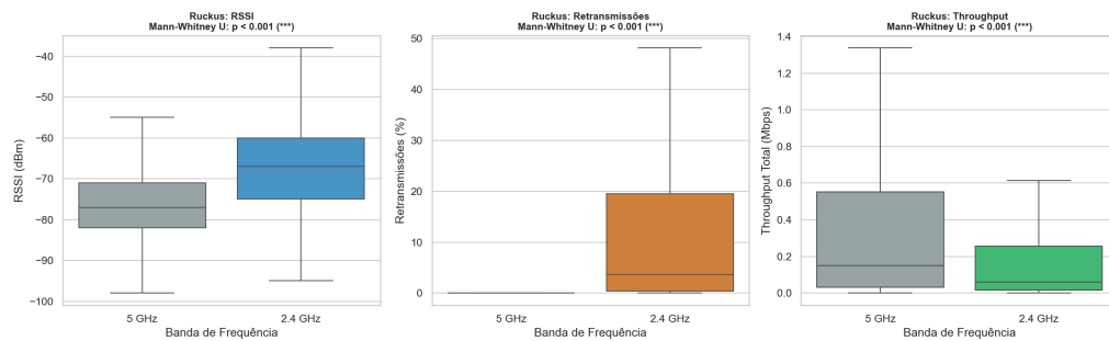
Figura 21 – Comparação de Bandas Ruckus
