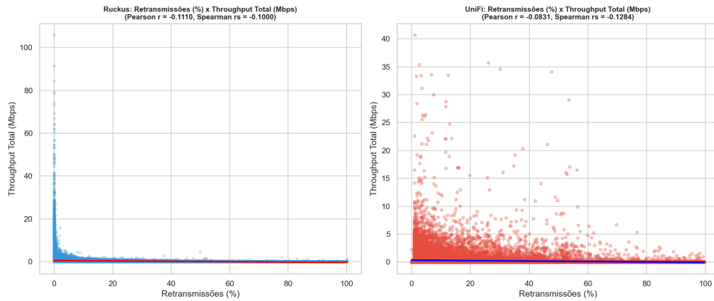
Figura 14 – Retransmissões x Throughput
