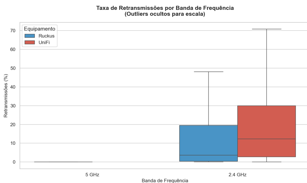
Figura 8 – Boxplot Retransmissões por Banda
