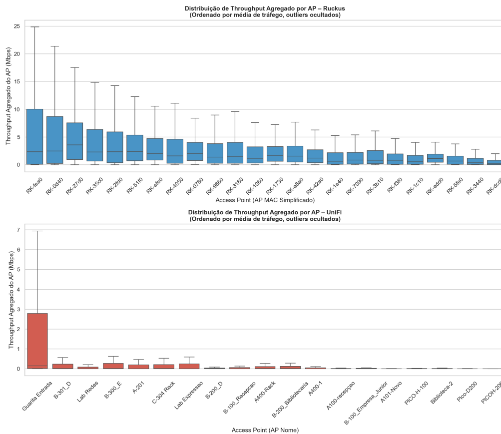
Figura 9 – Boxplot Throughput por AP
