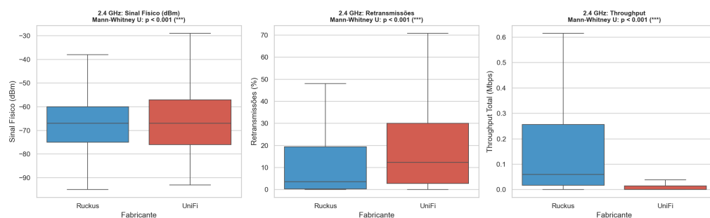
Figura 23 – Comparação de Fabricantes 2.4 GHz
