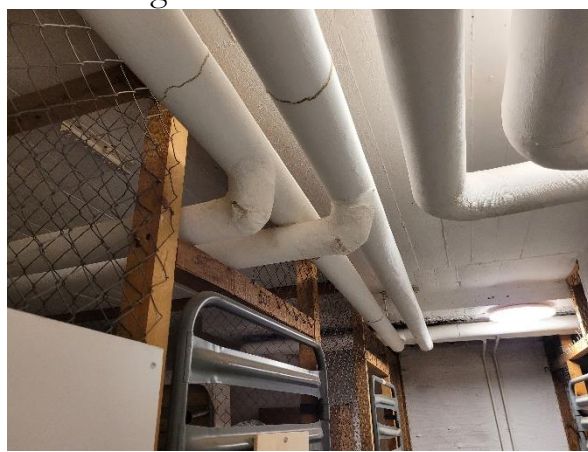
Bild 20: Rör med antagen asbestisolering i böjar, ändrar och t-rör (Foto: Dirigentgatan 3)
