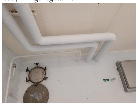
Bild 14: Rörböjar med antagen asbest. (Foto: Dirigentgatan 1)
