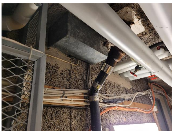
Bild 21: Synlig plåtkanal tätningsmassa som innehåller asbest (Prov P9). (Foto: Dirigentgatan 4)
