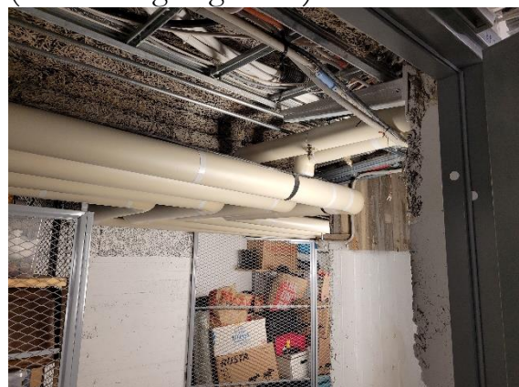
Bild 16: Rör bedömt utan asbest. Plastisol-inklädd rörisolering som är klädd med papp. (Foto: Dirigentgatan 1)
