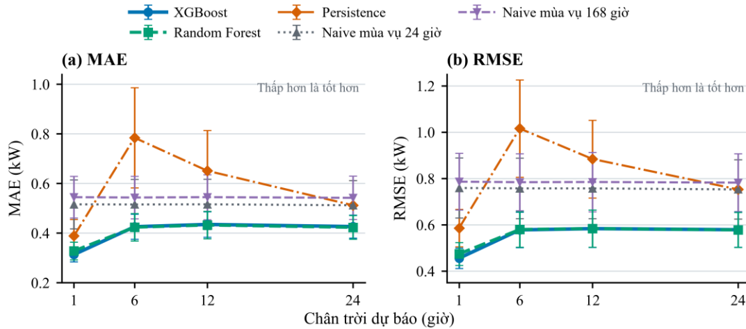
Hình 4. Sai số MAE và RMSE tại các chân trời h+1, h+6, h+12 và h+24; error bar biểu diễn sample SD
