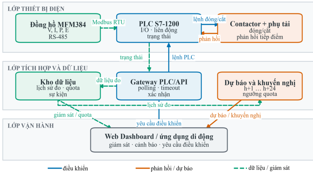
Hình 1. Kiến trúc dự kiến của chuỗi đo–điều khiển và quản lý phụ tải; các kết luận phần cứng phải được xác nhận bằng log thử nghiệm
