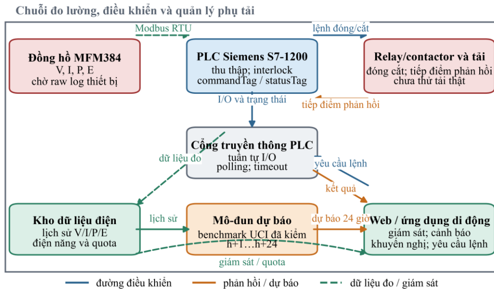
Hình 1. Kiến trúc dự kiến của chuỗi đo–điều khiển và quản lý phụ tải; các kết luận phản cứng phải được xác nhận bằng log thử nghiệm
