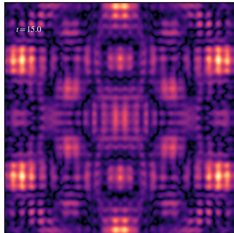
(d) numerical_fragmentation ( k_0=1.8 )
