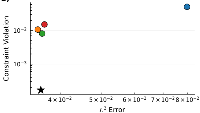
(d) Kuramoto-Sivashinsky
