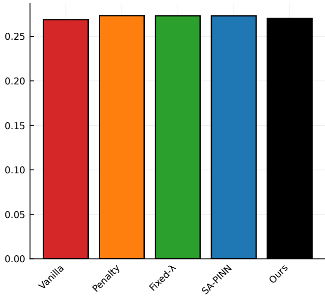
GPU Mem
