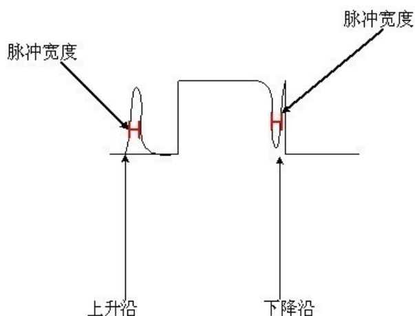
图 3-19 触发波形
