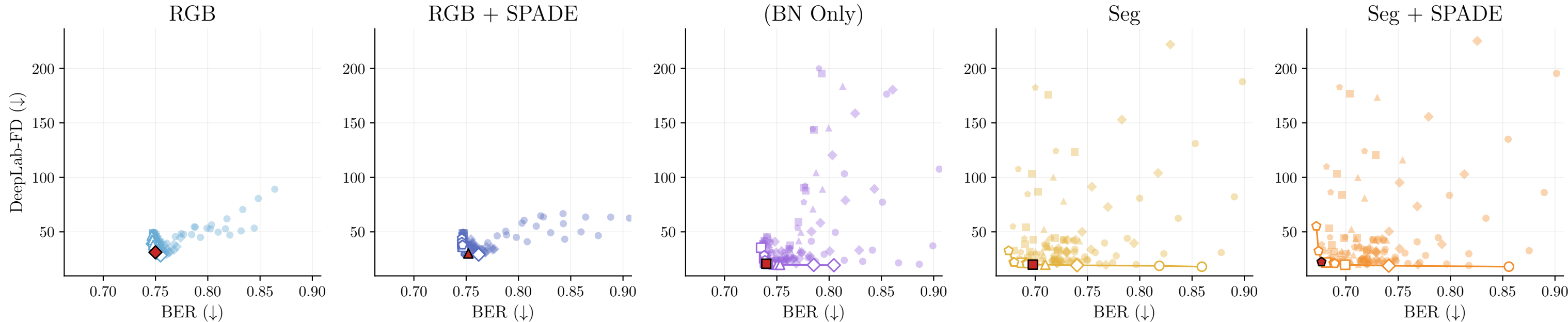
Pareto Tradeoff
