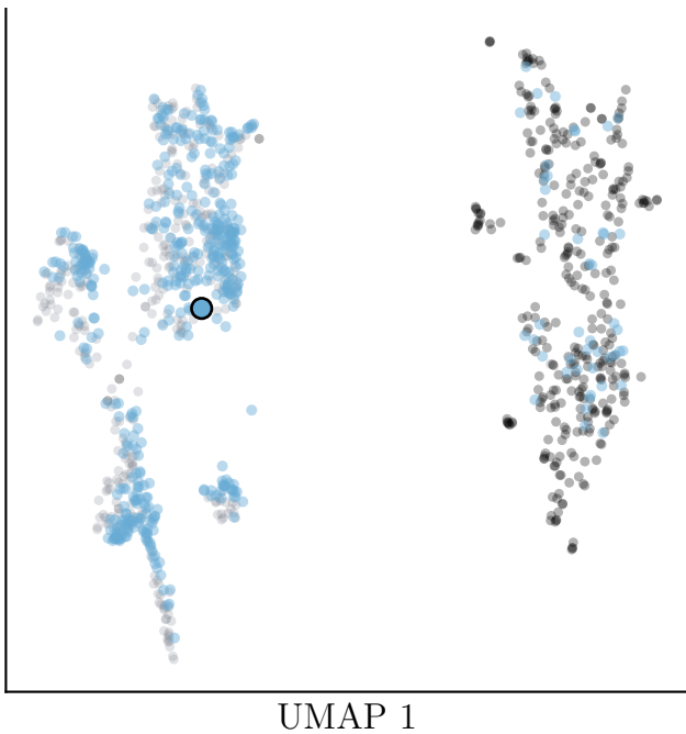
RGB
