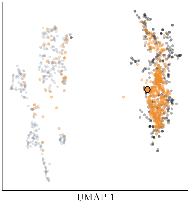
Seg + SPADE
