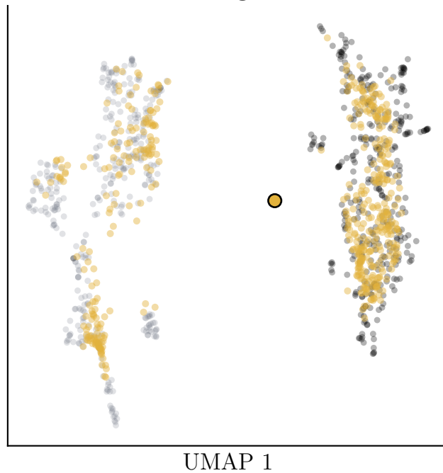
Seg
