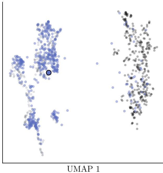
RGB + SPADE
