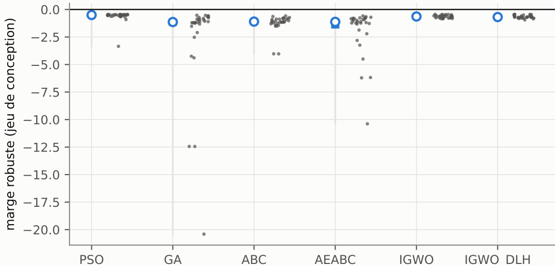
Distribution par graine — bras v5 (unite = graine)
