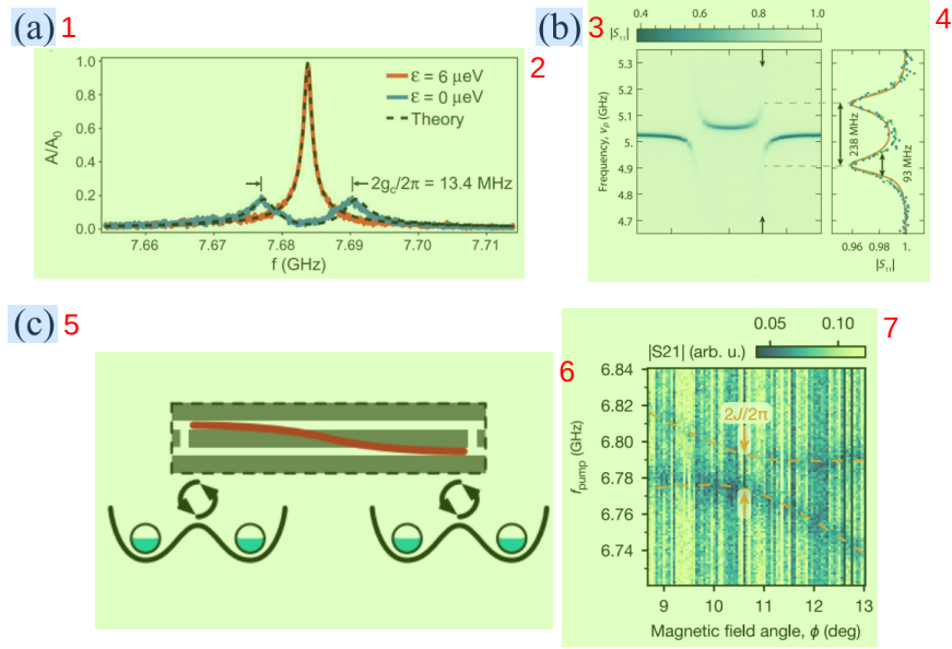
图 1.8 (a) Petta 组观察到的真空拉比劈裂 [32] 。(b) 利用 SQUID 阵列腔, wallraf 组实现了更大的劈裂 [33] 。(c) Vandersypen 组实现的两个自旋比特利用虚光子实现的长程相干耦合 [34] 。在这组图里我们只展示了几个重要的结果, 其他实验中观察到的现象与这些结果类似, 就没有重复展示。在后面的小节中, 我们也遵循同样的原则。
