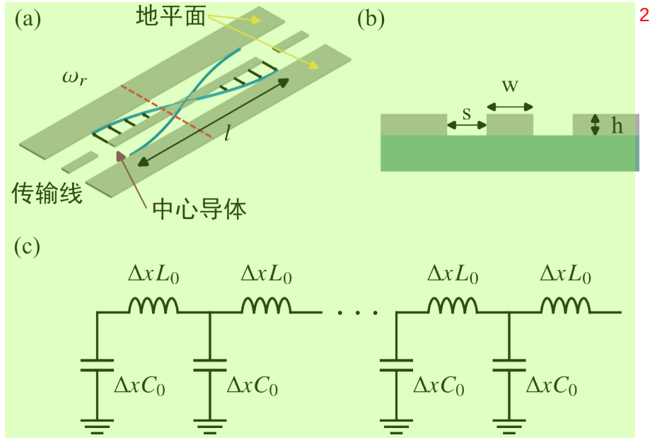
图 1.6 (a) 半波长 ( \lambda/2 ) 共面波导透射腔的示意图，包括中心导体、两个传输线以及两个地平面。其中灰色部分为金属。如果将其中一个传输线接地，那么就可以形成四分之一波长 ( \lambda/4 ) 的反射腔。(b) 腔的横截面（沿 (a) 中红色虚线）示意图。 w 为中心导体的宽度， s 为中心导体和地平面之间的间隔， h 为金属的厚度。绿色部分为衬底，在我们的样品中为砷化镓。(c) 腔的等效电路图。
