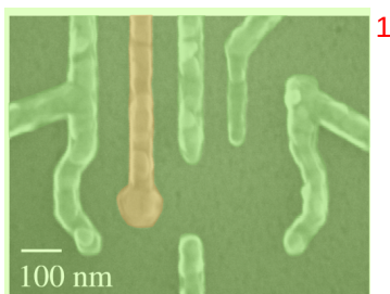
图 1.2 门控量子点电极结构图，图中绿色、粉色结构为微纳加工形成的金属栅极。 2
