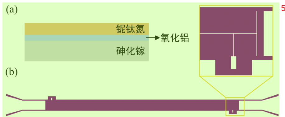
图 14 (a) 垂直衬底方向的结构示意图。(b) 铌钛氮透射腔的设计图。放大的地方为腔与量子点以及传输线耦合的部分。
