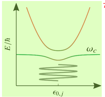
图 5.3 一个双量子点-腔耦合系统的能级示意图。绿色代表腔光子态,而红色代表双量子点的态,线的颜色代表了耦合相互作用导致的两个态的杂化程度。灰色的振荡曲线代表微波驱动。裸腔由一个谐振子哈密顿量描述,其能级是无穷维的,间隔为 \omega_r ,当然鉴于腔中的较低的光子数占据数目,一般只需要考虑最低的 N 个能级。这导致耦合后的系统态空间的维度为 2 \times N 维。图中展示的是激发数为 1 的两个态。对于本章涉及的实验参数,其他能级的能量较高,可以忽略 [17] 。
