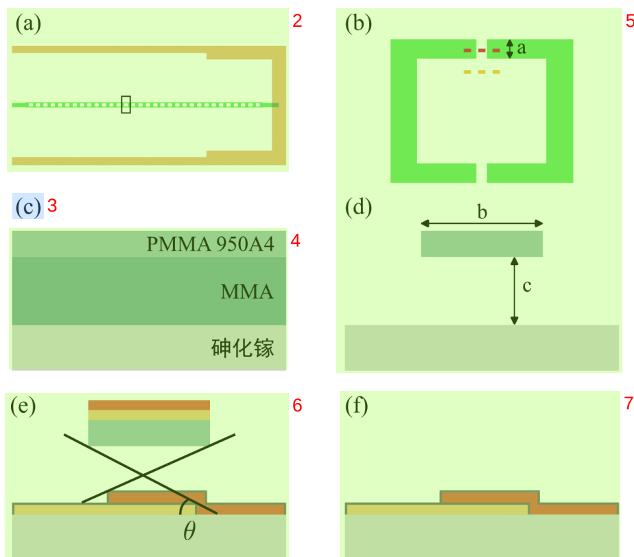
图 13 (a) SQUID 阵列反射腔设计图，图中绿色的部分即为 SQUID 阵列。(b) 图 (a) 中黑色方框部分的放大细节图。这是一个 SQUID 的设计图，红色虚线所在位置即形成约瑟夫森结的地方。绿色部分为被曝光的区域。(c) 甩完双层胶后的与衬底垂直方向的截面示意图。灰色部分即为衬底。上面两层为电子束胶。(d) 曝光显影后，红色虚线所在位置处的纵向截面示意图。(e) 双层蒸镀工艺示意图。图中黄色部分为第一层蒸镀的铝金属，而深灰色部分表示氧化后的氧化铝，橘红色部分为第二层蒸镀的铝金属。(f) 剥离后剩下的 SQUID 双层金属结构。
