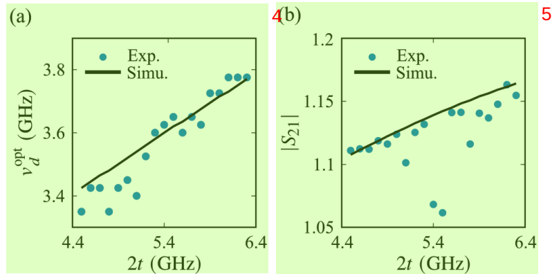
图 4.6 (a) 最佳驱动频率 v_d^{\text{opt}} 和 (b) 最大腔增益随 2t 的变化。图中的点提取自实验数据。而黑色实线 (Simu.) 为理论计算的结果，类似于图4.4，这里的理论数据也是提取自计算的 LZSM 干涉图。
