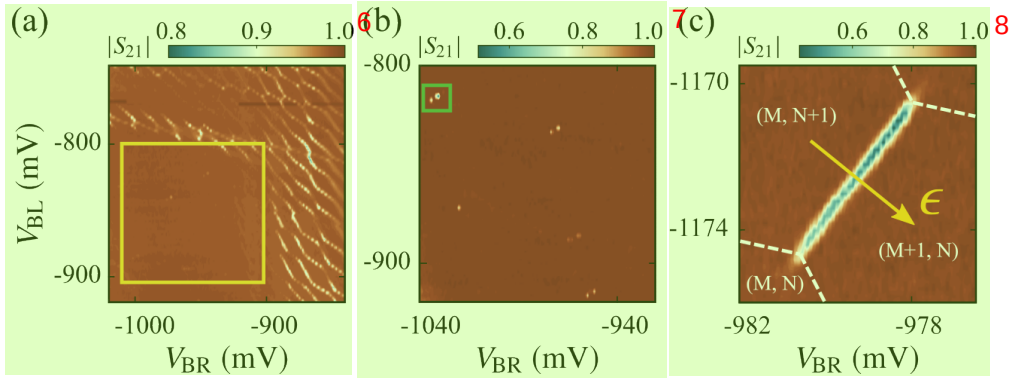
图 2.10 (a) 测得透射腔的透射幅值 |S_{21}| 、(b) 细扫的 |S_{21}| 、(c) 在量子点共振隧穿线附近的 |S_{21}| 随量子点电极电压变化的相图。图 (c) 中黄色箭头指示了量子点失谐 \epsilon 变化的方向。在测量这组数据时，我们把探测频率固定在腔频处，即 \omega = \omega_r 。
