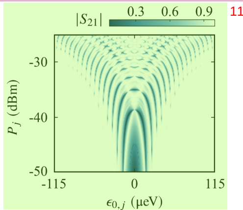
图 5.4 利用受驱动的双量子点和腔耦合系统的响应理论计算得到的 |S_{21}| 。具体计算的参数和图 5.2 (b) 相同。 12
