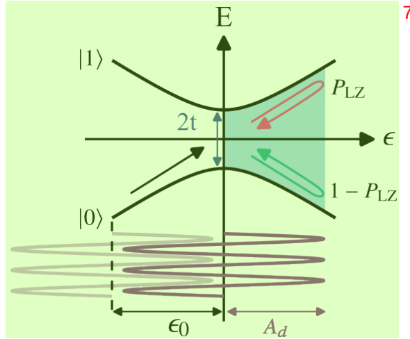
图 2.12 受驱动的二能级示意图。图中紫色的实线、散射的箭头以及积累的相位（蓝色区域）为 \epsilon_0 = 0 的情形。
