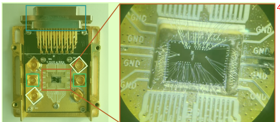
图 15 样品封装到样品盒后的实物图。放大部分更加清楚地展示了键合线将样品对应电极和印制电路板上对应区域连接。
