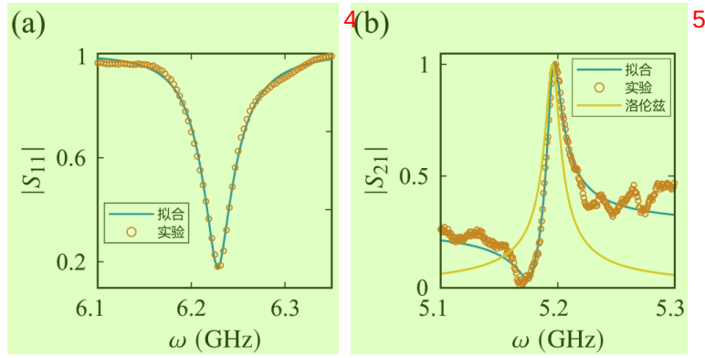
图 2.9 (a) 反射腔的反射信号幅值 |S_{11}| 、(b) 透射腔的透射信号幅值 |S_{21}| 随探测频率 \omega 的变化。圆圈为测得的实验数据，蓝色实线为公式拟合的曲线。没有法诺效应时，腔的线性为洛伦兹线形，即图中黄色实线。
