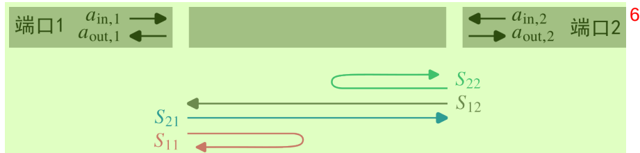
图 2.4 腔的二端口结构以及散射参数定义示意图。 7
