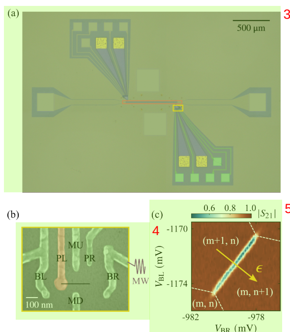
图 4.1 (a) 着色的器件光学显微镜图。这个器件由一个超导的铌钛氮透射腔和两个砷化镓双量子点组成。(b) 着色的双量子点的扫描电子显微镜图。电极 BL、PL、MU、PR、BR 和 MD 用来控制双量子点的势阱。Plunger 电极 PL（粉色）连接到腔的中心导体上。(c) 测量得到腔的归一化的透射信号 |S_{21}| 随电极电压 V_{BR} 和 V_{BL} 的变化，这其实就是双量子点的电荷稳态图。图中黄色的箭头代表了失谐 \epsilon 的方向。 3
