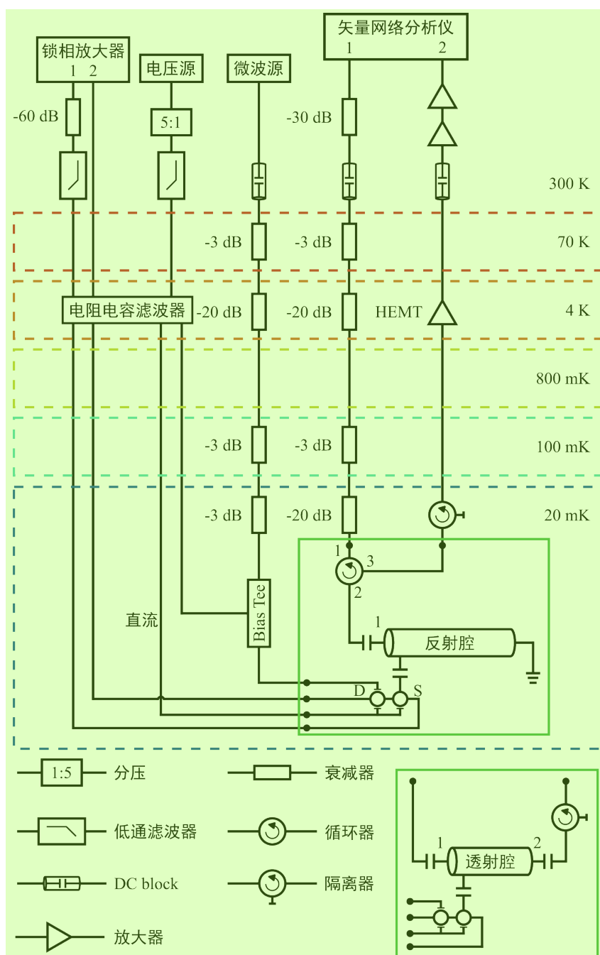
图 2.7 样品的测量线路示意图。不同颜色的虚线框代表稀释制冷机中不同的温度层。绿色实线框中为样品示意图。上面绿色方框中的为反射腔-量子点耦合的样品示意图。S 和 D 代表量子点的源漏，一个圆圈代表一个量子点。用下面绿色方框中的线路替换掉上面绿色方框中的线路，就可以得到透射腔-量子点耦样品测量线路。
