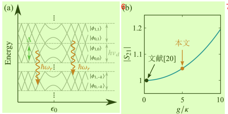
图 4.3 (a) Floquet 态的准能级结构示意图，其周期为 \hbar v_d 。红色的箭头代表两个准能级的能级差和腔频匹配时，受驱动的双量子点会向腔中发射一个光子。(b) 利用理论计算得到的在 G1 处的 |S_{21}| 随 g/\kappa 的变化曲线。图中黑色的点为文献 [20] 中的参数计算得到的增益值，而红色的点为我们的样品参数计算得到的增益值。
