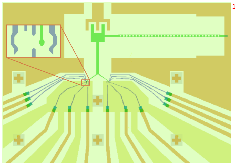
图 2.5 SQUID 阵列反射腔和量子点耦合样品设计图。图中绿色部分为 SQUID 阵列，构成了腔的中心导体，橘色部分为腔的地平面。紫色的小电极是两个双量子点，插图部分为放大的双量子点的电极结构，两个量子点的结构相同，成镜像对称。腔中心导体部分伸出一根金属导体连接到两个双量子点的 plunger 电极（绿色）上，实现腔和量子点的耦合。
