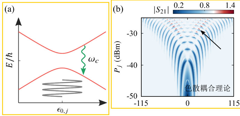
图 5.2 (a) 双量子点的能级示意图。灰色的振荡曲线代表微波驱动。(b) 利用色散耦合理论计算得到的 |S_{21}| 。具体计算的参数为 \omega_p = \omega , 2t_j/h = 5.2 GHz, g_j/2\pi = 85 MHz, f_d = 1.4 GHz。图中驱动功率 P_j = -40 dBm 对应于幅值 A_{d,j} = 20.2 \mu eV。
