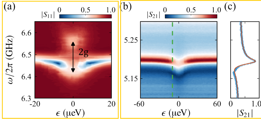
图 2.11 (a-b) 不同样品上测量得到的腔信号随 \epsilon 和探测频率 \omega 变化的相图。此时量子点的转变频率 \omega_q 与腔频 \omega_c 相等。当量子点和腔的耦合强度大于比特和腔的耗散速率时，可以看到真空拉比劈裂。(c) 在 \epsilon = -8 \mu\text{eV} 处（图 (b) 绿色虚线）， |S_{21}| 随 \omega_p 的变化。我们可以看到线型并不对称，这是前面讨论的法诺效应导致的 [30] 。
