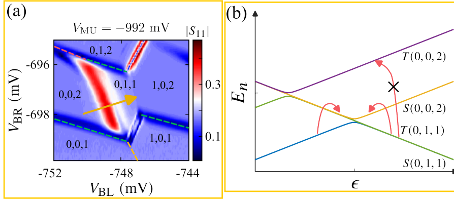
图 3.6 (a) 放大的电荷稳态图，展示了点 2 和点 3 之间隧穿线的细节。(b) 三量子点的本征能量随 \epsilon 变化的示意图。由于没有外加磁场，因此这里相同电荷态的自旋三态是简并的。图中的 |T(0, 1, 1)\rangle 是三重简并的，代表了 |T_0(0, 1, 1)\rangle ， |T_+(0, 1, 1)\rangle 和 |T_-(0, 1, 1)\rangle 。图中的 |T(0, 0, 2)\rangle 代表了 |T_0(0, 0, 2)\rangle ， |T_+(0, 0, 2)\rangle 和 |T_-(0, 0, 2)\rangle 。
