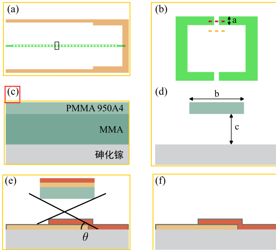
图 13 (a) SQUID 阵列反射腔设计图，图中绿色的部分即为 SQUID 阵列。(b) 图 (a) 中黑色方框部分的放大细节图。这是一个 SQUID 的设计图，红色虚线所在位置即形成约瑟夫森结的地方。绿色部分为被曝光的区域。(c) 用完双层胶后的与衬底垂直方向的截面示意图。灰色部分即为衬底。上面两层为电子束胶。(d) 曝光显影后，红色虚线所在位置处的纵向截面示意图。(e) 双层蒸镀工艺示意图。图中黄色部分为第一层蒸镀的铝金属，而深灰色部分表示氧化后的氧化铝，橘红色部分为第二层蒸镀的铝金属。(f) 剥离后剩下的 SQUID 双层金属结构。
