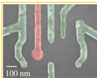
图 1.2 门控量子点电极结构图，图中绿色、粉色结构为微纳加工形成的金属栅极。
