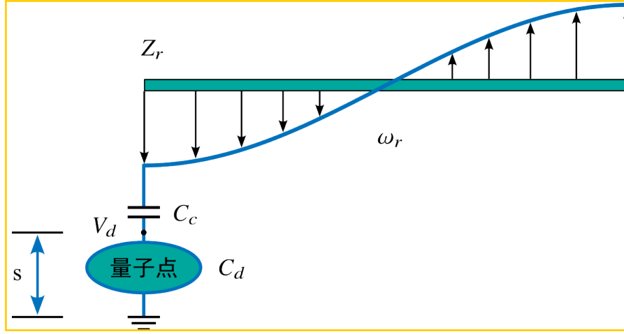
图 1.7 量子点和腔耦合示意图。由于我们这里利用的是电偶极相互作用，一般将量子点制备在腔的电压波腹处从而尽可能大地增强量子点和腔之间的耦合强度。
