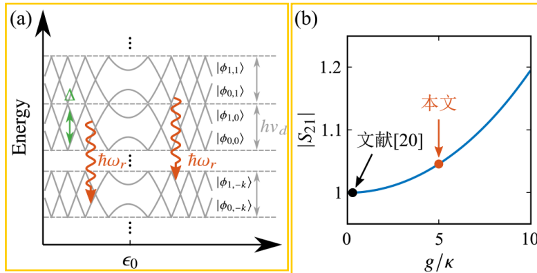
图 4.3 (a) Floquet 态的准能级结构示意图，其周期为 hv_d 。红色的箭头代表两个准能级的能级差和腔频匹配时，受驱动的双量子点会向腔中发射一个光子。(b) 利用理论计算得到的在 G1 处的 |S_{21}| 随 g/\kappa 的变化曲线。图中黑色的点为文献 [20] 中的参数计算得到的增益值，而红色的点为我们的样品参数计算得到的增益值。
