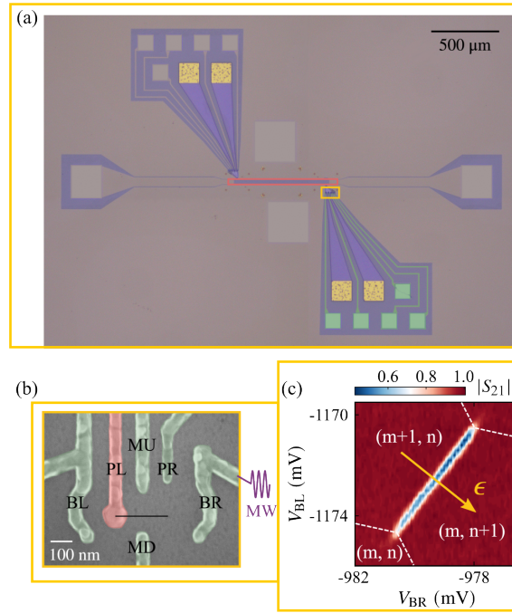
图 4.1 (a) 着色的器件光学显微镜图。这个器件由一个超导的铌钛氮透射腔和两个砷化镓双量子点组成。(b) 着色的双量子点的扫描电子显微镜图。电极 BL、PL、MU、PR、BR 和 MD 用来控制双量子点的势阱。Plunger 电极 PL (粉色) 连接到腔的中心导体上。(c) 测量得到腔的归一化的透射信号 |S_{21}| 随电极电压 V_{BR} 和 V_{BL} 的变化，这其实就是双量子点的电荷稳态图。图中黄色的箭头代表了失谐 \epsilon 的方向。
