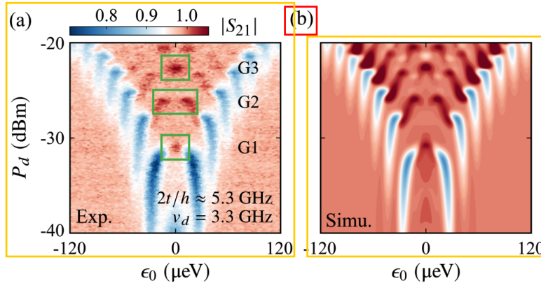
图 4.2 (a) 测量 |S_{21}| 得到的 LZSM 干涉图，驱动频率 \nu_d = 3.3 GHz， 2t/h \approx 5.3 GHz。图中绿色方框指示的区域，按施加驱动功率的大小，从小到大分别定义为 G1、G2、G3。图中最大的幅值增益约为 1.07。(b) 利用理论计算得到的模拟图。这里驱动功率 P_d = -40 dBm 对应于驱动幅值 A_d = 11.4 \mu eV。由于我们的样品上存在准静态的电荷噪声 (quasistatic charge noise) 以及施加的微波幅值存在抖动，这会导致信号非均匀的展宽。为了模拟这种展宽导致的信号的平滑，我们对计算得到的数据在 \epsilon 和 P_d 轴方向上都做了高斯卷积 [12,24-25] ，使得模拟结果更加符合实际情况。我们使用的高斯分布的标准差为 \sigma_\epsilon = 3.3 \mu eV， \sigma_{P_d} = 0.2 dBm。
