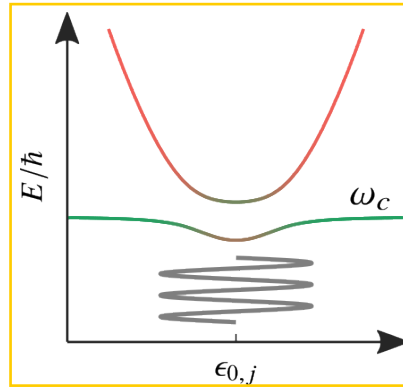
图 5.3 一个双量子点-腔耦合系统的能级示意图。绿色代表腔光子态,而红色代表双量子点的态,线的颜色代表了耦合相互作用导致的两个态的杂化程度。灰色的振荡曲线代表微波驱动。裸腔由一个谐振子哈密顿量描述,其能级是无穷维的,间隔为 \omega ,当然鉴于腔中的较低的光子数占据数目,一般只需要考虑最低的 N 个能级。这导致耦合后的系统态空间的维度为 2 \times N 维。图中展示的是激发数为1的两个态。对于本章涉及的实验参数,其他能级的能量较高,可以忽略 [17] 。
