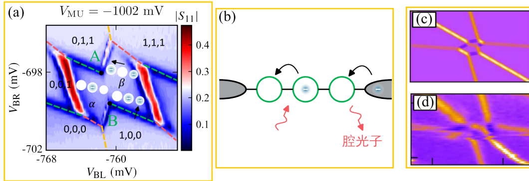
图 3.4 (a) 放大的电荷稳态图。图中黑色的箭头代表了电子的跃迁方向。(b) 量子元胞自动机现象中的跃迁过程的示意图, 图中黑色箭头代表电子的跃迁, 粉色的箭头代表了腔光子的吸收和发射。(c) 模拟的 OPC 测量的电荷稳态图, 图自文献 [10] 。(d) Ludwig 组用 QPC 测得的电荷稳态图 [10] 。
