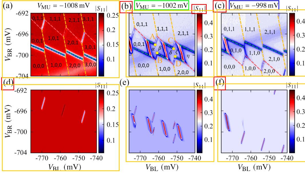
图 3.3 三量子点在不同的 V_{MU} 电压下的电荷稳态图。(a) V_{MU} = -1008 \text{ mV} ，(b) V_{MU} = -1002 \text{ mV} ，其中希腊字母 \alpha, \beta, \delta, \zeta, \eta 分别代表态 (0, 1, 0) ， (1, 0, 1) ， (1, 1, 0) ， (2, 0, 1) 和 (2, 1, 0) 。(c) V_{MU} = -998 \text{ mV} 。为了区别不同的电荷态区域，我们在图中添加了一系列黄色、粉色、绿色的线，这对应于量子点 1、2、3 的充电线。(d-f) 由公式(3.10)计算得到的电荷稳态图。计算时采用的具体参数：(d) (t_{12}, t_{13}, t_{23}) = (9.9, 0, 11.9) \mu\text{eV} ，在中间的隧穿线处 ( V_{BL} = -760 \text{ mV} 附近)， t_{12} = 3.2 \mu\text{eV} ，(e) (t_{12}, t_{13}, t_{23}) = (13.5, 0, 13.1) \mu\text{eV} ，(f) (t_{12}, t_{13}, t_{23}) = (13.3, 0, 13.1) \mu\text{eV} 。此外，我们发现在测量期间，腔频率有所漂移，计算这三幅图时所用的腔频分别为 (d) \omega_r/2\pi = 6.235 \text{ GHz} ，(e) \omega_r/2\pi = 6.234 \text{ GHz} ，(f) \omega_r/2\pi = 6.235 \text{ GHz} 。电子温度 T_e = 80 \text{ mK} ，三量子点的退相干速率为 \gamma = 0.25 \text{ GHz} ， g/2\pi = 80 \text{ MHz} ， a_1 = -1 ， a_2 = 1 ， a_3 = -0.825 。利用式(3.3)可知，上述参数代表点 1 和 2 之间的耦合强度为 g^{12}/2\pi = 80 \text{ MHz} ，而点 2 和 3 之间的耦合强度为 g^{23}/2\pi = 73 \text{ MHz} 。值得注意的是，在模拟结果图中，我们没有看到量子点的充电线。正如 3.3 节所讨论的，这是因为我们的模型只能描述腔对总电子数目相同的态之间的跃迁的响应。考虑腔对电子在量子点和源漏之间的信号，需要其他的模型 [26-27] 。
