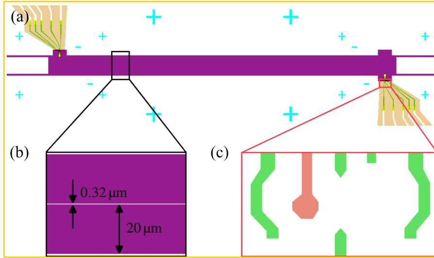
图 2.6 (a) 铌钛氮透射腔和量子点耦合样品设计图。图中紫色部分为铌钛氮透射腔，绿色的小电极为两个双量子点。(b) 放大的透射腔的结构，中心导体部分宽为 0.32\ \mu\text{m} ，离地平面的距离为 20\ \mu\text{m} 。(c) 放大的量子点结构，粉色的 plunger 电极连接到腔中心导体上，从而实现腔和量子点的耦合。
