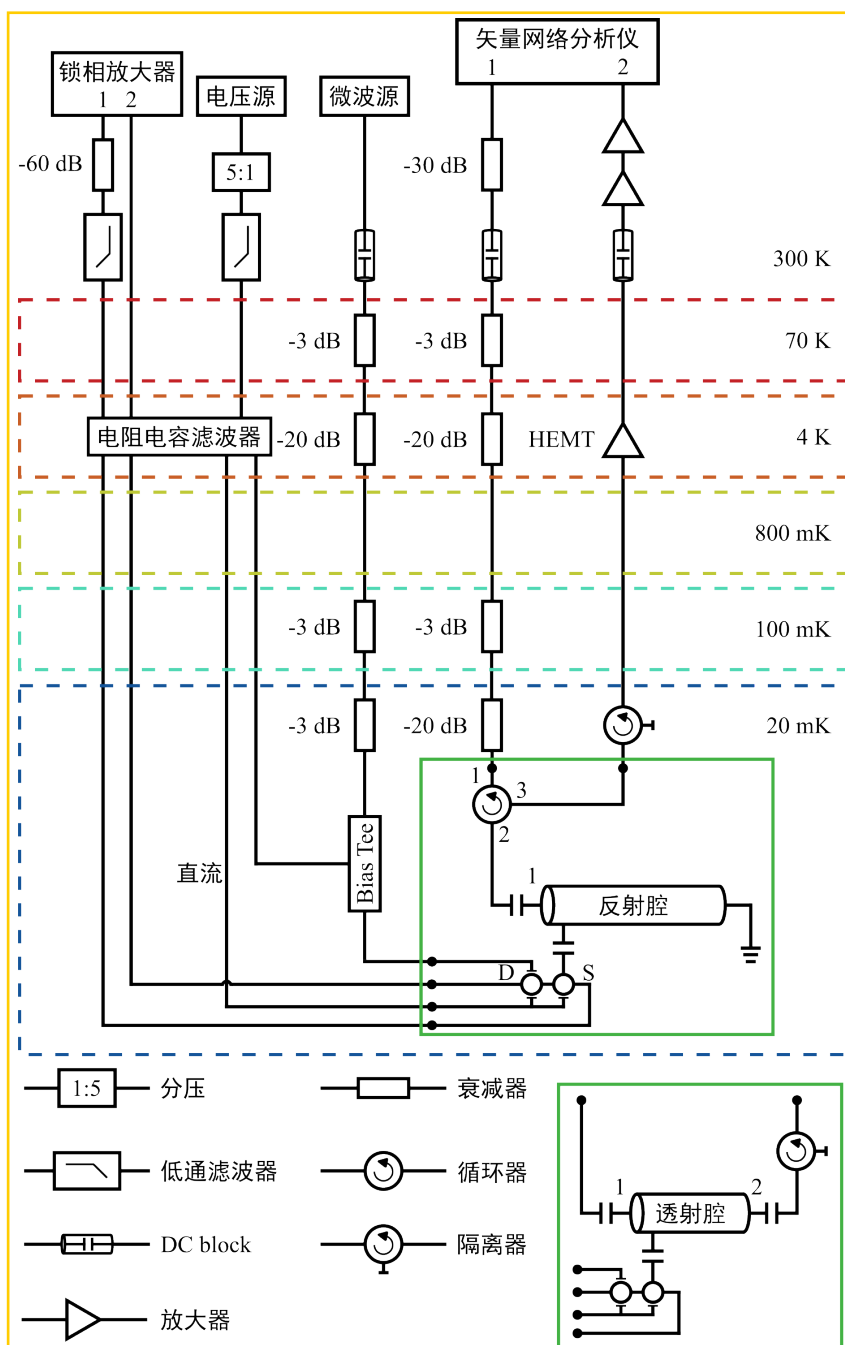
图 2.7 样品的测量线路示意图。不同颜色的虚线框代表稀释制冷机中不同的温度层。绿色实线框中为样品示意图。上面绿色方框中的为反射腔-量子点耦合的样品示意图。S 和 D 代表量子点的源漏，一个圆圈代表一个量子点。用下面绿色方框中的线路替换掉上面绿色方框中的线路，就可以得到透射腔-量子点耦合样品的测量线路。
