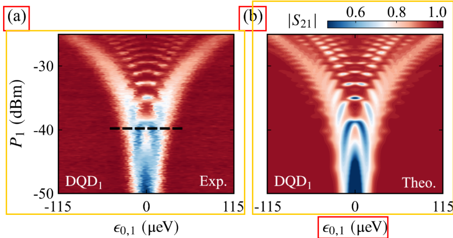
图 5.5 (a) 测量的腔透射信号幅值 |S_{21}| 随失谐偏移量 \epsilon_{0,1} 和驱动功率 P_d \propto A_{d,1}^2 变化的相图。(b) 利用响应理论计算得到的结果。这里计算时使用的参数为: \omega = \omega_c , 2t_j/\hbar = 5.2 \text{ GHz} , g_j/2\pi = 85 \text{ MHz} , f_d = 1.4 \text{ GHz} 。类似于上一章, 为了考虑准静态的电荷噪声和施加的微波幅值的抖动, 我们对计算得到的数据在 \epsilon_{0,1} 和 P_{d,1} 轴方向上都进行了高斯卷积的处理。在 \epsilon_{0,1} 轴方向上的标准差为 \sigma_\epsilon = 4 \mu\text{eV} , 而在 P_{d,1} 轴方向上的标准差为 \sigma_p = 0.1 \text{ dBm} [7,13,51]。
