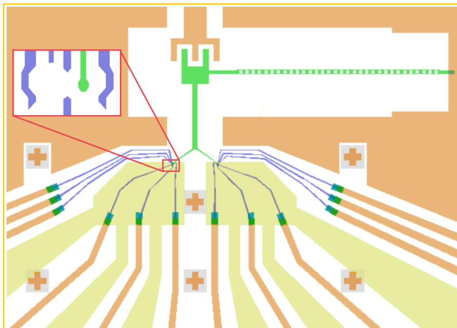
图 2.5 SQUID 阵列反射腔和量子点耦合样品设计图。图中绿色部分为 SQUID 阵列，构成了腔的中心导体，橘色部分为腔的地平面。紫色的小电极为两个双量子点，插图部分为放大的双量子点的电极结构，两个量子点的结构相同，成镜像对称。腔中心导体部分伸出一根金属导体连接到两个双量子点的 plunger 电极（绿色）上，实现腔和量子点的耦合。
