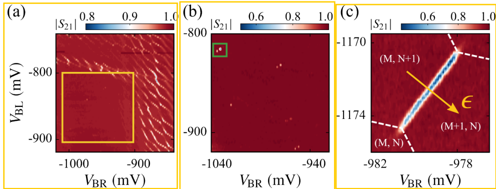
图 2.10 (a) 测得透射腔的透射幅值 |S_{21}| 、(b) 细扫的 |S_{21}| 、(c) 在量子点共振隧穿线附近的 |S_{21}| 随量子点电极电压变化的相图。图 (c) 中黄色箭头指示了量子点失谐 \epsilon 变化的方向。在测量这组数据时，我们把探测频率固定在腔频处，即 \omega = \omega_c 。
