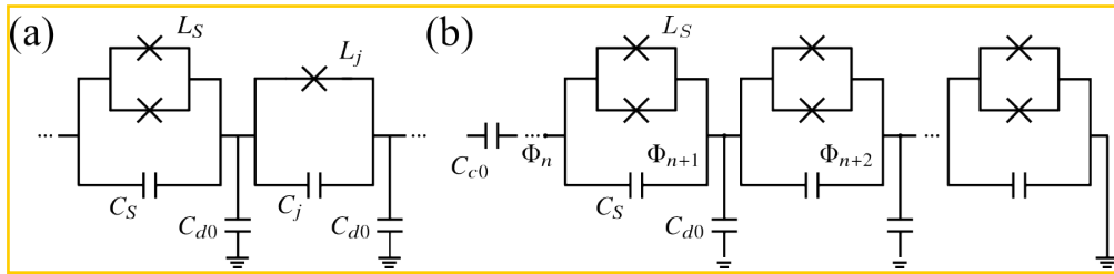
图 2.2 (a) SQUID 的电路模型示意图。(b) SQUID 阵列反射腔的电路模型示意图。 C_{c0} 为传输线和腔之间的耦合电容。
