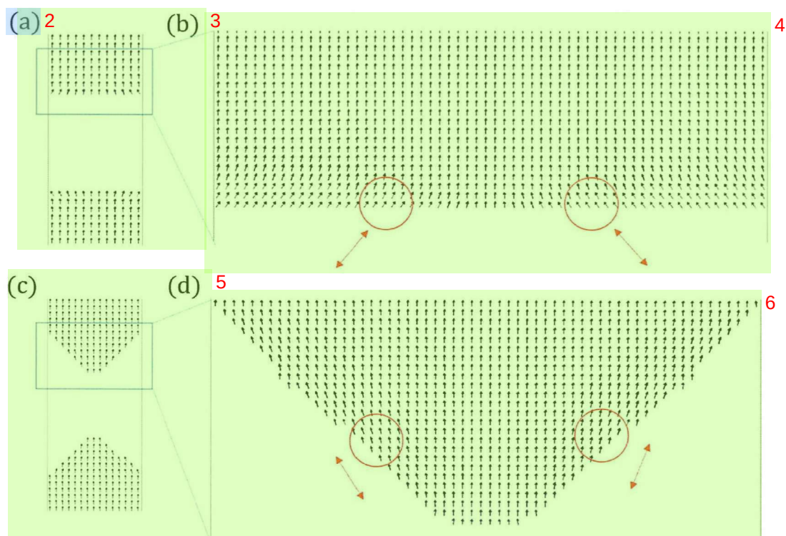
图 4.11 在 OOMMF 中模拟的微磁体磁化分布。(a) - (b) 矩形微磁体的磁化分布。(c) - (d) 多边形微磁体的磁化分布。红色双箭头是微磁体在红色圆圈内的磁化方向。
