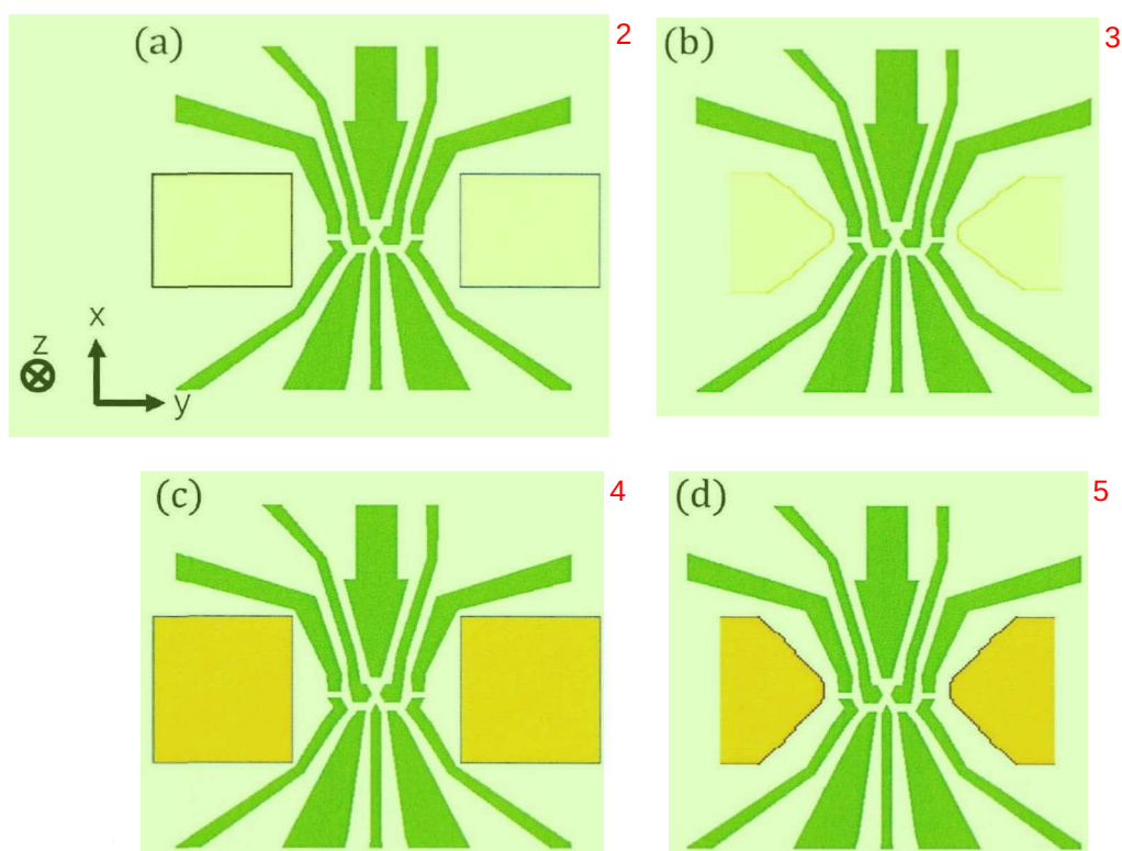
图 5.11 (a) 微磁体与栅极的多层结构，橙色半透明矩形表示在栅极上层的微磁体结构，宽度为 340 nm。(b) 微磁体与栅极的多层结构，橙色半透明多边形表示在栅极上层的最优多边形微磁体结构，宽度为 340 nm。(c) 微磁体与栅极的同层结构，橙色矩形表示与栅极同层的微磁体结构，宽度为 600 nm。(d) 微磁体与栅极的同层结构，橙色多边形表示迭代所得的同层最优微磁体结构，宽度为 600 nm。 x - y - z 坐标轴表示微磁体与量子点的相对位置。绿色电极表示栅极结构。
