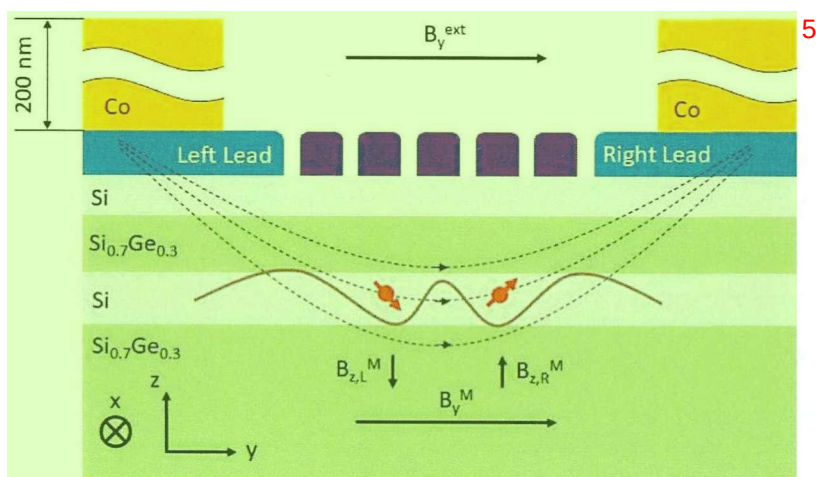
图 4.3 双量子点器件的截面示意图。黄色矩形为钴微磁体。栅电极标记为紫色，左右 lead 标记为蓝色。棕色曲线表示静电限制电势，它限制了电子的位置（以实心圆圈表示）。电子自旋（红色箭头）可以由 EDSR 控制。x-y-z 坐标轴展示了微磁体相对于量子点的位置。
