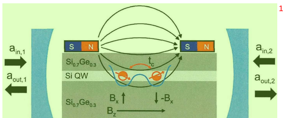
图 2.5 双量子点受外加匀强磁场 B_z 和微磁体产生的非均匀垂直磁场影响的示意图 2 。蓝色表示的微波超导腔与量子点区域的电子自旋发生耦合。微波腔场通过左端口( a_{in,1} )和右端口( a_{in,2} )被激发,输出可以在左端口( a_{out,1} )或右端口( a_{out,2} )被测量。图片引用自[88]。
