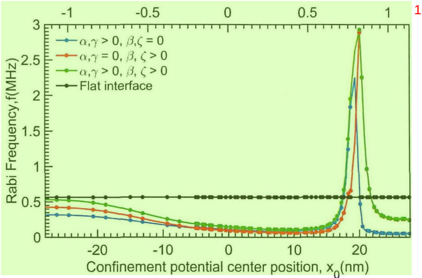
图 2.4 Rabi 频率与量子点中心位置的函数关系图，沿着(001)晶向，台阶高度为 5.43 Å，全局磁场 B = 1\text{ T} 。增强出现在台阶右侧 x_0 = 20\text{ nm} 处。图片引用自 [62]。
