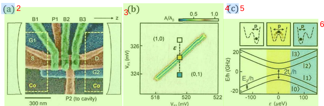
图 3.6 (a) 伪彩色 SEM 图像。微磁体的位置由黄色虚线表示。双量子点的栅极 P2 电连接超导腔的中心引脚。 2 (b) 栅极电压 V_{P1} 和 V_{P2} 在点间电荷跃迁附近的腔传输幅度 A/A_0 。 3 (c) 远失谐单点模式 ( \varepsilon \gg t_c ) 和 flopping-mode 模式 ( \varepsilon = 0 ) 的能级示意图对比。图片引用自[101]。 4 5 6 7
