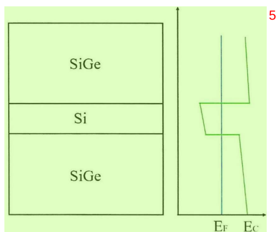
图 1.1 Si/SiGe 异质结的能带和结构的示意图。其中的绿色实线 E_C 表示载流子导带能级, 蓝色实线 E_F 表示费米能级。
