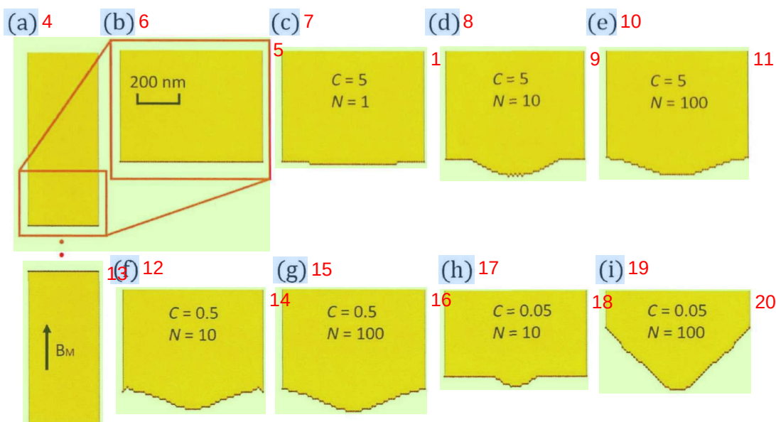
图 4.5 不同 C 参数值下的模拟结果。(a) 微磁体的初始结构。微磁体的初始间隙 21 设置为 300 nm。(b) - (e) 分别显示了当函数 R 中 C=5 时 0、1、10 和 100 次迭代的结果。(f) - (g) 和 (h) - (i) 分别是 C=0.5 和 C=0.05 时 10 次和 100 次迭代后的结果。
