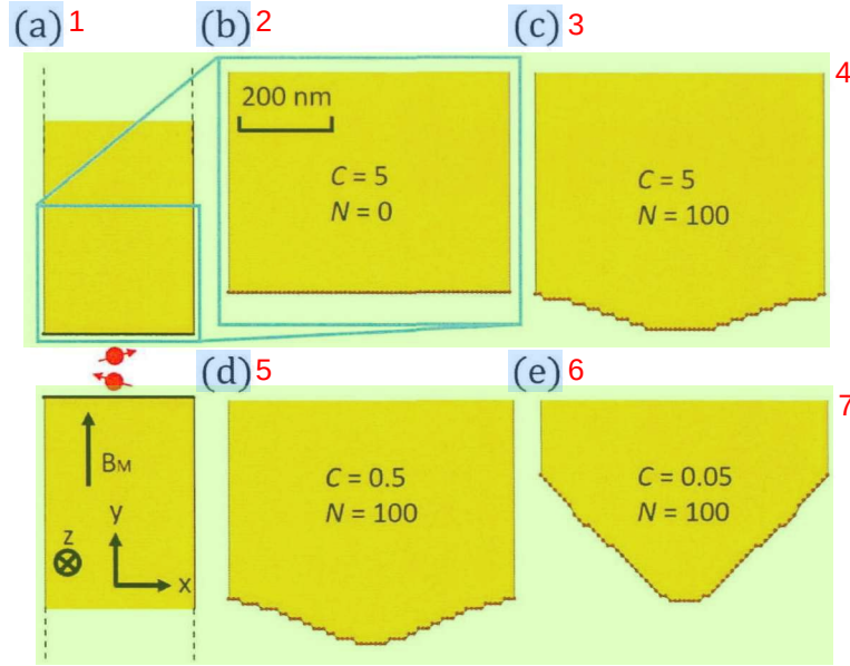
图 4.4 在不同参数 C 值下的模拟结果。(a) - (b) 微磁体的初始结构。微磁体的初始间隙设置为 300 nm。红点表示 DQD 的位置。(c) - (e) 显示了当函数 R 中的 C 值分别为 5、0.5 和 0.05 时 100 次迭代后的结果。迭代后微磁体的间隙分别为 180 nm、220 nm 和 400 nm。x-y-z 坐标轴表示微磁体与量子点的相对位置。
