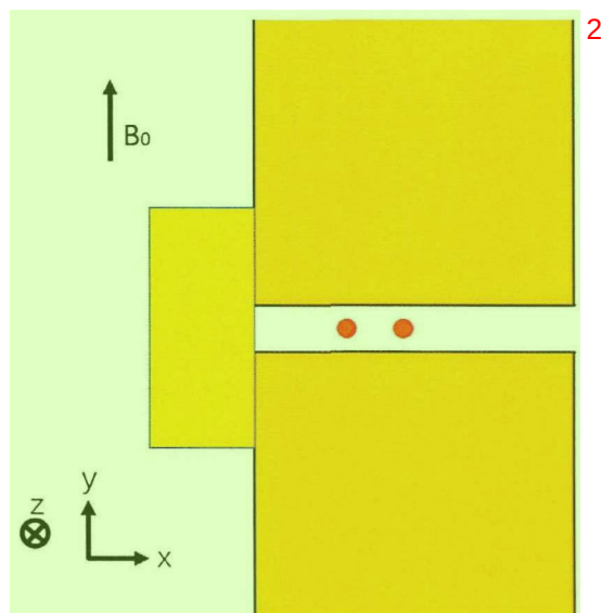
图 4.1 传统的矩形微磁体结构。x-y-z 坐标轴表示微磁体与量子点的相对位置。外磁场沿 y 轴方向，大小为 B_0 。
