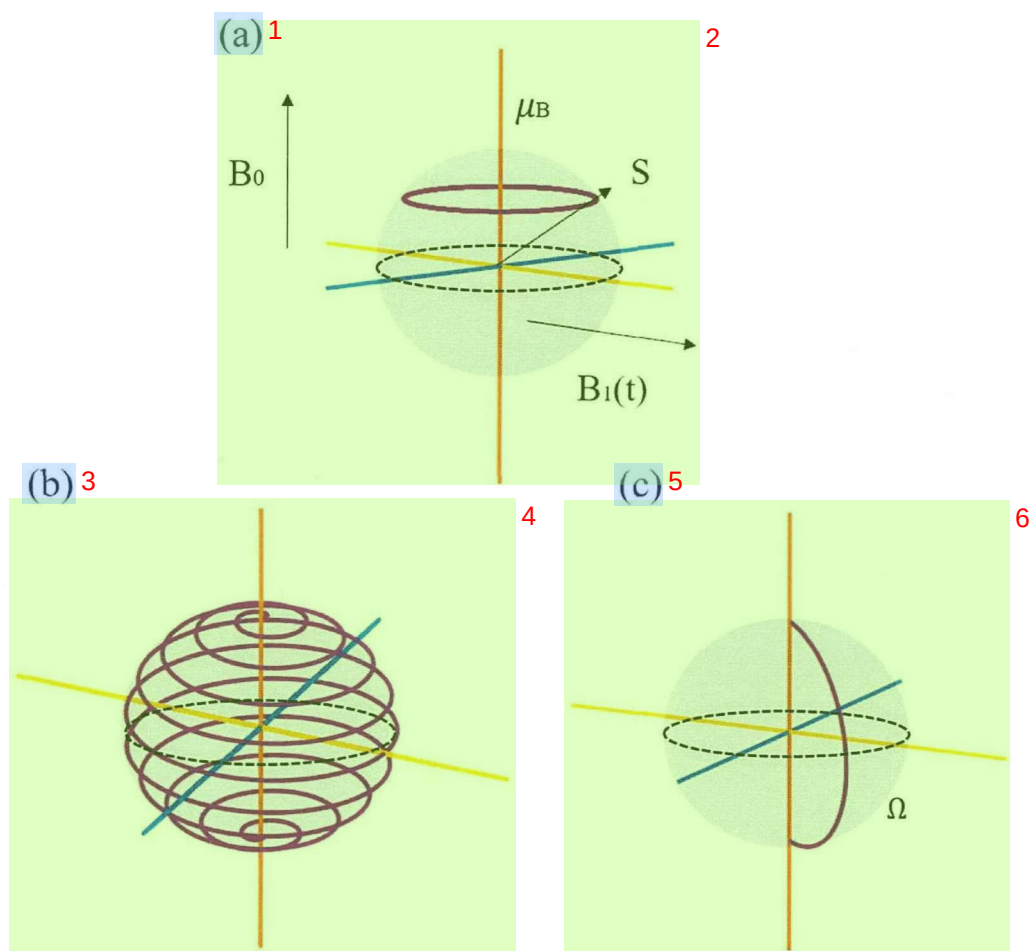
图 2.1 (a) 展示了外磁场 B_0 和交变磁场 B_1 在 Bloch 球中的方向。(b) 展示了在原坐标轴中自旋在 Bloch 球中的运动轨迹。(c) 表示了旋转坐标变换之后，自旋在新的 Bloch 球中的运动轨迹， \Omega 为自旋翻转速率。
