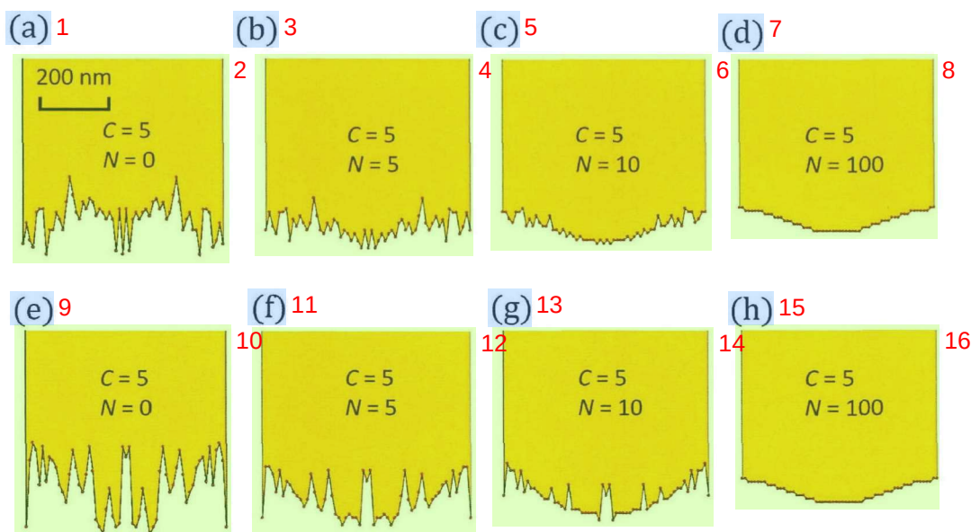
图 4.7 (a) - (d) 和 (e) - (h) 分别展示了具有不同复杂初始结构的微磁体的 0、17 5、10 和 100 次迭代的结果。可调参数 C = 5 。
