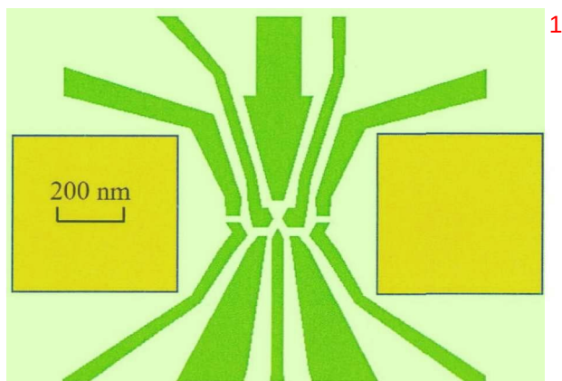
图 5.3 微磁体与栅极同层结构。绿色结构为栅极结构，橙色矩形为微磁体结构。 2
