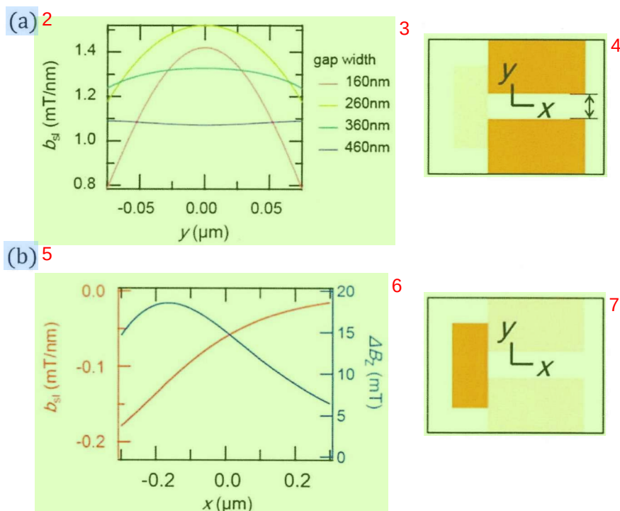
图 3.3 (a) 模拟一对具有固定间隙的微磁体的梯度磁场。右图中深橙色为突出显示模拟的微磁体部分。外磁场磁化方向沿 y 方向。微磁体间隙宽度约为 260 nm 时量子点区域的 b_{SL} 最大。(b) 仅考虑“垂直”结构部分微磁体模拟空间磁场。右图中以深橙色突出显示模拟的微磁体部分。在 |x| < 75 nm 范围内, |b_{SL}| < 0.1 mT/nm, 而 \Delta B_z > 10 mT, 可以将两个共振峰显著分离, 方便比特自旋的寻址操作。图片引用自[91]。 8
