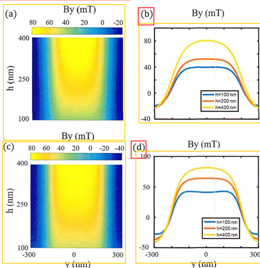
图 5.8 (a) 多层结构 d=70\text{ nm} 时，模拟绘制的 B_y 与微磁体厚度 h 和轴上位置 y 的二维关系图。(b) 蓝线，红线和黄线分别代表图 (a) 中 h=100\text{ nm} 、 h=200\text{ nm} 和 h=400\text{ nm} 处的切面图。绿线与三条曲线的交点展示了 y=50\text{ nm} 处 (量子点位置)，有害磁场梯度 b_{\text{deph}} (曲线交点处斜率) 的大小。(c) 同层结构 d=50\text{ nm} 时，
