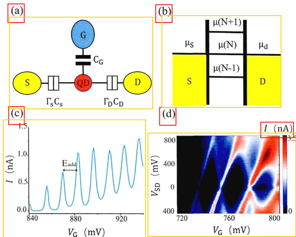
图 1.2 (a) 单量子点器件结构图。左右的黄色椭圆分别表示源极 S 和漏极 D, 蓝色椭圆表示栅极 G, 红色圆表示量子点, 量子点与 S 和 D 的隧穿耦合强度分别为 \Gamma_S 和 \Gamma_D , 量子点到 S 和 D 的电容耦合分别为 C_S 和 C_D , C_G 是量子点到栅极 G 的电容耦合。(b) 电子能级与 \mu_S 或者 \mu_D 齐平时的单量子点的电子输运示意图。(c) 单量子点在实验中测得的库伦峰曲线图。(d) 单量子点通过调节栅极电压 V_G 和源漏极电压差 V_{SD} , 在实验上测得的库伦菱形图案。图片引用自[42]。
