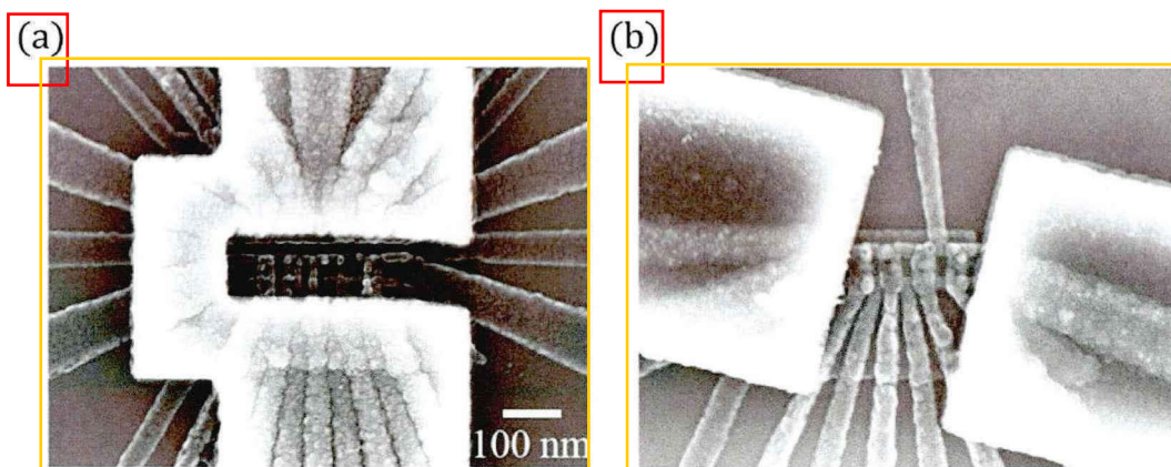
图 5.2 (a) 电子显微镜拍摄的带微磁体的一维四量子点阵列器件。(b) 电子显微镜拍摄的微磁体旋转 15 度的自旋比特与腔耦合器件。
