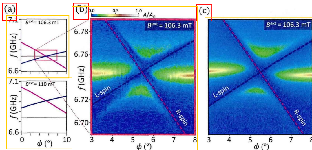
图 3.5 (a) B^{ext} = 106.3 mT (上图) 和 B^{ext} = 110 mT (下图) 时, 角度 \phi 与驱动频率 f 的函数关系图。L 和 R 自旋的共振频率分别以蓝色和紫色绘制。(b) A/A_0 作为驱动频率 f 和角度 \phi 的函数, B^{ext} = 106.3 mT, \phi = 5.6^\circ 时, 两个自旋同时与腔共振。(c) A/A_0 的理论预测图。图片引用自[99]。
