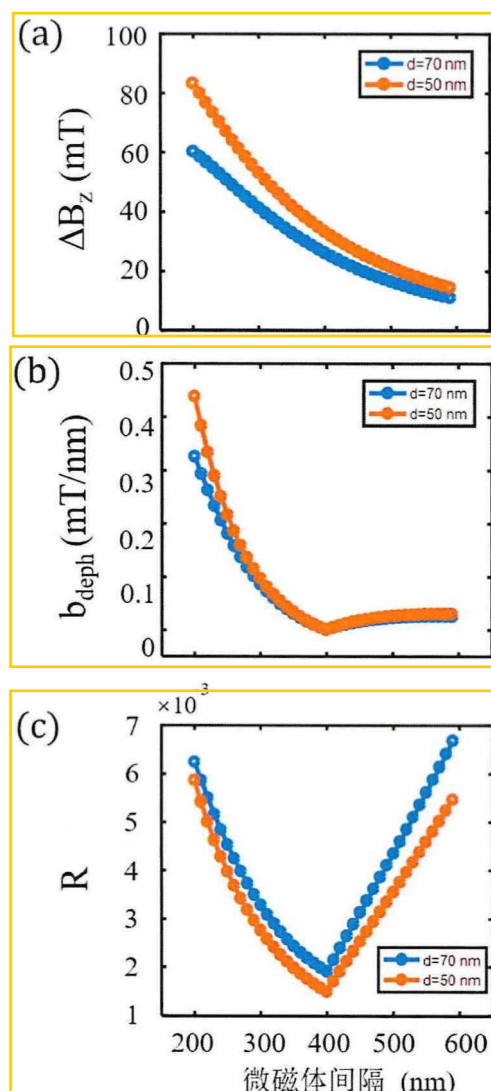
图 5.9 (a) \Delta B_z 与微磁体间隔的关系图。(b) b_{deph} 与微磁体间隔的关系图。(c) 目标函数 R 与微磁体间隔的关系图。蓝色和红色分别对应多层结构 ( d=70 nm) 和同层结构 ( d=50 nm)。
