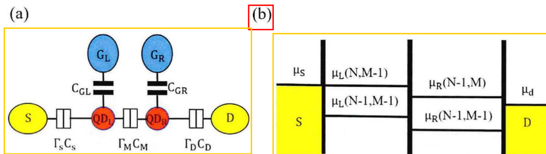
图 1.3 (a) 双量子点器件结构图。左右的黄色椭圆分别表示源极 S 和漏极 D, 左右的蓝色椭圆表示左右栅极 G_L 和 G_R , 左右的红色圆表示左右量子点 QD_L 和 QD_R , 量子点到 D 和 S 的隧穿耦合分别为 \Gamma_D 和 \Gamma_S , \Gamma_M 为左量子点和右量子点之间的隧穿耦合, 量子点到 D 和 S 的电容耦合分别为 C_D 和 C_S , C_M 左量子点和右量子点之间的电容耦合, 左右量子点到栅极 G_L 和 G_R 的电容耦合分别为 C_{GL} 和 C_{GR} 。
