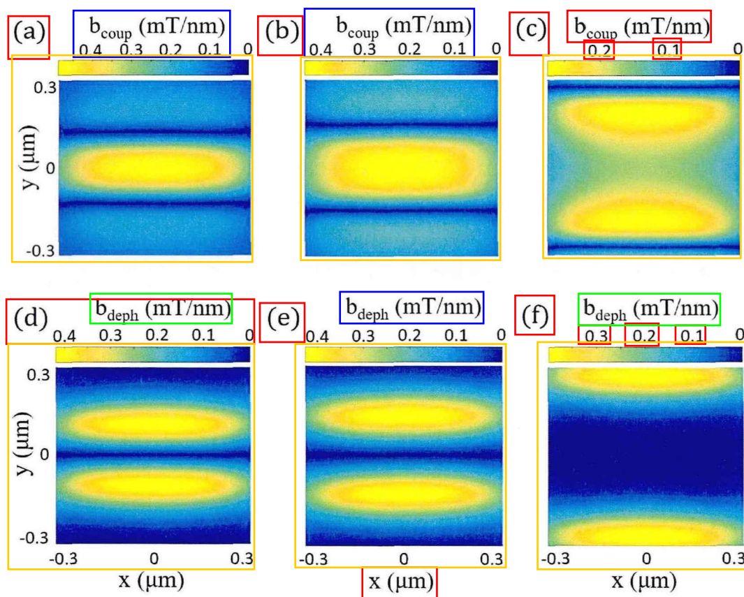
图 4.6 (a) - (c) 180 nm, 240 nm 和 420 nm 间隔下矩形微磁体的磁场梯度 b_{\text{coup}} 。(d) - (f) 180 nm, 240 nm 和 420 nm 间隔下矩形微磁体的有害的微磁体梯度 b_{\text{deph}} 。
