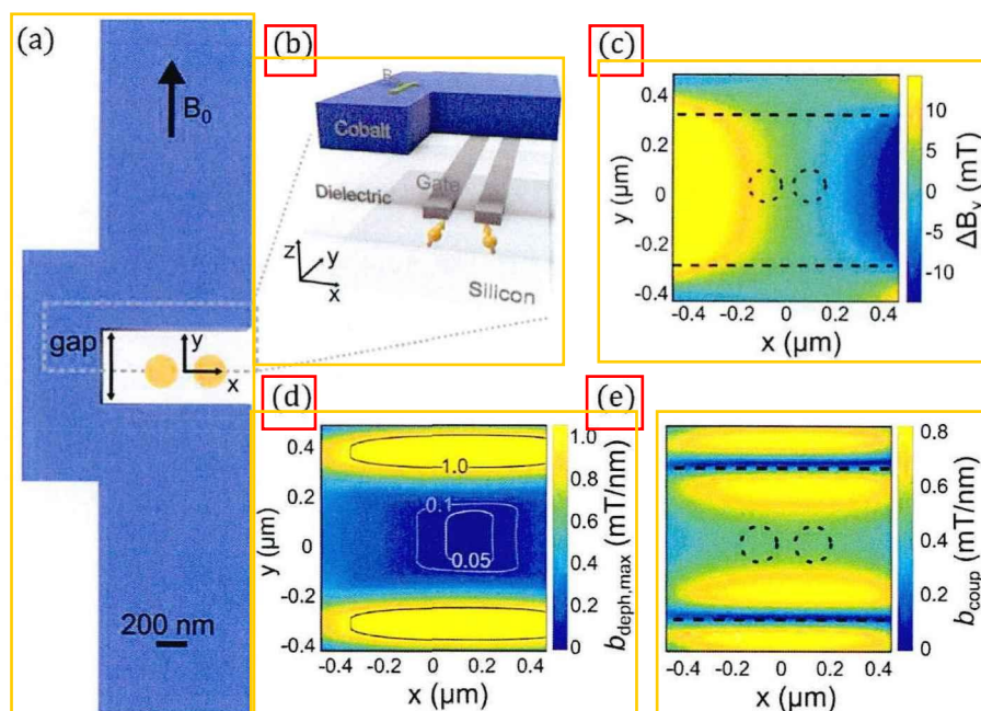
图 3.8 (a) 微磁体的结构。x-y-z 坐标轴表示微磁体与量子点的相对位置。(b) 微磁体的 3D 结构。(c) 沿量子点连线方向(x 方向)的磁场差与空间位置的关系图。(d) 磁体产生的有害磁场梯度与空间位置的关系图。(e) 磁体产生的有效耦合磁场梯度与空间位置的关系图。虚线圆圈表示量子点的位置，水平虚线表示微磁体的轮廓。图片引用自[104]。
