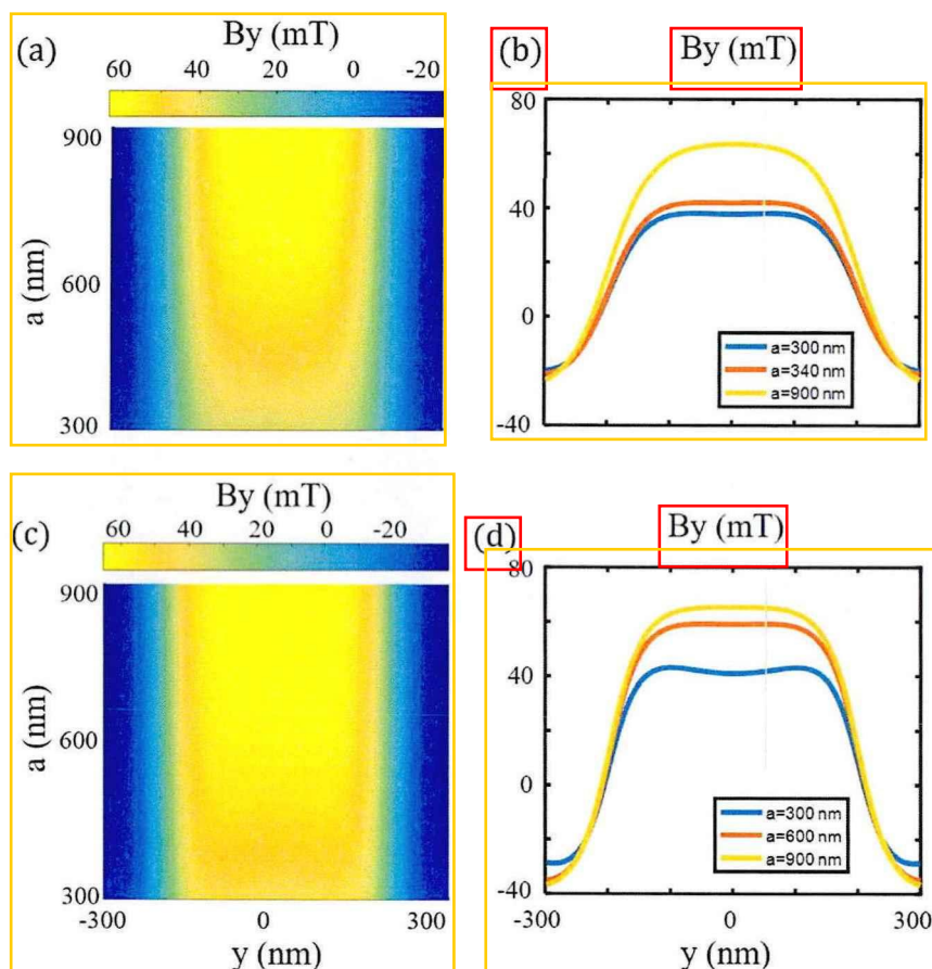
图 5.6 (a) 多层结构 d=70\text{ nm} 时，模拟绘制的 B_y 与微磁体宽度 a 和轴上位置 y 的二维关系图。(b) 蓝线，红线和黄线分别代表图 (a) 中 a=300\text{ nm} 、 a=340\text{ nm} 和 a=900\text{ nm} 处的切面图。绿线与三条曲线的交点展示了 y=50\text{ nm} 处（量子点位置），有害磁场梯度 b_{deph} （曲线交点处斜率）的大小。(c) 同层结构 d=50\text{ nm} 时，模拟绘制的 B_y 与微磁体宽度 a 和轴上位置 y 的二维关系图。(d) 蓝线，红线和黄线分别代表图 (c) 中 a=300\text{ nm} 、 a=600\text{ nm} 和 a=900\text{ nm} 处的切面图。绿线与三条曲线的交点展示了 y=50\text{ nm} 处，有害磁场梯度 b_{deph} 的大小。
