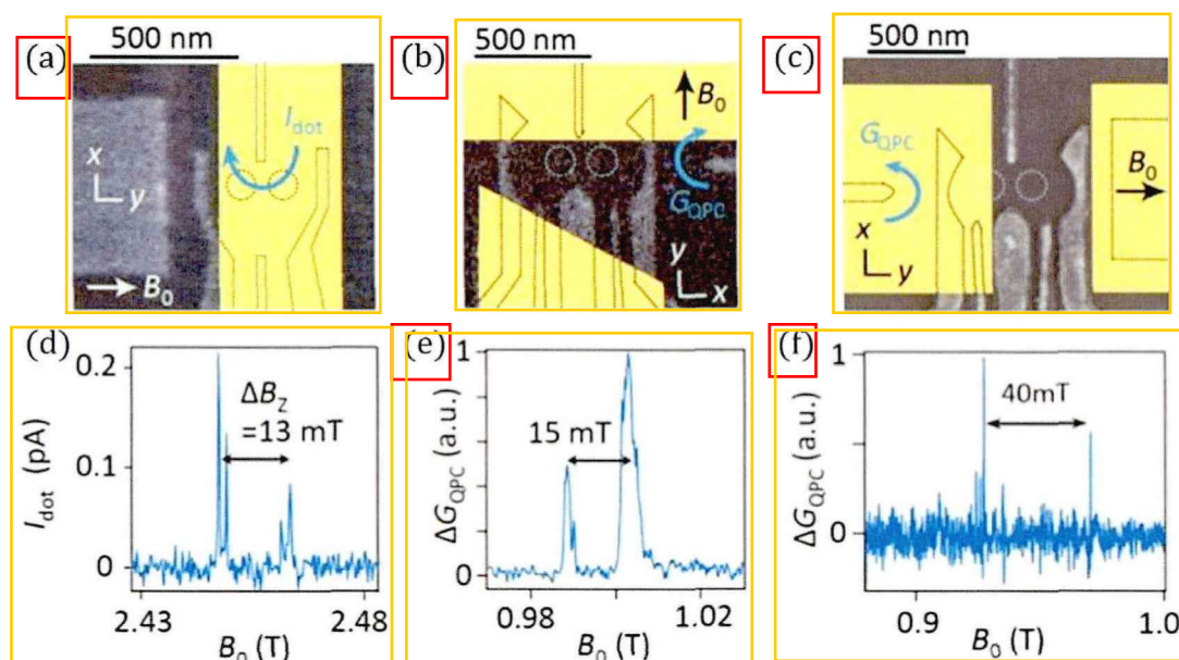
图 3.2 (a) - (c) 顶部带有伪彩色钴微磁体的 GaAs 量子点器件的扫描电子显微照片。GaAs/AlGaAs 基片上的金属栅定义了量子点的静电势能,二维电子气在表面下约 90 \text{ nm} 处。 160 \text{ nm} 厚的微磁体沉积在约 100 \text{ nm} 厚的绝缘层的顶部,并在 B_0 \geq 1 \text{ T} 的平面内外加磁场下磁化。当输入的驱动频率与其自旋发生共振时,自旋态会发生翻转。(d) - (f) 分别在这些器件中测量的 ESR 谱 [95] 。图片引用自[91]。
