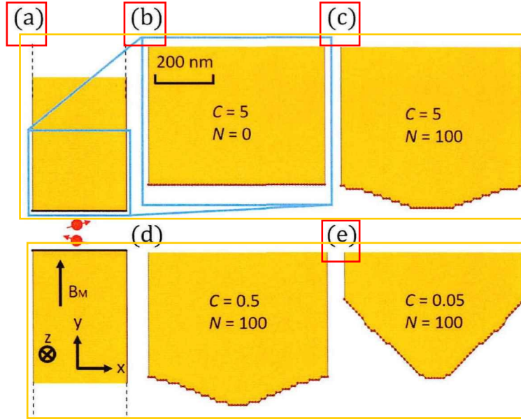
图 4.4 在不同参数 C 值下的模拟结果。(a) - (b) 微磁体的初始结构。微磁体的初始间隙设置为 300 nm。红点表示 DOD 的位置。(c) - (e) 显示了当函数 R 中的 C 值分别为 5、0.5 和 0.05 时 100 次迭代后的结果。迭代后微磁体的间隙分别为 180 nm、220 nm 和 400 nm。 x - y - z 坐标轴表示微磁体与量子点的相对位置。
