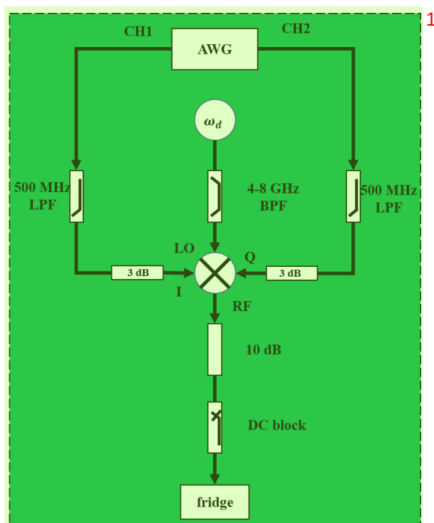
图 3.2.3 用于生成单个 qubit 的 XY-control pulse 的 IQ 混频调制线路。 2
