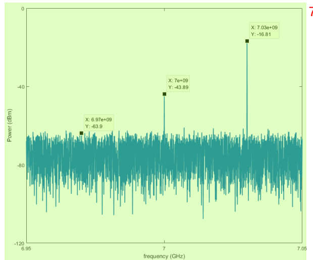
图 5.2.2 使用频谱仪校准 IQ 混频器。
