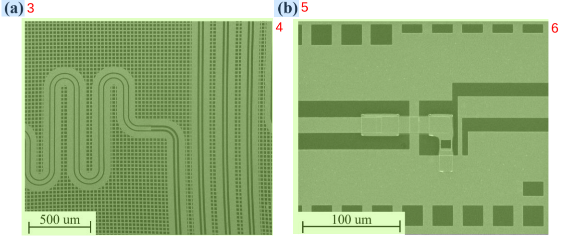
图 3.5.2 J-IMP A 的 SEM 电镜照片。其中 (a) 是阻抗变换线结构, 由于第一段为信号 7 引入段, 因此没有给出, 图中的结构从左到右分别为四分之一波长传输线以及二分之一波长传输线; (b) J-Amp 结构, 其中电容结构为 Al-AlO x -Al 平行板电容器, AlO x 氧化层为第一层铝膜在纯氧干燥腔体中原位氧化 12h 制备出来。
