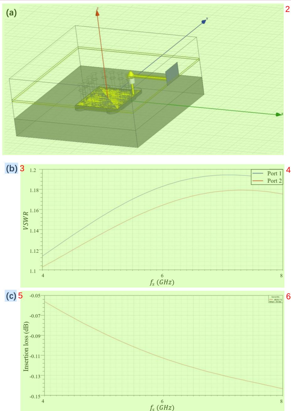
图 3.6.6 (a) 改进弹簧针结构后的整体模型; (b) 整体 VSWR; (c) 整体插入损耗。
