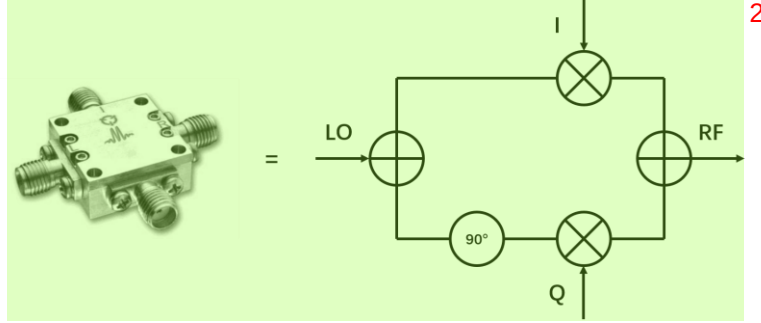
图 5.2.1 IQ mixer 及其内部等效电路。
