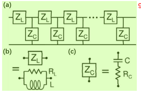
图 A.2 (a) 谐振腔的等效电路结构； (b) (c) 分别为 (a) 中基本单元的等效电路。 10
