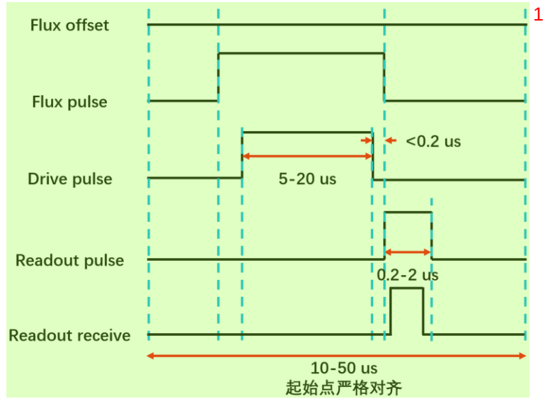
图 5.1.3 典型的单比特读取脉冲时序关系图。 2
