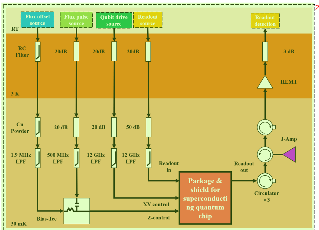
图 3.2.1 改造后的稀释制冷机的低温测控线路示意图。
