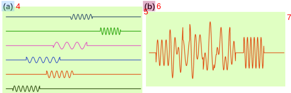
图 3.2.5 (a) 使用 6 路 IQ 混频线路方式生成的 6 路 readout 调制信号；(b) 使用 1 路 IQ 混频线路合成时，AWG 实际输出的波形，该波形与 (a) 实际效果完全一致。
