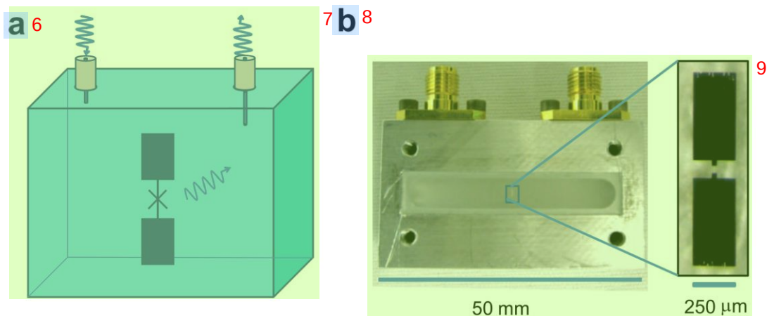
图 3.8.1 (a) 3D 腔示意图结构示意图，中心放置的是一个 transmon qubit。(b) 3D 腔实物图。它具有两个微波端口，一进一出，transmon qubit 放置在 3D 腔中心，与 3D 腔的 TE101 模式耦合，3D 腔中心恰好是 TE101 模式的电场强度最大处。引自[49]。 10
