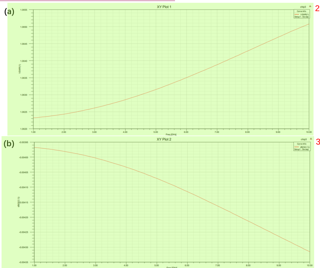
图 3.6.3 信号通过弹簧针到 quantum chip 上的信号 pad 的 (a) VSWR 与 (b) 插入损耗。 4
