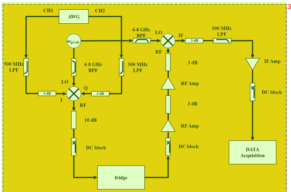
图 3.2.4 基于 IQ 多点频混频调制线路的 qubit readout 线路。 4
