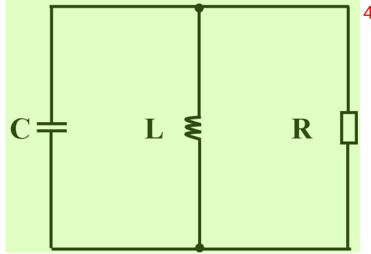
图 A.1 并联 LCR 振荡电路。 5
