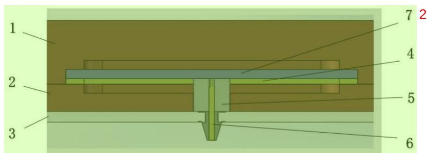
图 3.6.1 立体封装结构剖面图。图中 1——固定腔；2——对准腔；3——带热沉的 PCB 板；4——铜皮；5——聚四氟乙烯套；6——弹簧针；7——quantum chip。 3
