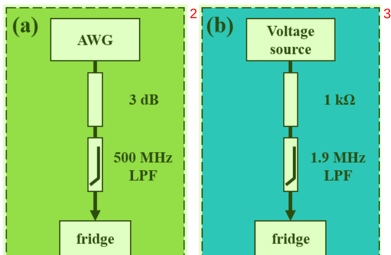
图 3.2.2 用于生成单个 qubit 的 Z-control pulse 的 (a) flux pulse 源以及 (b) flux offset 源。
