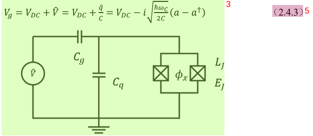
图 2.4.2 Transmon 与 CPW 耦合的等效电路示意图。 4
