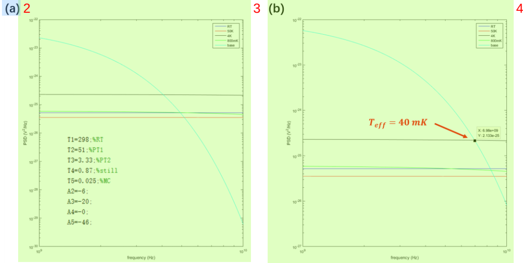
图 3.3.4 (a) 在图 C.3 基础上，我们在 mc 层加了 46dB 衰减，各级到读取腔的噪声谱分布，其中 mc 温度取 25mK，横轴范围为 1-10GHz，纵轴范围为 10^{-22} - 10^{-30} V^2/Hz ； (b)对应(a)图，读取腔的实际等效温度被有效地降低到 40mK。
