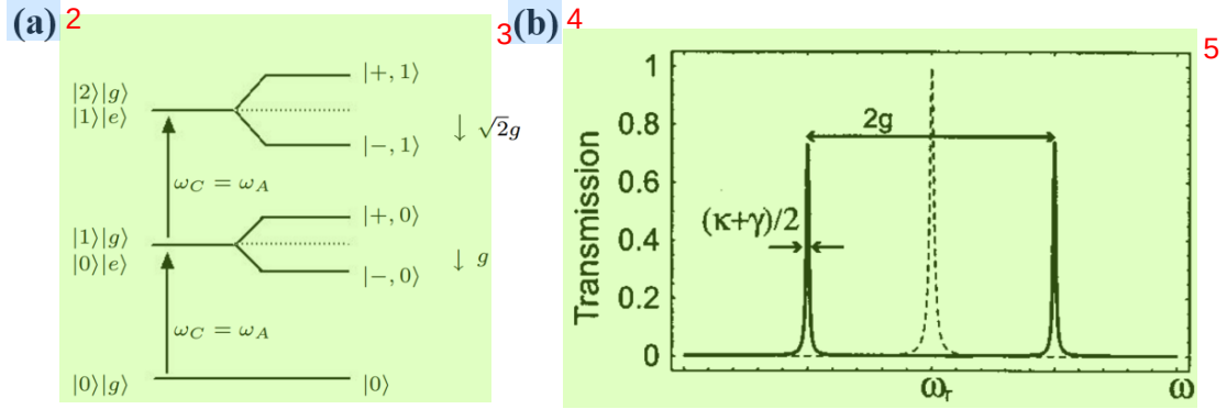
图 2.1.2 (a) \Delta = 0 时 J-C 模型对应的能级简图；(b) 满足公式 (2.1.16) 时 dressed 态原子与真空光子相互作用时的能级频谱分布，引用自[3]。 6
