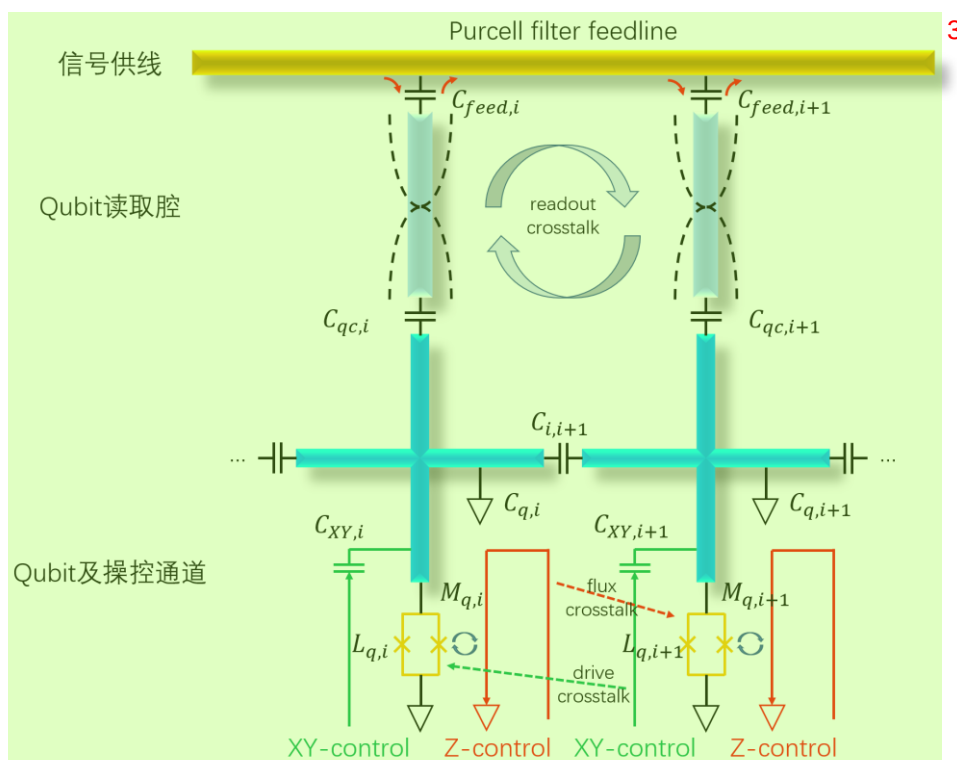
图 2.7.1 多 qubit 超导量子芯片结构设计示意图
