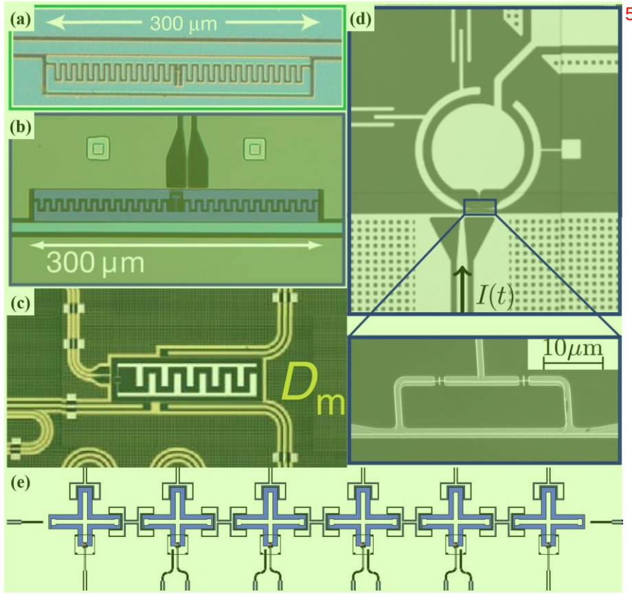
图 2.2.4 (a) 2007 年 Yale 的 Schoelkopf 组的 transmon[16]，电容部分为交指电容； 6 (b) 2009 年 Yale 的 Schoelkopf 组的 transmon[17]，相比两年前的结构，大体上没有变化，参数设计、加工工艺更加精致； (c) 2014 年 Delft 的 Dicarlo 组的 transmon[18]，他们把原有对称的交指电容去掉了一半，更加便于施加 qubit 调控信号； (d) 2017 年 Rigetti Computing 的 transmon[19]，在他们的结构中，电容结构为圆形的分布式电容，寄生参数得到了降低； (e) 2018 年我们实验室最新 6 个 transmon qubit 一维耦合阵列的芯片结构设计图。
