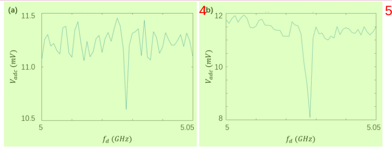
图 5.3.1 (a) 一条需要优化的能谱数据，在该数据中，drive 功率合适，也测到了 qubit 能谱在 5.027GHz 附近，但是能谱噪声较大，并且信噪比不高；(b) 优化后的能谱数据，我们将 probe 功率增大了 2dB，微调了 probe 的频率，并缩短了采集卡所采集的数据长度（从 900ns 缩短至 600ns）。我们可以看到，能谱本底有一定程度的提高，但其抖动大幅降低，同时 qubit 能谱的有效信号增大，读取信噪比大幅提高。
