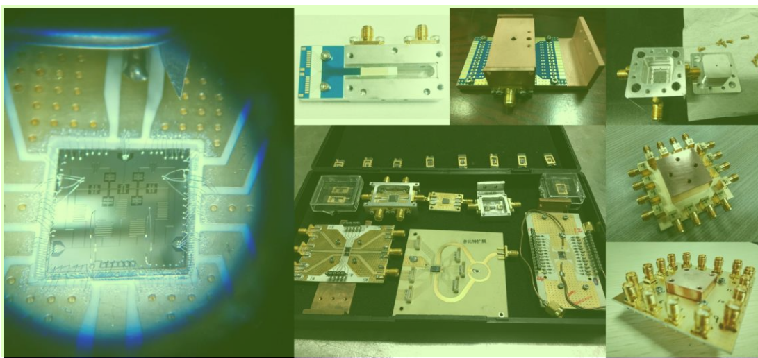
图 3.3.1 大量的量子芯片封装盒以及正在封装中的量子芯片实物照片。 4
