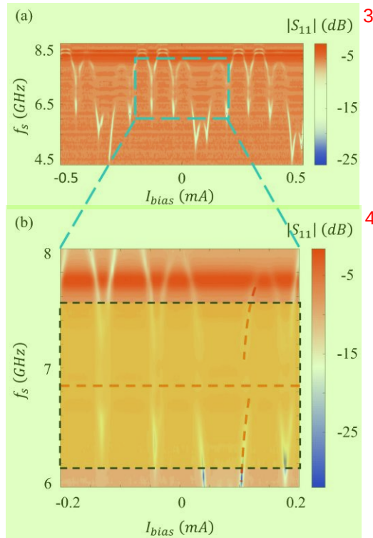
图 3.5.5 (a) 当 P_s = -120\text{dBm} 时 J-IMPA 的磁通调制性质；(b) 图 (a) 中蓝色虚线框内区域的细扫。
