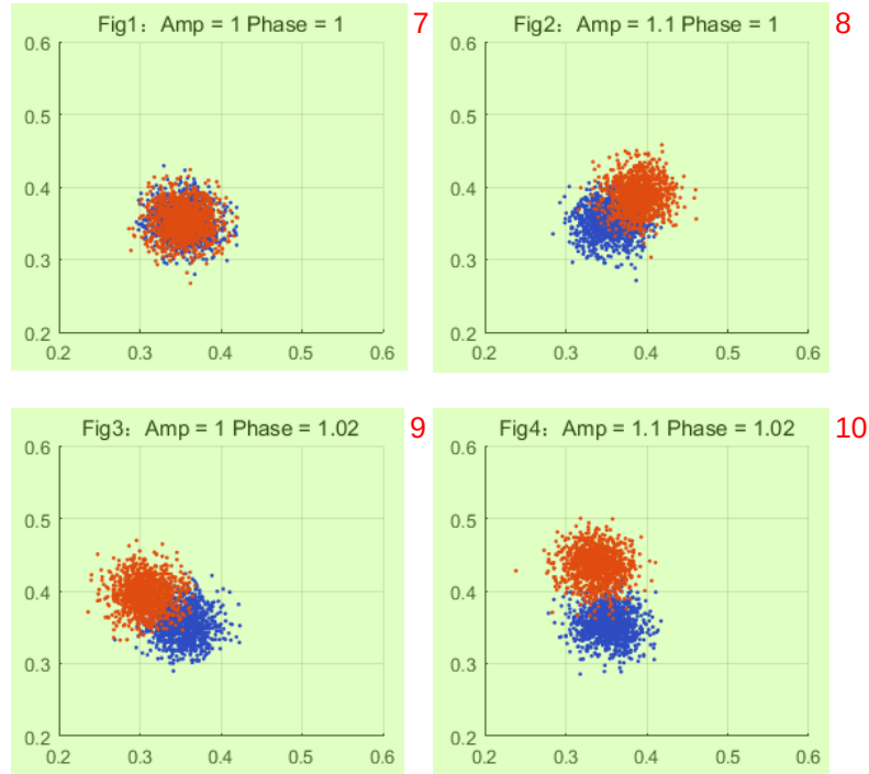
图 3.2.6 数字 IQ 解调示意图。横轴为 I，纵轴为 Q，采集到的原始数据经过转化后落在 IQ 坐标轴下的对应位置上。在此我们通过引入具有不同中心位置的高斯分布的形式来还原针对 qubit 的 |0\rangle 态（蓝色）与 |1\rangle 态（红色）的有限读取信噪比。 11
