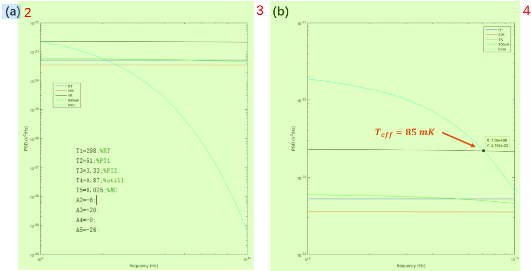
图 3.3.3 (a) 一种典型的错误衰减器施加方案，各级温度以及施加的衰减器见小图。在 5 该方案下，制冷机各级到读取腔的噪声谱分布，其中 mc 温度取 25mK，横轴范围为 1-10GHz，纵轴范围为 10^{-22} - 10^{-30} \text{V}^2/\text{Hz} ； (b) 对应 (a) 图，读取腔的实际等效温度高达 85mK。
