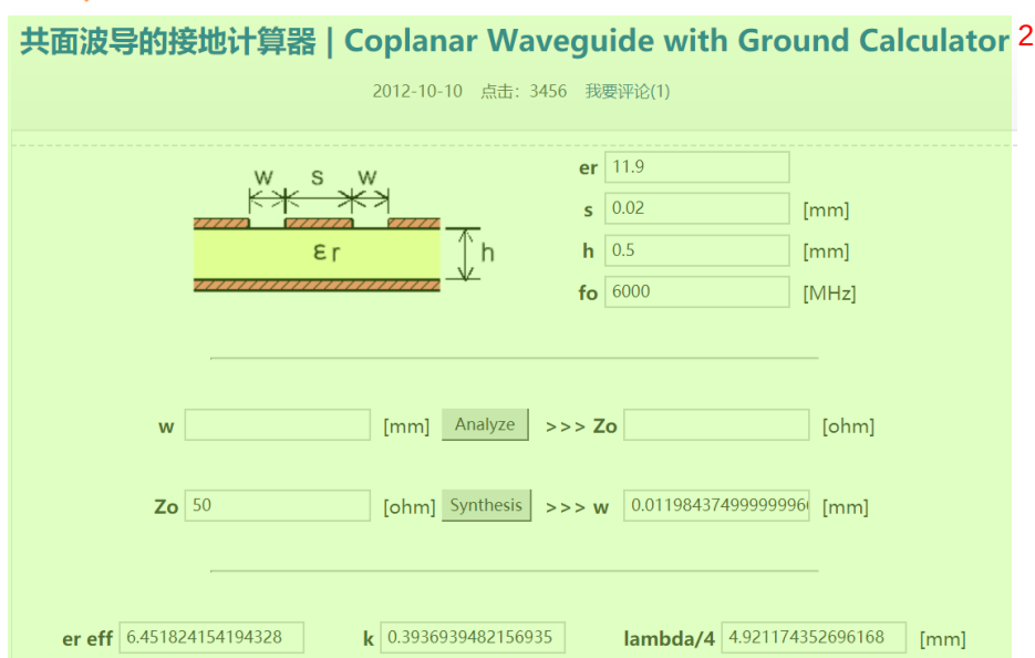
图 2.3.1 共面波导的接地计算器界面
