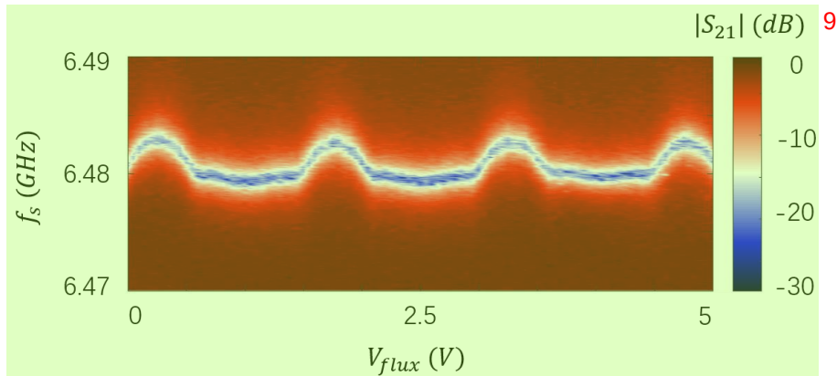
图 5.1.2 设定 P_s = -120 \text{ dBm} ，使用网络分析仪获取的读取腔随着 V_{flux} 的周期性变化。 10
