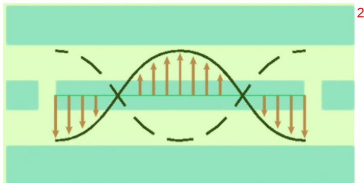
图 2.3.2 半波长共面波导传输线谐振腔的结构以及共振模式下信号的电压幅度分布示意图，可见电场主要分布在谐振腔的两个端口处。引自[14]。
