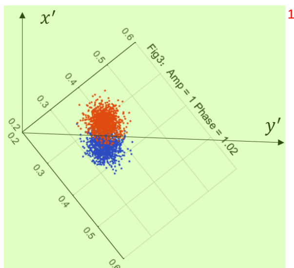
图 3.2.7 数字 IQ 解调示意图。通过调节标准数字信号中的相位 \phi ，将所有信息保留到新的坐标轴 x' 上，以最大化读取信噪比。
