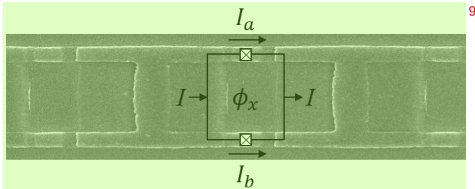
图 2.2.3 一种 SQUID 链状结构的 SEM 照片。
