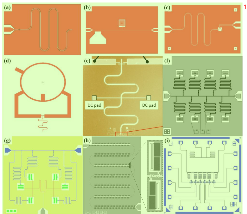
图 2.3.3 (a) 一种 \lambda/4 反射腔设计图； (b) 一种 \lambda/2 透射腔设计图； (c) 一种 \lambda/4 反射腔式 JPA 设计图； (d) 一种引入了 180^\circ 反向环的差分带线反射腔设计图； (e) 一种差分带线反射腔的光显照片，该结构用于研究和两个石墨烯双量子点的耦合[26]-[27]； (f) 一种 8-qubit 测试芯片设计图； (g) 一种引入了多终端可调量子数据总线的 6-qubit 测试芯片设计图； (h) 一种以约瑟夫森结链改造的传输线式行波参量放大器 (J-TWPA) 的设计图； (i) 一种引入传输线信号供线的 6-qubit 测试芯片设计图。
