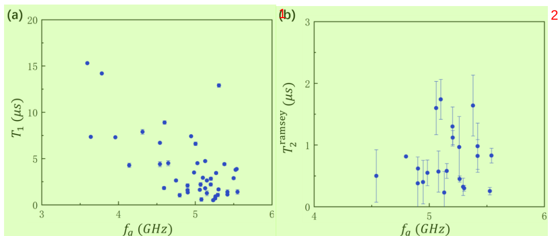
图 3.7.1 Qubit 相干时间统计数据，截止到 2018 年 4 月 1 日。 3
