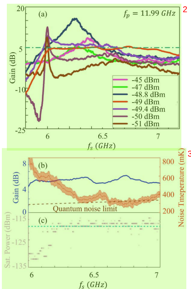
图 3.5.9 (a) 当 f_p = 11.99 \text{ GHz} 时改变 pump 功率，所得到的 J-IMPA 增益曲线变化关系，特别是当 P_p = -49 \text{ dBm} 时（红色曲线），我们得到了非常平坦的增益曲线，在 1.2 GHz 的 3 dB 带宽内有非常稳定的 5 dB 增益，5 dB 阈值用虚线标出；(b) P_p = -49 \text{ dBm} 时对应的带 error-bar 的噪声温度曲线（红色曲线）与量子噪声极限曲线（褐色曲线）对比图，增益也画在同一张图中，见蓝色曲线；(c) P_p = -49 \text{ dBm} 时对应的信号饱和功率曲线，浅蓝色虚线标出的是 -120 dBm 的阈值。
