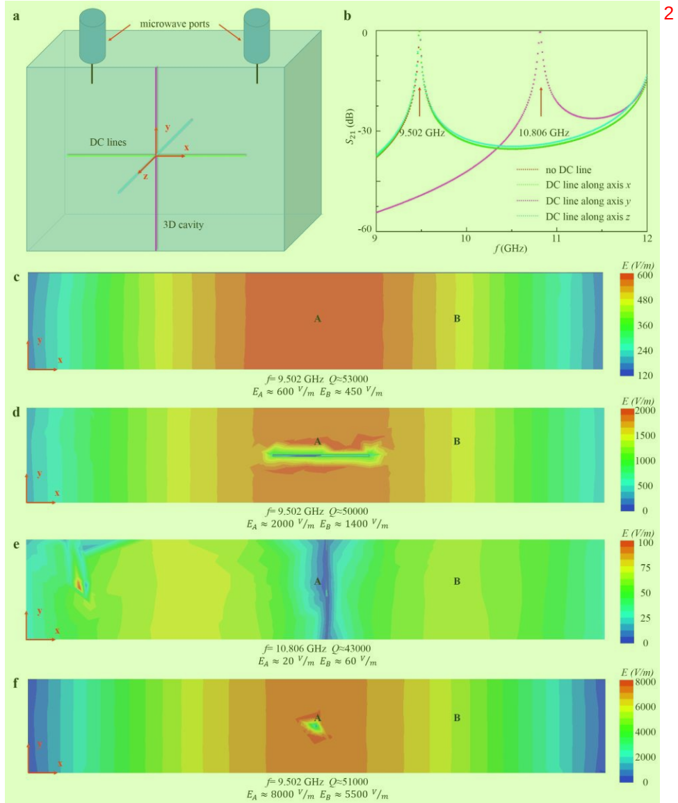
图 3.8.3 引入直流调控的 3D 微波谐振腔 HFSS 仿真结果。(a) 仿真结构示意图，其中，x, y, z 为所研究的三个直流电极引入的方向。微波通道的方向为 y 方向。(b) HFSS 仿真得到的 S_{21} 随电极引入方向的不同结果。我们发现，DC 电极引入方向为 y 方向时，会严重破坏 TE 101 模式，而其他的引入方式对 TE 101 模式几乎没有影响。(c) – (f) 分别为不引入直流电极、引入一根 x 方向电极、引入一根 y 方向电极、引入一根 z 方向电极所导致的 xy 平面电场分布剖面仿真图。从结果来看，沿着 y 方向引入电极已经完全破坏了 TE 101 的模式。而沿着 x, z 方向引入电极，仅会使得电极周围局部区域电场强度减弱，但不会导致 TE 101 模式的变化。
