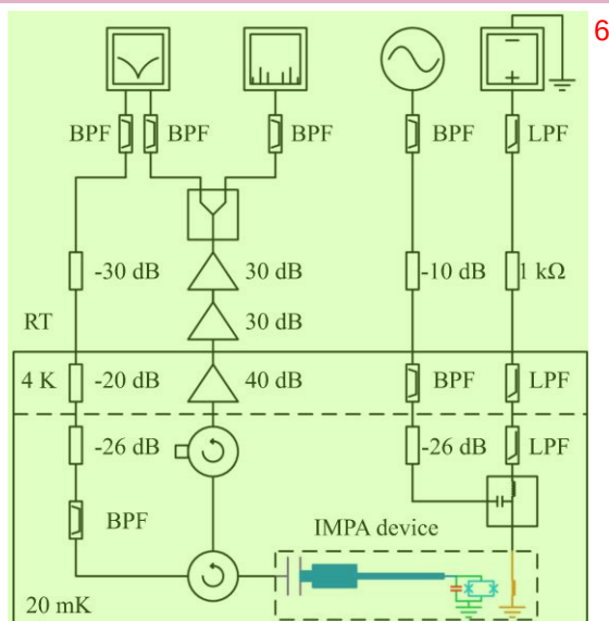
图 3.5.4 flux-pump 工作模式下 J-IMPA 的测试电路。
