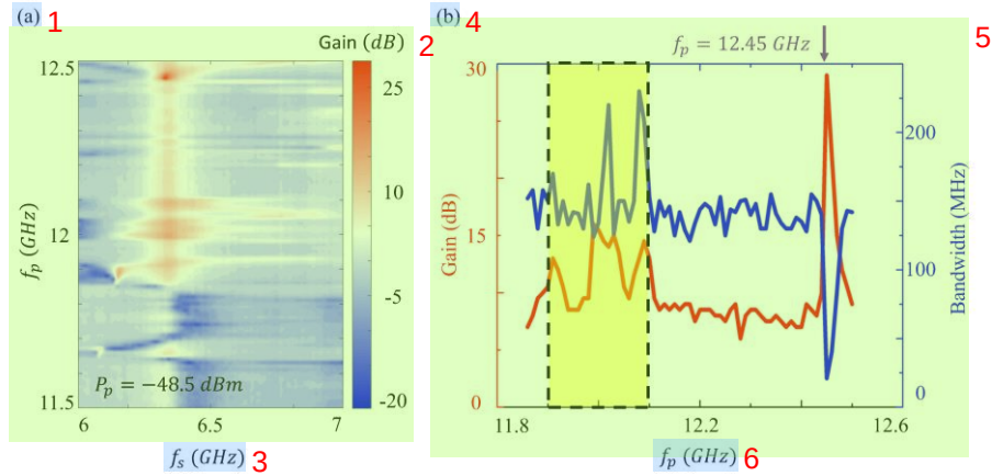
图 3.5.8 (a) f_{J-Amp} \approx 6.23 \text{ GHz} 时放大器在 flux-pump 模式下的增益性质。我们设定到样品的 pump 功率为 P_p = -48.5 \text{ dBm} ，然后在 11.5\text{--}12.5 \text{ GHz} 范围内扫描 f_p ；(b) 从 (a) 图中提取出的增益/增益带宽随 f_p 的变化关系，我们发现，在标黄区域内，当 f_p \sim 11.9 - 12.1 \text{ GHz} 时，放大器的增益以及增益带宽得到了同时增强，除此以外， f_p = 12.45 \text{ GHz} \approx 2f_{J-Amp} 时，具有尖峰增益同时增益带宽锐减。
