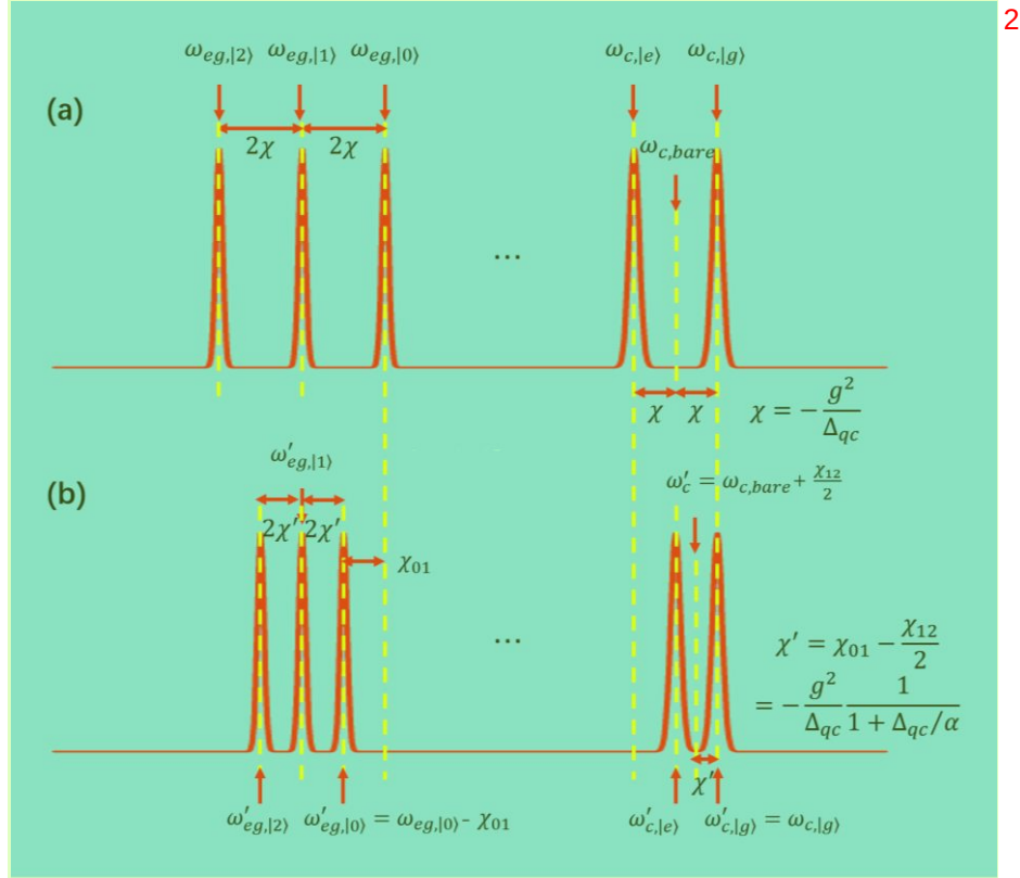
图 2.4.3 由 transmon qubit 与 CPW 构成的 dispersive-strong coupled circuit QED system 的能级结构示意图。(a) 为理想的二能级原子；(b) 为考虑第二激发态修正下的实际能级结构。
