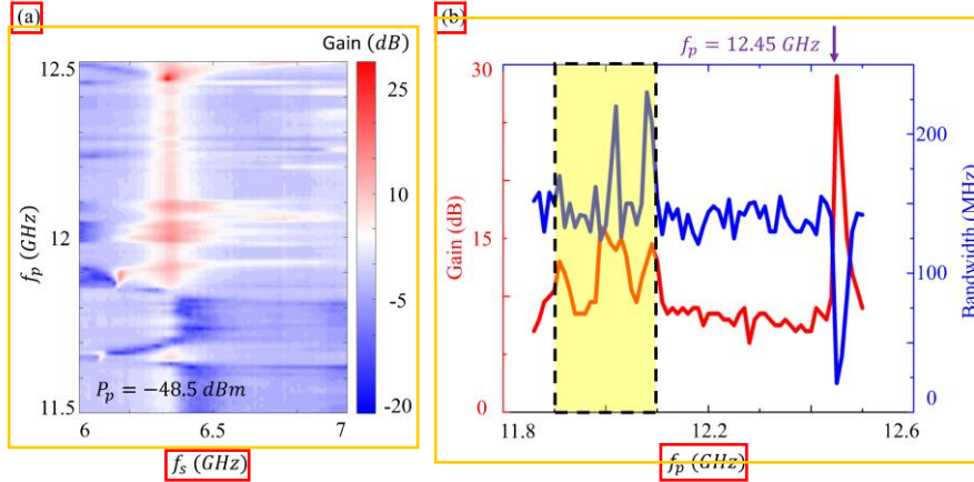
图 3.5.8 (a) f_{J-Amp} \approx 6.23 \text{ GHz} 时放大器在 flux-pump 模式下的增益性质。我们设定到样品的 pump 功率为 P_p = -48.5 \text{ dBm} ，然后在 11.5\text{--}12.5 \text{ GHz} 范围内扫描 f_p (b) 从 (a) 图中提取出的增益/增益带宽随 f_p 的变化关系，我们发现，在标黄区域内，当 f_p \sim 11.9 - 12.1 \text{ GHz} 时，放大器的增益以及增益带宽得到了同时增强，除此以外， f_p = 12.45 \text{ GHz} \approx 2f_{J-Amp} 时，具有尖峰增益同时增益带宽锐减。
