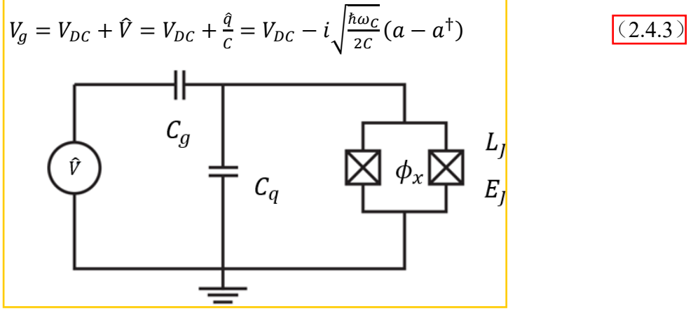
图 2.4.2 Transmon 与 CPW 耦合的等效电路示意图。
