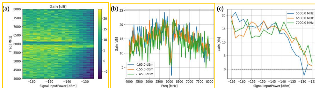
图 3.5.1 (a) J-TWPA 的增益数据，横轴为信号功率，纵轴为信号频率； (b) 在 (a) 图中截取的信号功率分别取 -165 dBm/-155 dBm/-145 dBm 的三条数据； (c) 利用 (a) 图，在三个不同的信号频率处增大信号功率所得到的增益曲线，从曲线中估算出增益饱和功率大约是 -140 dBm 左右。在此要感谢浙江大学王腾辉博士以及张贞兴博士在测量数据上提供的帮助。
