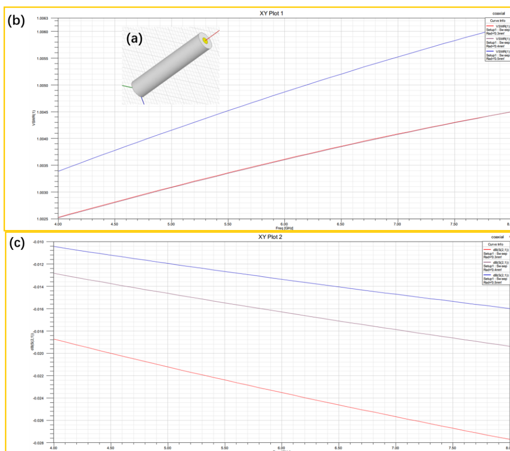
图 3.6.2 (a) 弹簧针与聚四氟乙烯套组合的 HFSS 模型，内层黄色为弹簧针；(b) 和 (c) 分别为在不同聚四氟乙烯套外径下的端口电压驻波比以及插入损耗仿真数据。红色，暗红色，蓝色曲线分别为聚四氟乙烯套外半径 0.3mm、0.4mm、0.5mm 对应的仿真结果。
