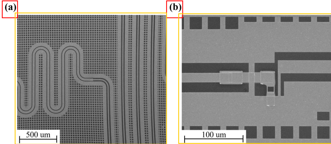
图 3.5.2 J-IMP 的 SEM 电镜照片。其中 (a) 是阻抗变换线结构, 由于第一段为信号引入段, 因此没有给出, 图中的结构从左到右分别为四分之一波长传输线以及二分之一波长传输线; (b) J-Amp 结构, 其中电容结构为 Al-AlO x -Al 平行板电容器, AlO x 氧化层为第一层铝膜在纯氧干燥腔体中原位氧化 12h 制备出来。
