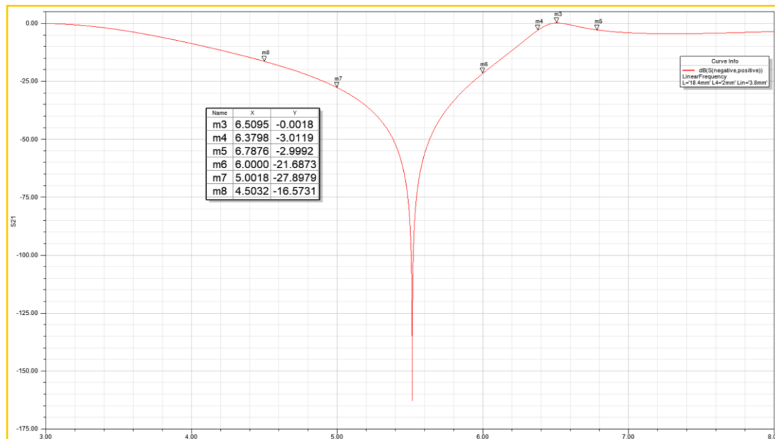
图 3.4.4 在 L_{in} = L_{out} = 3.8 \text{ mm} 的参数条件下，半波长谐振腔 Purcell filter 的 HFSS |S_{21}| 仿真结果。
