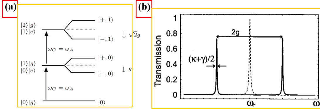
图 2.1.2 (a) \Delta = 0 时 J-C 模型对应的能级简图；(b) 满足公式 (2.1.16) 时 dressed 态原子与真空光子相互作用时的能级频谱分布，引用自[3]。
