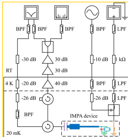
图 3.5.4 flux-pump 工作模式下 J-IMPAs 的测试电路。
