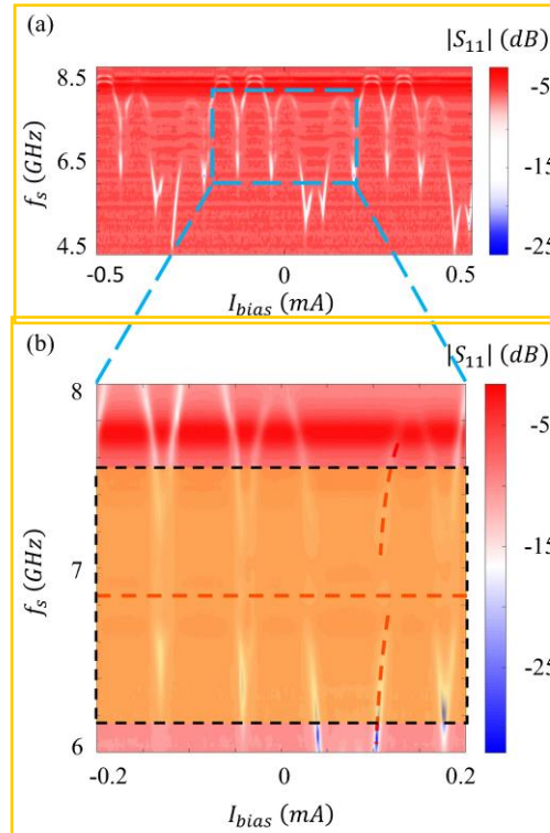
图 3.5.5 (a) 当 P_s = -120 dBm 时 J-IMPA 的磁通调制性质；(b) 图 (a) 中蓝色虚线框内区域的细扫。
