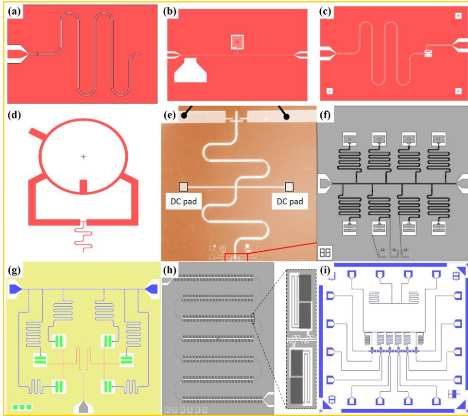
图 2.3.3 (a) 一种 \lambda/4 反射腔设计图；(b) 一种 \lambda/2 透射腔设计图；(c) 一种 \lambda/4 反射腔式 JPA 设计图；(d) 一种引入了 180^\circ 反向环的差分带线反射腔设计图；(e) 一种差分带线反射腔的光显照片，该结构用于研究和两个石墨烯双量子点的耦合[26] [27]；(f) 一种 8-qubit 测试芯片设计图；(g) 一种引入了多终端可调量子数据总线的 6-qubit 测试芯片设计图；(h) 一种以约瑟夫森结链改造的传输线式行波参量放大器 (J-TWPA) 的设计图；(i) 一种引入传输线信号供线的 6-qubit 测试芯片设计图。
