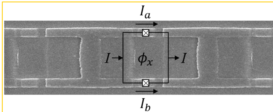
图 2.2.3 一种 SQUID 链状结构的 SEM 照片。
