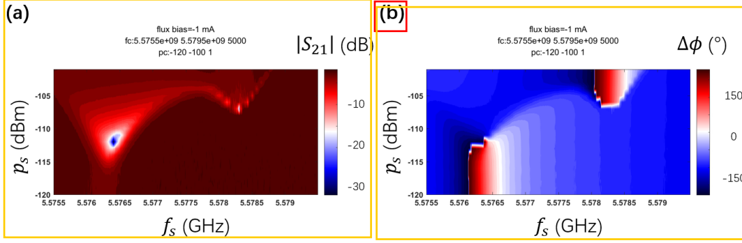
图 5.1.1 使用网络分析仪获取的读取腔散射矩阵的 (a) 幅值 (b) 相位响应随信号功率的变化。
