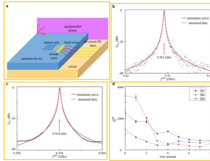
图 3.8.4 (a) 引入直流调控的 3D 微波谐振腔结构模型示意图。(b) 不引入直流电极以及 wire-bonding 的 TE101 室温模式测量与仿真结果。(c) 引入 8 根直流电极后的 TE101 室温模式测量与仿真结果。(d) 引入 wire-bonding 后, bonding 数量与 3D 腔的 TE101、TE102、TE103 模式品质因子的室温测量结果。可见随着 wire-bonding 数量的增加, 3D 腔的 Q 值会急剧下降, 因而我们最多只能引入 8 根直流电极。
