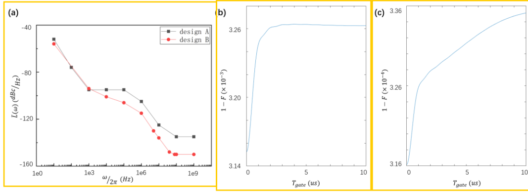
图 5.3.2 (a) 两种测控系统设计方案对应的 LO 相噪以及他们分别对操作保真度的影响， (b) design A； (c) design B，它产生的固有非保真度只有 design A 的十分之一。
