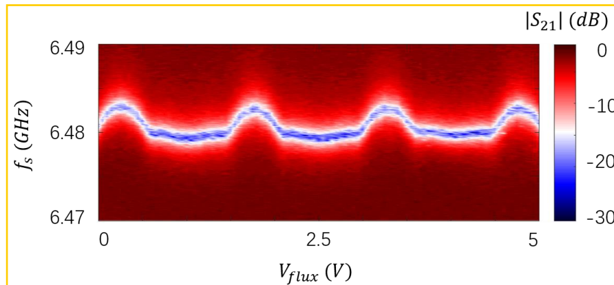
图 5.1.2 设定 P_s = -120 \text{ dBm} ，使用网络分析仪获取的读取腔随着 V_{flux} 的周期性变化。
