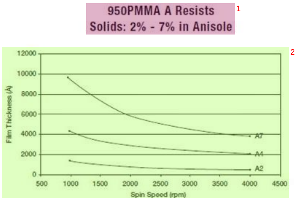
图 2.4 950PMMA A 系列电子束曝光胶厚度随匀胶转速的变化曲线
