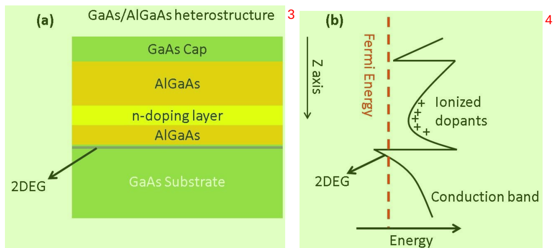
图 1.1 (a) 掺杂型 GaAs/AlGaAs 基片的异质结构。利用分子束外延 (MBE) 的方法, 5 依次生长纯 GaAs 基底、AlGaAs 缓冲层、n-type AlGaAs 层、AlGaAs 隔离层和表面的 GaAs 盖帽层。其中, AlGaAs 中 Al 的质量分数为 30%, 掺杂原子为 Si 原子, 掺杂浓度为 5-11 \times 10^{17}/\text{cm}^3 。图 1.1 (b) 为沿垂直基片方向半导体的能带图。由于 AlGaAs 掺杂层的存在, 会在异质结中间形成内建电场, 使得 GaAs 基底靠近 AlGaAs 层位置的导带弯曲到费米面以下, 形成二维电子气 15 。
