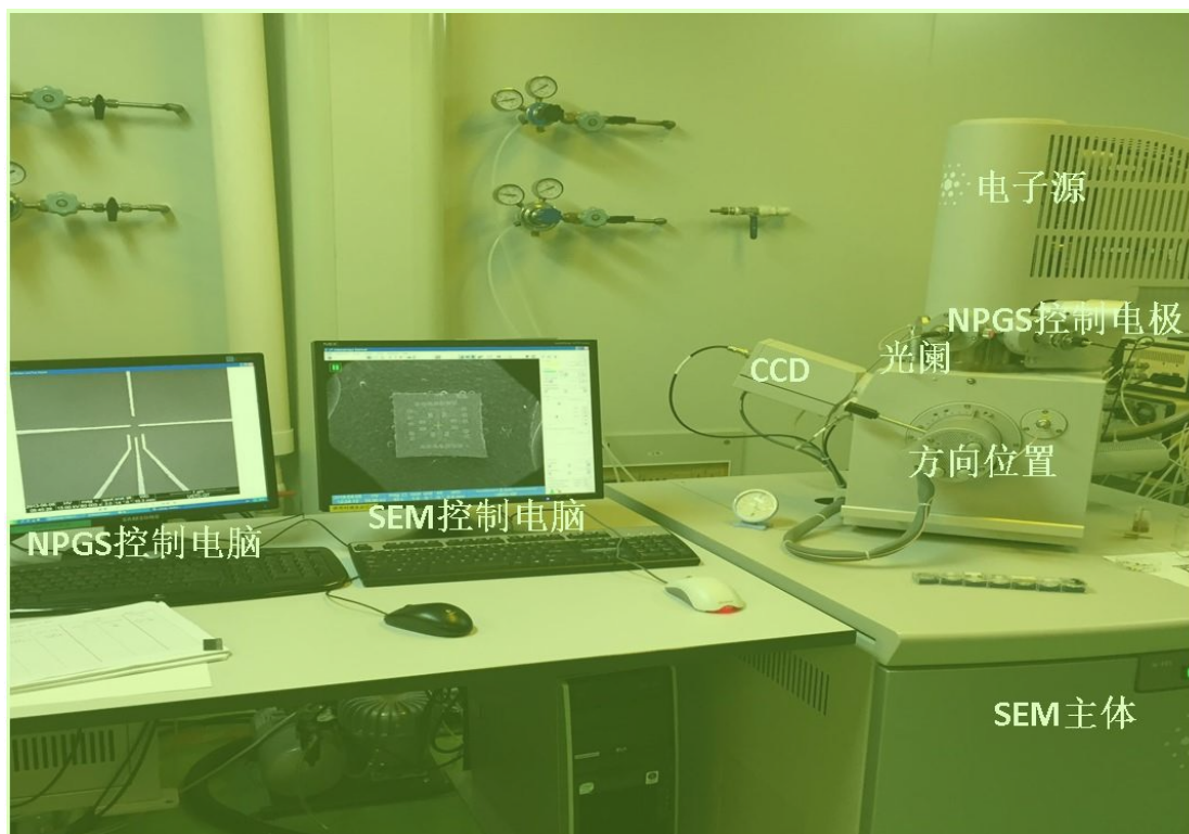
图 2.3 我们实验小组使用的 SEM 及 NPGS 控制系统。主要包括：场发射电子源及电学 5 透镜系统；SEM 光阑；CCD 探头；NPGS 控制电极；样品台方向位置调节；SEM 控制电脑；NPGS 控制电脑；SEM 机柜。
