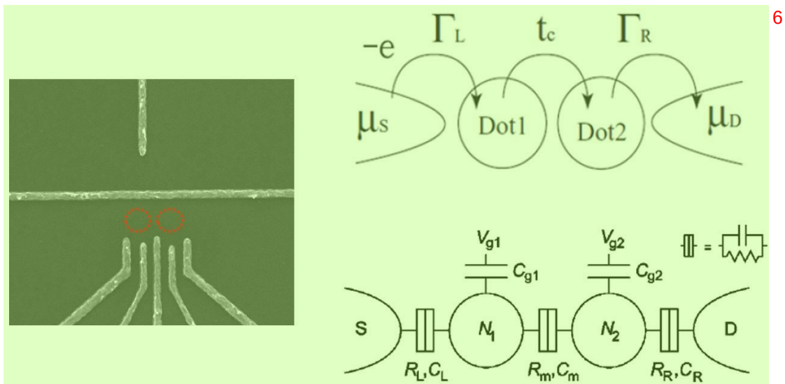
7 图 3.1 (a) 常见串联 DQD 的 SEM 图，红色圆圈表示两个量子点形成位置。(b) 串联
