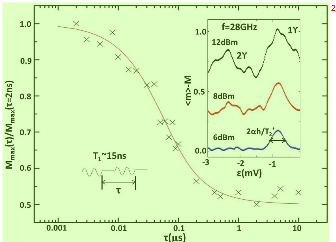
图 6.4 一阶 PAT 共振峰的相对高度随斩波周期 \tau 的变化曲线。实线表示最佳拟合曲线， T_1\approx 15\text{ns} 。插图：当微波频率 f=28\text{GHz} 时，三种不同功率下的共振峰情况。为了三条曲线的清晰分辨，上面两条曲线分别有 0.3 和 0.6 的纵轴偏置。随着微波功率的增加，一阶共振峰达到饱和，高阶共振峰开始出现。黑色箭头表示饱和一阶共振峰的半高全宽 (FWHM)，用于估计二能级体系的退相干时间 T_2^* 。
