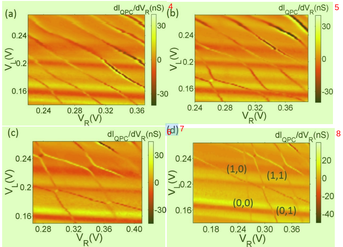
图 5.5 不同中间电极电压 V_{\text{T}} 下, QPC 微分电流信号随电极 V_{\text{L}} 、 V_{\text{R}} 变化的电流相图。 9
