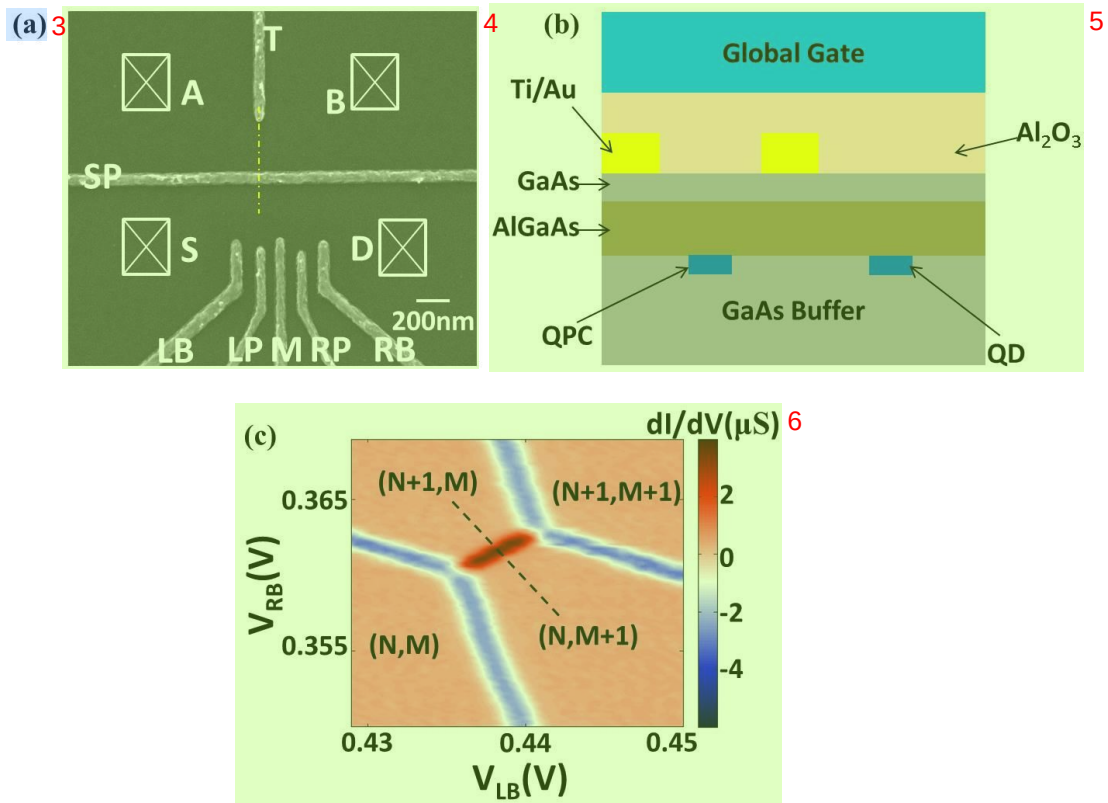
图 6.1 (a) 这次实验所使用双量子点器件的 SEM 图片。下面的五个电极限制出双量子点, T 电极用来调节 QPC 通道的电导, SP 电极用来隔离量子点与 QPC 通道。白色方框 A,B,S,D 表示欧姆电极, 与 2DEG 直接相连。(b) 非掺杂双量子点器件横截面图, 这次实验顶部电极电压 V_T=2.9\text{V} 。(c) QPC 微分电导 dI/dV 随门电极电压 V_{LB} 和 V_{RB} 的变化相图。沿着黑色虚线方向, 电子态从 (N+1, M) 到 (N, M+1) 发生转变。
