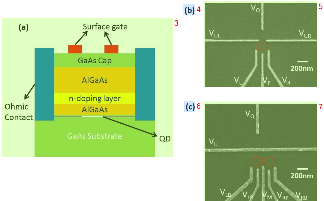
图 1.3 (a) 传统掺杂 GaAs 量子点的纵向横截面。(b) 和 (c) 分别表示常见的单点和双点的内部纳米电极结构 SEM 图片，下方是量子点输运通道，上方 QPC 通道为电荷探测器来感应量子点中的电荷态。
