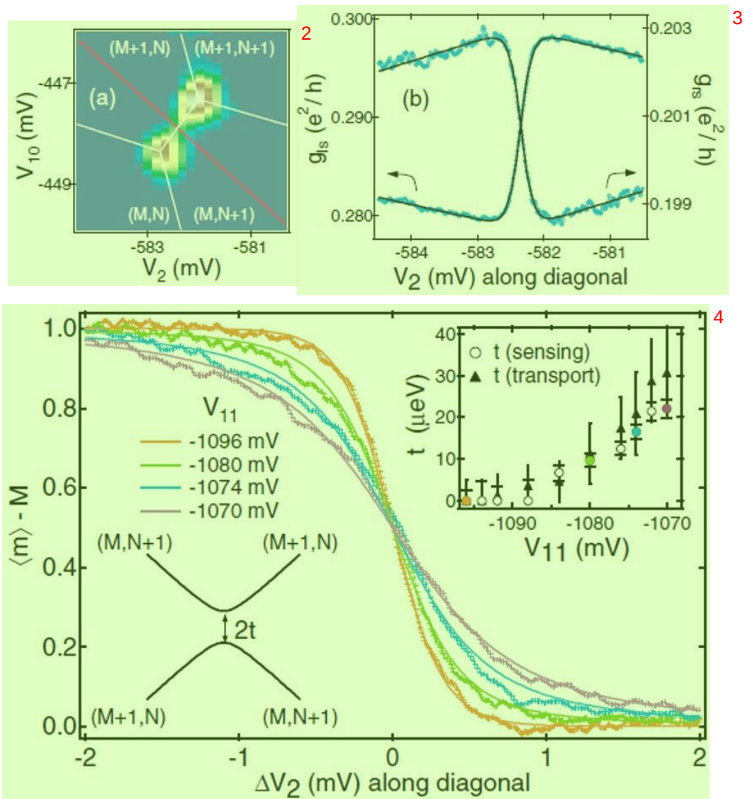
图 3.6 (a) 在三相点附近的细扫电流相图，红色线表示保持双量子点中总电荷数目不变的扫描方向。(b) 沿着 detuning 方向，两边 QPC 电导与栅极电压 V_2 的变化曲线。(c) 改变 V_{11} 电压，沿 detuning 方向得到台阶宽度的变化。右上插图表示耦合强度随着门电极电压
