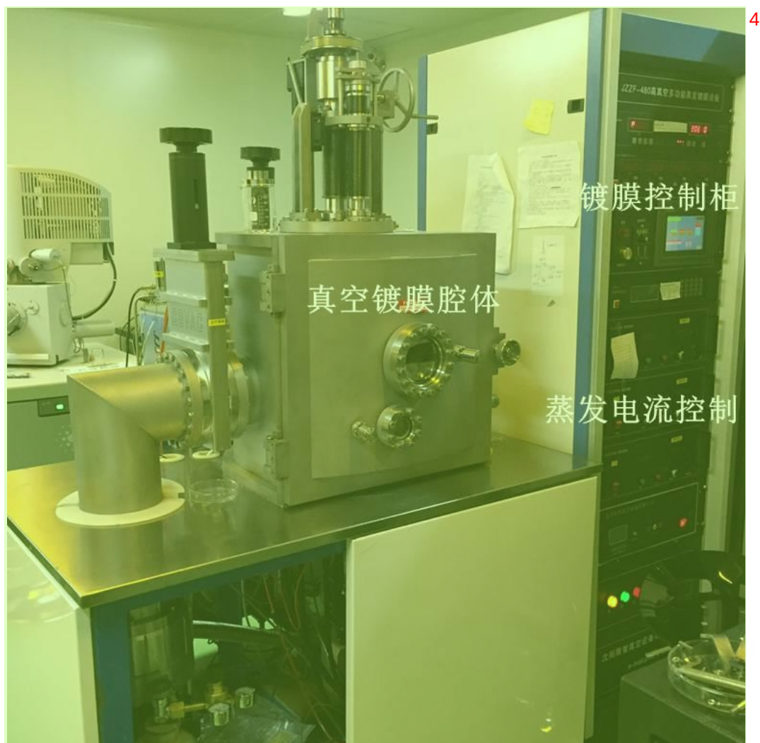
图 2.6 国产热蒸发镀膜机。
