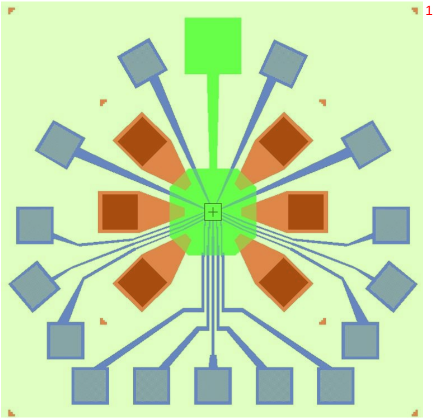
图 5.2 非掺杂砷化镓量子点整体示意图，中心十字为纳米小电极区域。 2
