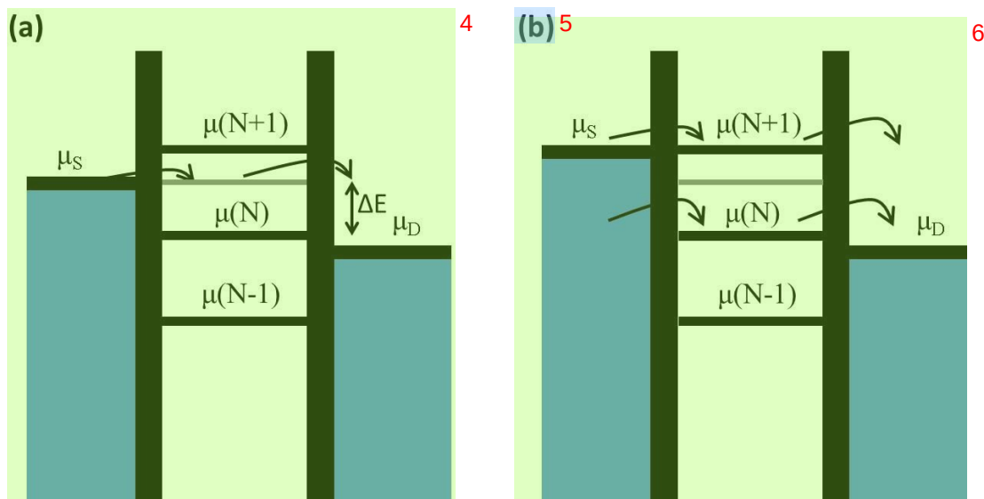
图 1.6 增大偏压窗口解除库仑阻塞。(a) 第 N 个电子的激发态化学势进入偏压窗口, 电子可以任意选择通道完成输运, 电流发生变化。(b) N+1 电子基态化学势进入偏压窗口, 电流剧增。
