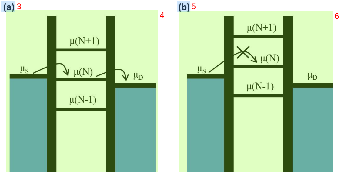
图 1.4 (a) V_{SD} 较小，第 N 个电子能级进入源漏偏压窗口，完成电子输运。(b) V_{SD} 较小，没有电子能级处在源漏窗口内，这时电子无法通过量子点完成输运，形成库仑阻塞。
