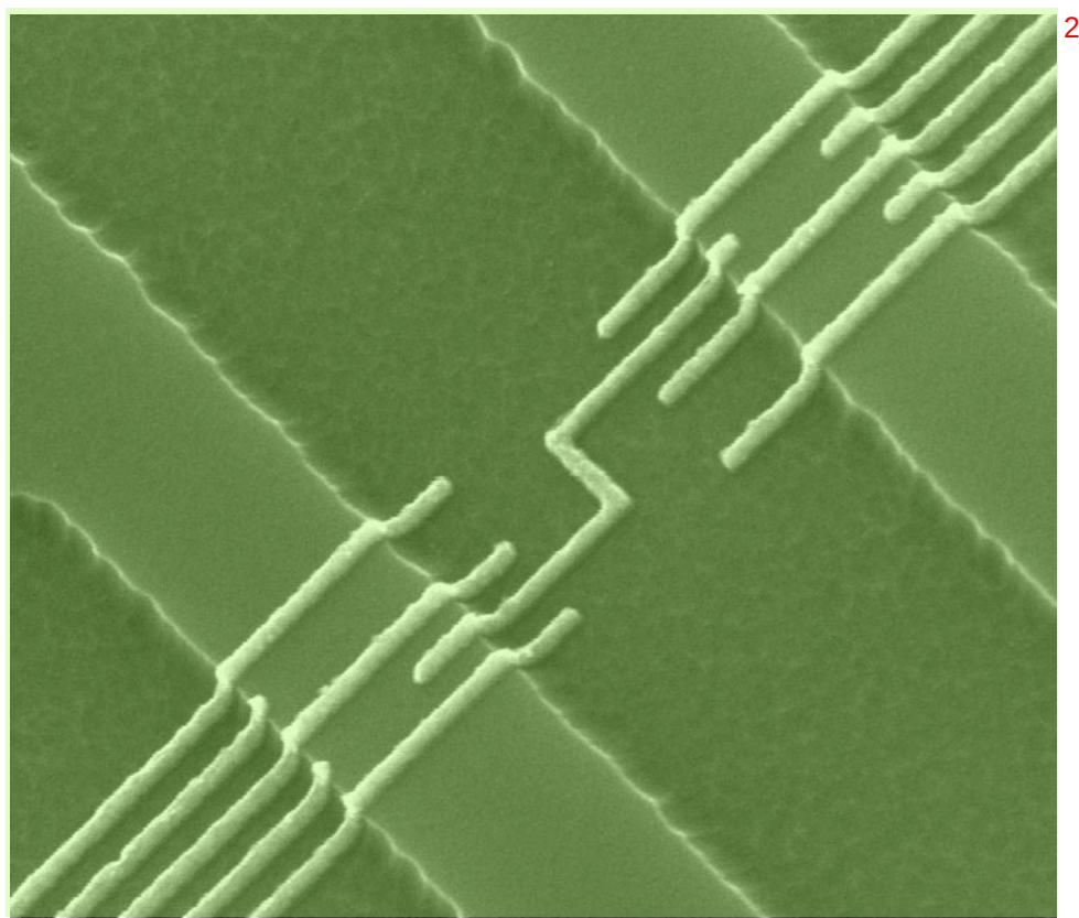
图 4.2 制备完成的浅刻蚀砷化镓量子点的 SEM 图(扫描角度与基片垂直方向夹角 30^\circ )。 3
