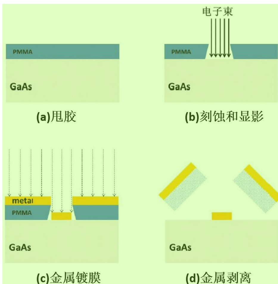
图 2.7 EBL 及金属 lift-off 工艺过程示意图。 3
