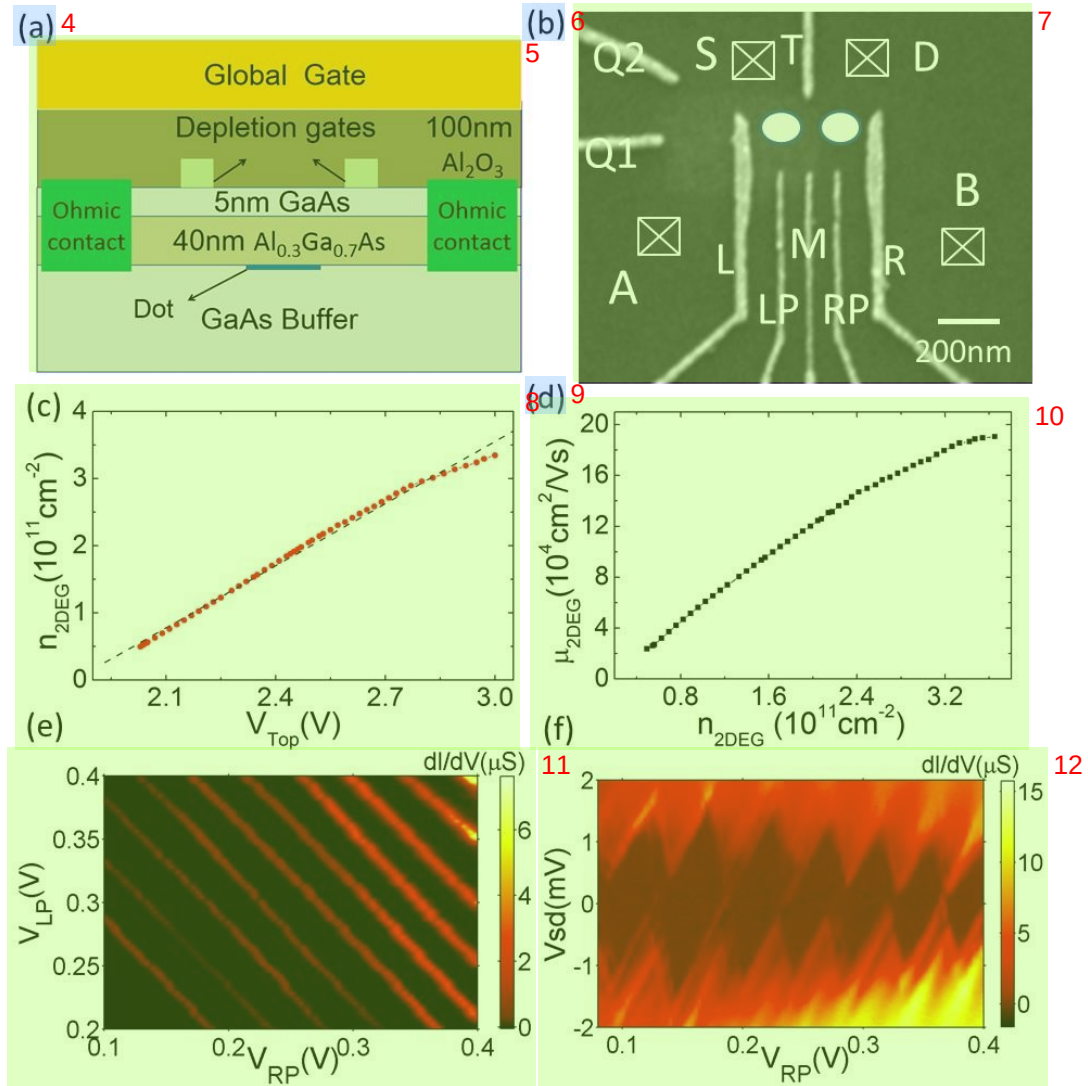
图 5.4 (a) 双量子点器件的横截面图。(b) 双量子点器件内部纳米电极的 SEM 图片。 13
