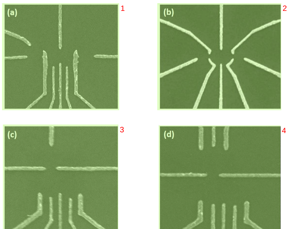
图 7.1 各种结构空穴型双量子点器件 SEM 图 5
