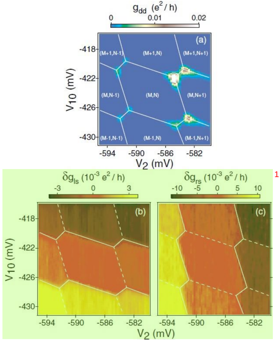
图 3.5 串联双量子点测量相图。(a) 双量子点通道输运信号相图。(b) (c) 使用左右两个 QPC 通道输运信号探测量子点状态得到的相图。图片引自文献 5 。
