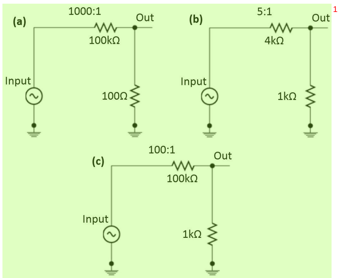
图 2.17 我们实验室三种常用分压盒子内部电路示意图 2
