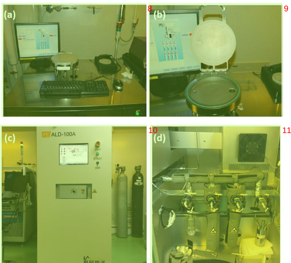
图 2.9 (a) 和 (b) 我们常用的热型 ALD 设备。(c) 和 (d) 是国内自己研发的热型和等离子体增强型双功能 ALD 设备。
