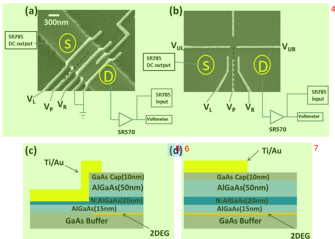
图 4.2 制备完成的浅刻蚀砷化镓量子点的 SEM 图(扫描角度与基片垂直方向夹角 30^\circ )。 3
