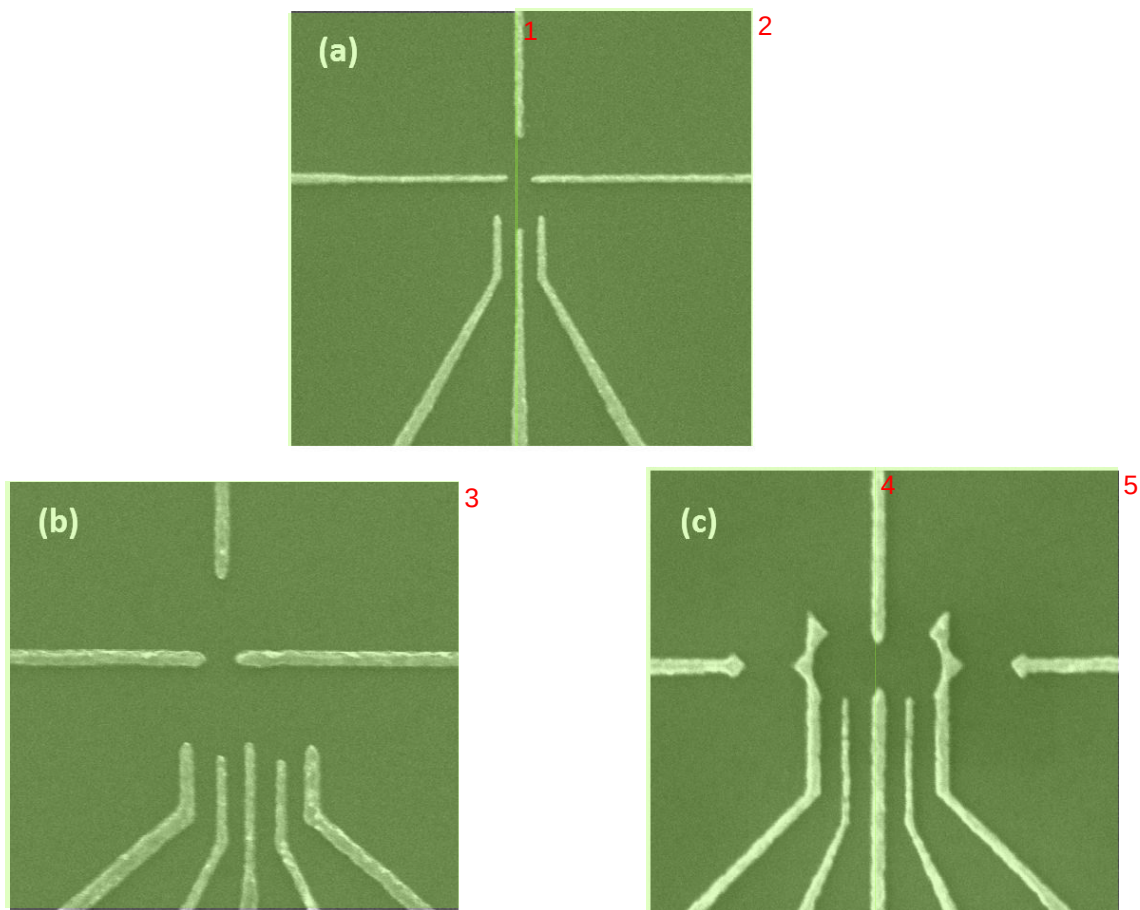
图 2.14 (a) 常见单量子点结构。(b) 顶部 QPC 双量子点结构。(c) 侧面双 QPC 双量子点结构。
