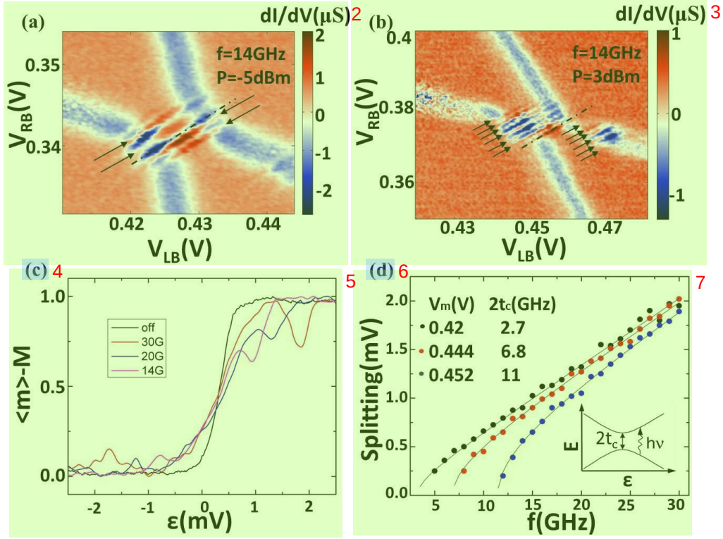
图 6.3 (a) 微分电导随 V_{LB} 和 V_{RB} 的变化相图。此时 V_m=0.42\text{V} ，微波频率 14\text{GHz} ，功率 -5\text{dBm} 。黑色虚线表示电荷跃迁线中心位置，在图中可以观察到两阶光子辅助隧穿过程。 8 (b) 微分电导随 V_{LB} 和 V_{RB} 的变化相图。此时 V_m=0.42\text{V} ，微波频率 14\text{GHz} ，功率 3\text{dBm} 。可以看到六阶光子辅助隧穿过程，因为微波功率的增加，相图整体信号变弱。 (c) 在三种不同频率微波驱动下，左边量子点的平均电荷增加数随失谐量的变化曲线。 4 (d) 三种不同门电极电压 V_m 下，共振峰劈裂距离随驱动微波频率的变化曲线。实线为测量数据的拟合曲线，左上的表格为拟合出来的耦合能 2t_c 数据。 5 插图表示双量子点中的二能级体系及 PAT 过程示意图。 6
