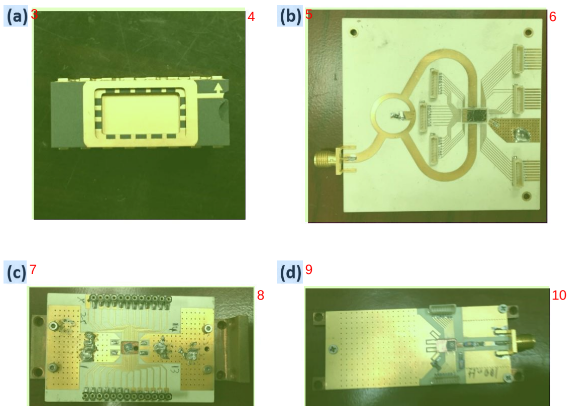
图 2.15 我们实验室常用的几种样品底座。(a) 主要用于粗测杆和 He3 制冷机。(b) (c) (d) 用于我们的无液氦稀释制冷机。
