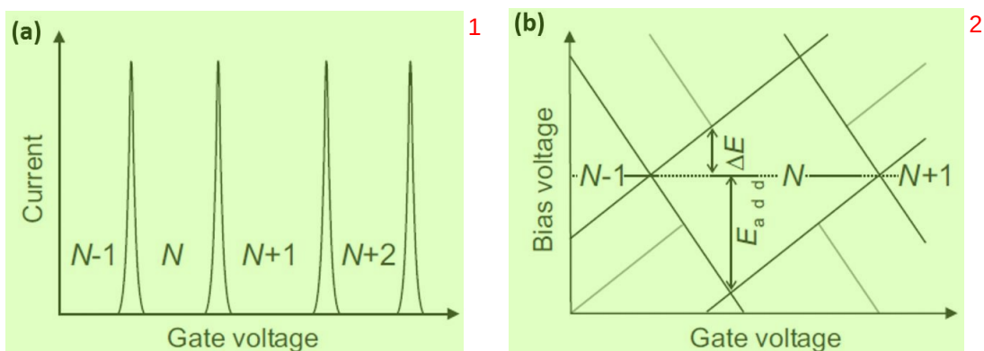
图 1.5 (a) V_{SD}=0 时, 量子点通道电流的周期性库仑峰。(b) 微分电导随着直流偏置电压和栅极电压变化的理论相图, 菱形内部没有隧穿电流, 菱形外部浅色实线说明出现了电子激发态。
