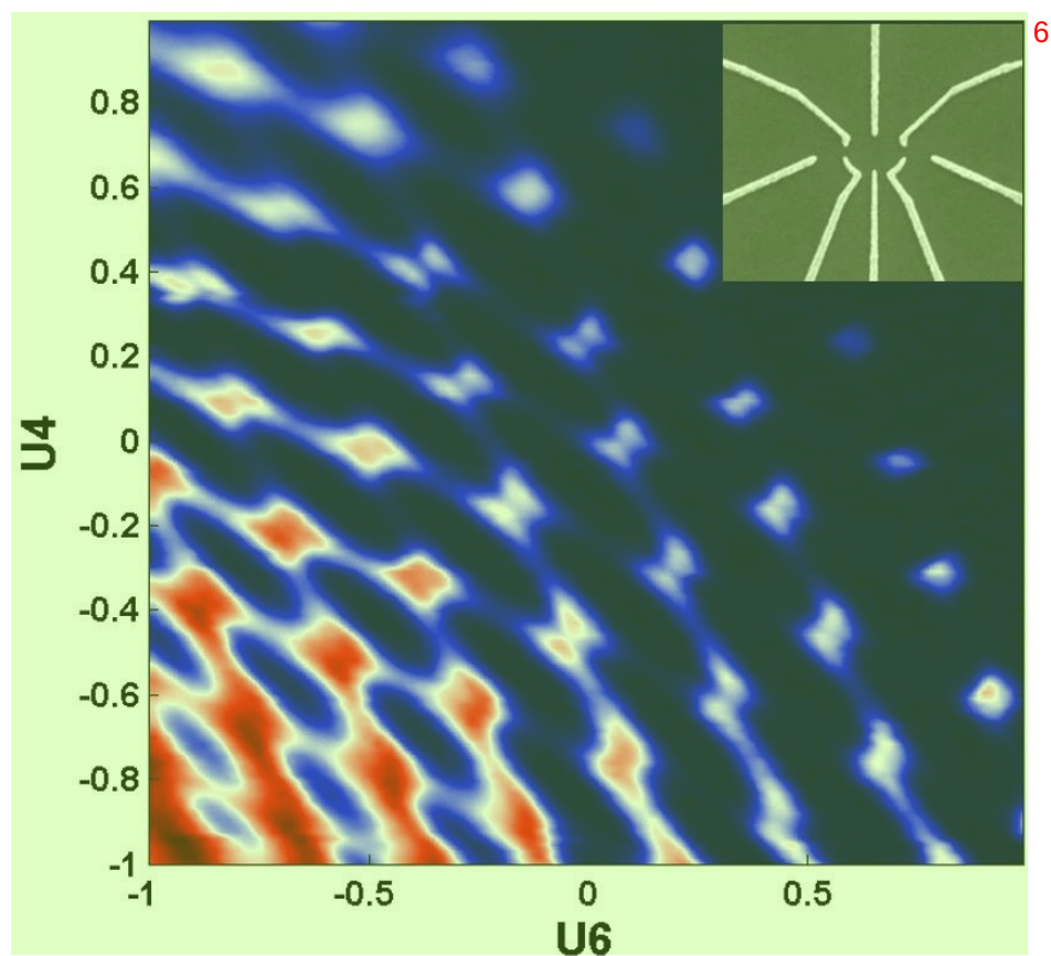
图 7.2 空穴型双量子点测量得到的电流稳定相图（右上为内部纳米电极 SEM 图片）。7
