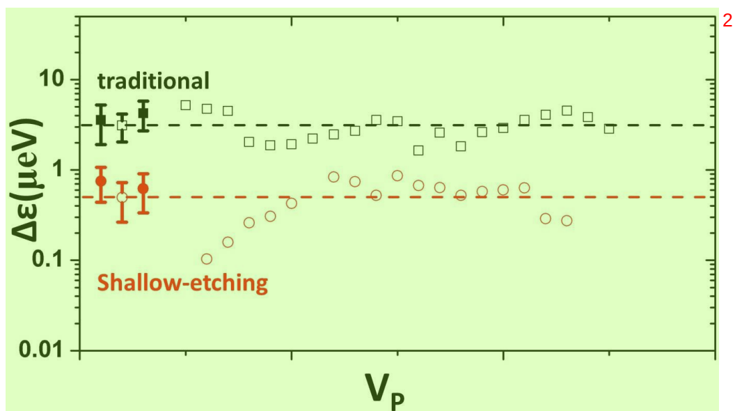
图 4.6 能量涨落与电极电压 V_p 的关系（在同一基片上制备、在同一测量系统测量的浅刻蚀量子点和传统量子点）。右侧的空心点表示沿着一个库仑峰得到的能量涨落数据，为了方便对比，我们将所有的数据点都转换到相同的 x 轴上。左边的黑色空心方块表示传统量子点的统计平均值 3.1 \pm 1.1 \mu\text{eV} ，红色空心圆圈表示浅刻蚀量子点上得到的统计平均数据 0.50 \pm 0.23 \mu\text{eV} 。实心的数据是我们从其他浅刻蚀量子点和传统量子点的不同库仑峰上得到的数据。
