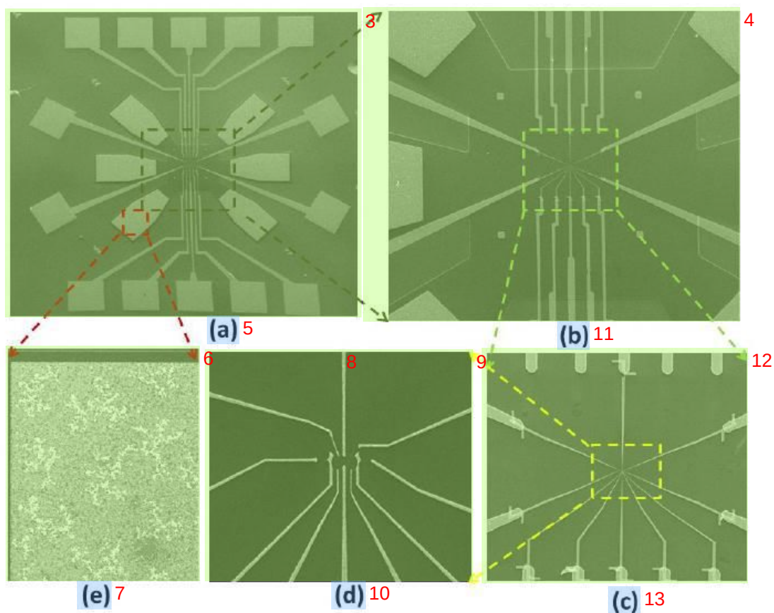
图 2.13 加工完成的传统 GaAs 双量子点的 SEM 照片。(a) 为量子点整体示意图。(b) (c) (d) (e) 为逐渐放大的量子点结构图。(d) 为 EBL 完成的纳米尺度的电极结构。
