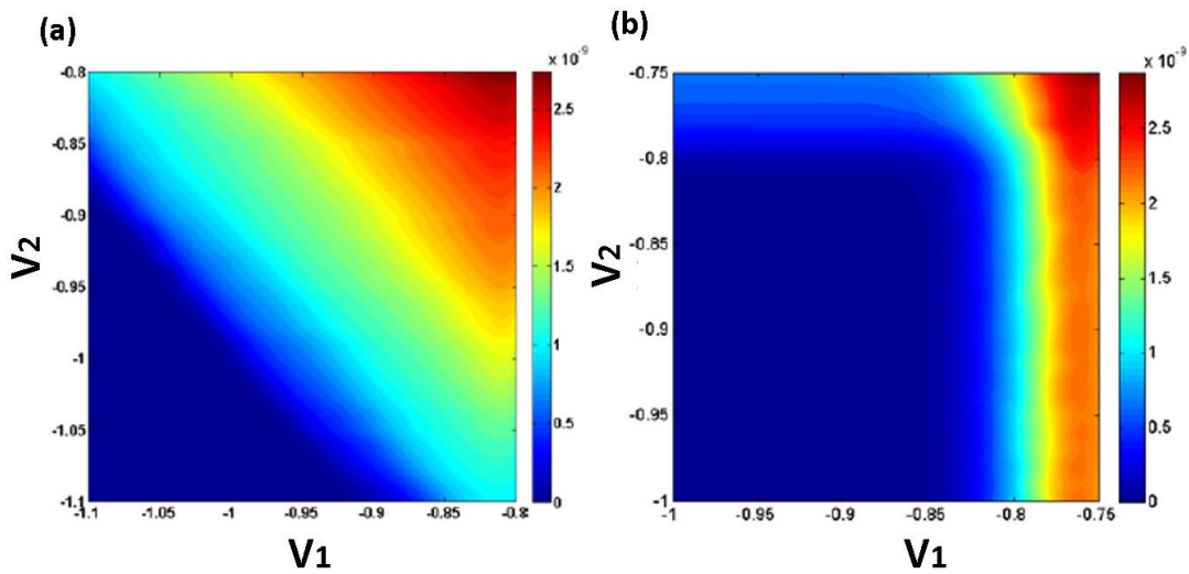
图 2.18 通道电导随门电极电压变化相图。(a) 出现平行的等电流线，说明两个门电极和电流通道耦合良好。(b) 等电流线出现直角情况，大部分区域的电导只由一个电极来控制，说明两个门电极和电流通道耦合不好，极低温下形成量子点可控性较差。
