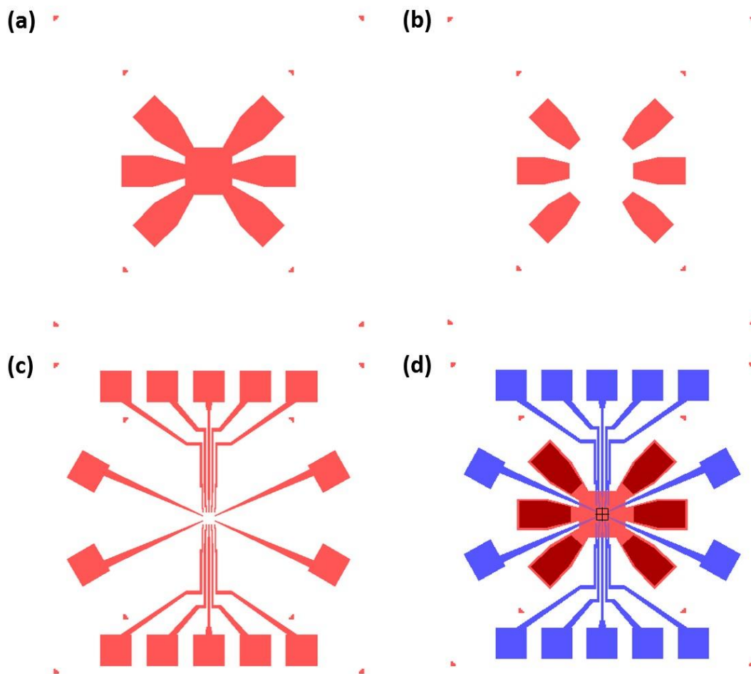
图 2.12 传统 GaAs 量子点制备使用的光刻板图案。(a) 二维电子气平台。(b) 欧姆接触电极。(c) 表面大电极。(d) 整体套刻效果图。
