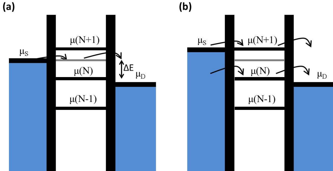
图 1.6 增大偏压窗口解除库仑阻塞。(a) 第 N 个电子的激发态化学势进入偏压窗口，电子可以任意选择通道完成输运，电流发生变化。(b) N+1 电子基态化学势进入偏压窗口，电流剧增。
