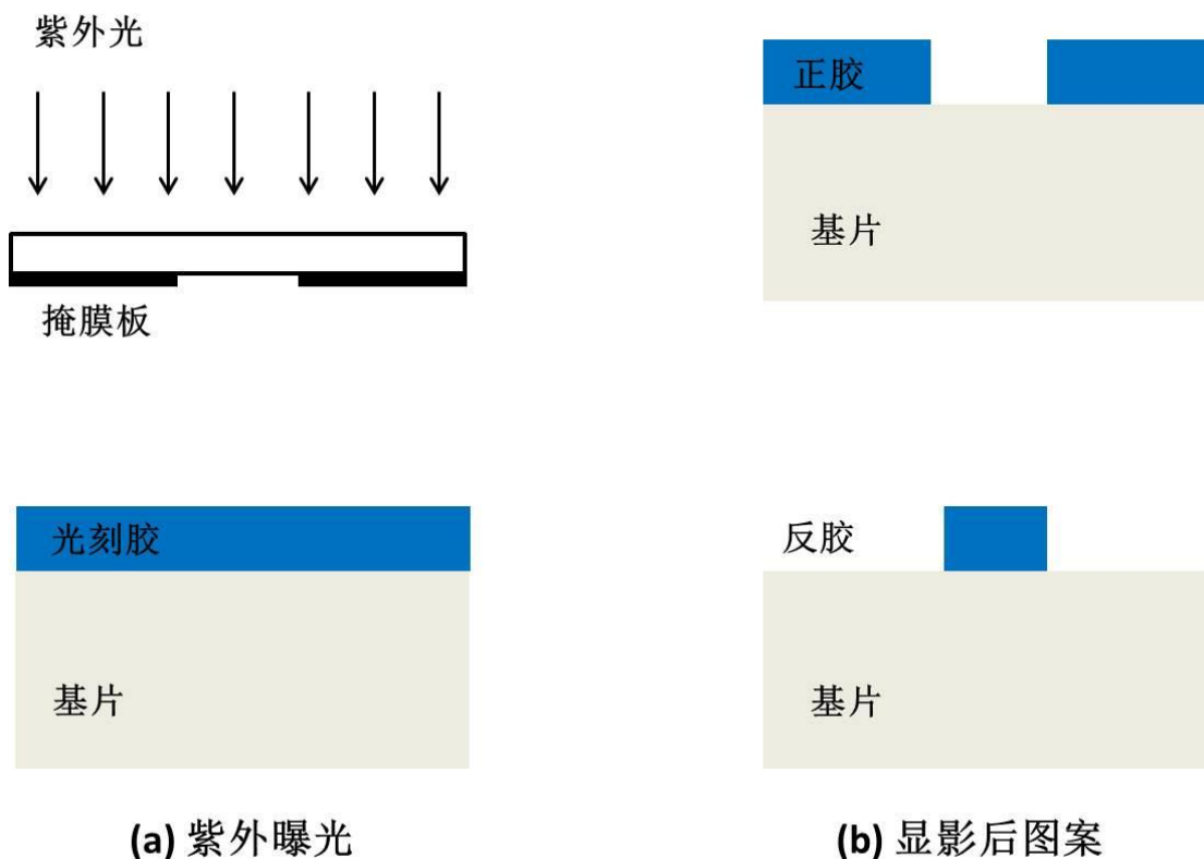
图 2.2 (a) 紫外曝光刻蚀。(b) 正、反胶显影之后胶的图案。
