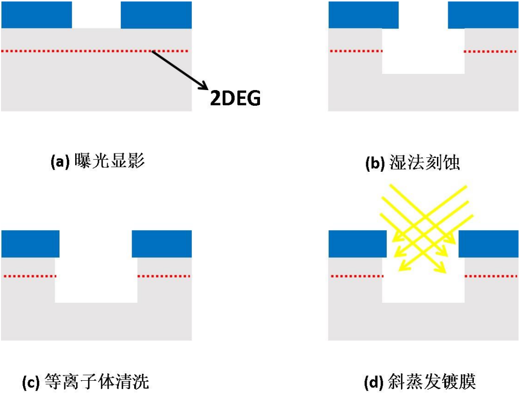
图 5.3 斜蒸发镀膜工艺流程示意图
