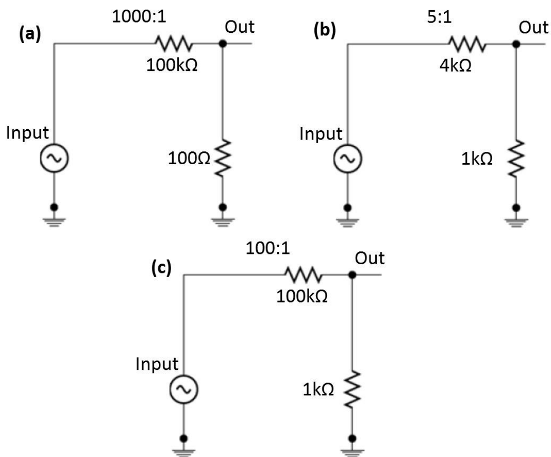
图 2.17 我们实验室三种常用分压盒子内部电路示意图
