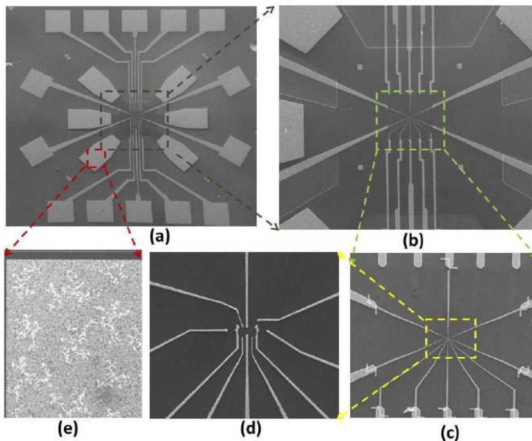
图 2.13 加工完成的传统 GaAs 双量子点的 SEM 照片。(a) 为量子点整体示意图。(b) (c) (d) (e) 为逐渐放大的量子点结构图。(d) 为 EBL 完成的纳米尺度的电极结构。
