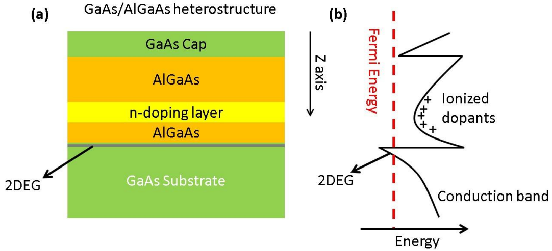
图 1.1 (a) 掺杂型 GaAs/AlGaAs 基片的异质结构。利用分子束外延 (MBE) 的方法,依次生长纯 GaAs 基底、AlGaAs 缓冲层、n-type AlGaAs 层、AlGaAs 隔离层和表面的 GaAs 盖帽层。其中, AlGaAs 中 Al 的质量分数为 30%, 掺杂原子为 Si 原子, 掺杂浓度为 5-11 \times 10^{17}/\text{cm}^3 。图 1.1 (b) 为沿垂直基片方向半导体的能带图。由于 AlGaAs 掺杂层的存在, 会在异质结中间形成内建电场, 使得 GaAs 基底靠近 AlGaAs 层位置的导带弯曲到费米面以下, 形成二维电子气 15 。
