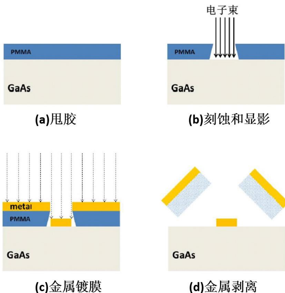
图 2.7 EBL 及金属 lift-off 工艺过程示意图。
