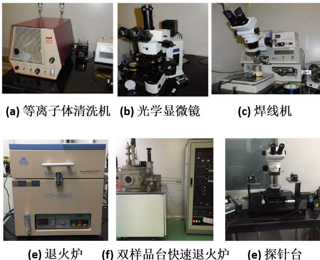
图 2.11 常用小型设备（二）。
