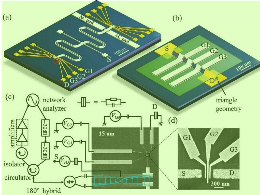
图5.1 (a) 量子点和谐振腔复合结构的三维示意图。谐振腔由两个超导传输线组成，并通过 AC板连接到微波的输入和输出端口。一个量子点位于红色矩形框区域。(b) 锗硅自组织纳米线量子点的结构三维示意图，由源漏电极和三个顶栅极以及一层绝缘层构成。图中可以看出锗硅自组织纳米线的三角形横截面。(c) 复合结构的直流输运测量和微波测量电路系统。两个超导传输线上的差分微波信号构建了稳定的电磁场。(d) 单量子点的扫描电子显微镜照片。
