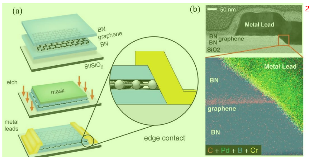
图 7.1 (a) 石墨烯和上下两层氮化硼的三明治结构的一维接触工艺。插图: 接触面的示意图。 (b) 透射电子显微镜图以及接触面的示意图。图片来自于[1]。
