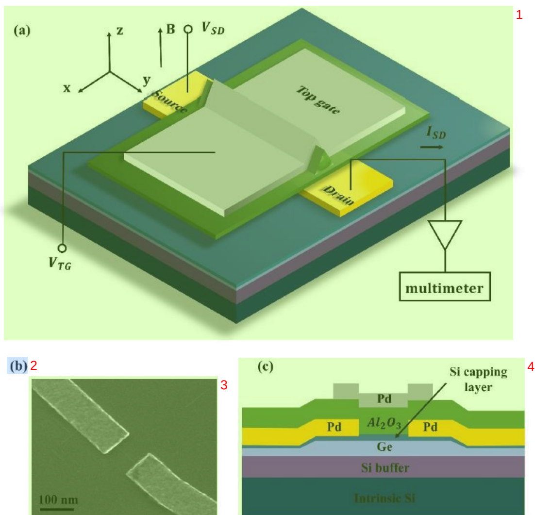
图 3.1 (a) 锗硅自组织纳米线的基片以及量子点的电极三维示意图。(b) 自组织纳米线和源漏电极的扫描电子显微镜照片。(c) 基片和量子点电极的横截面图。自下而上分别是本征硅，硅缓冲层，锗层和硅包覆层以及硅自然氧化层。
