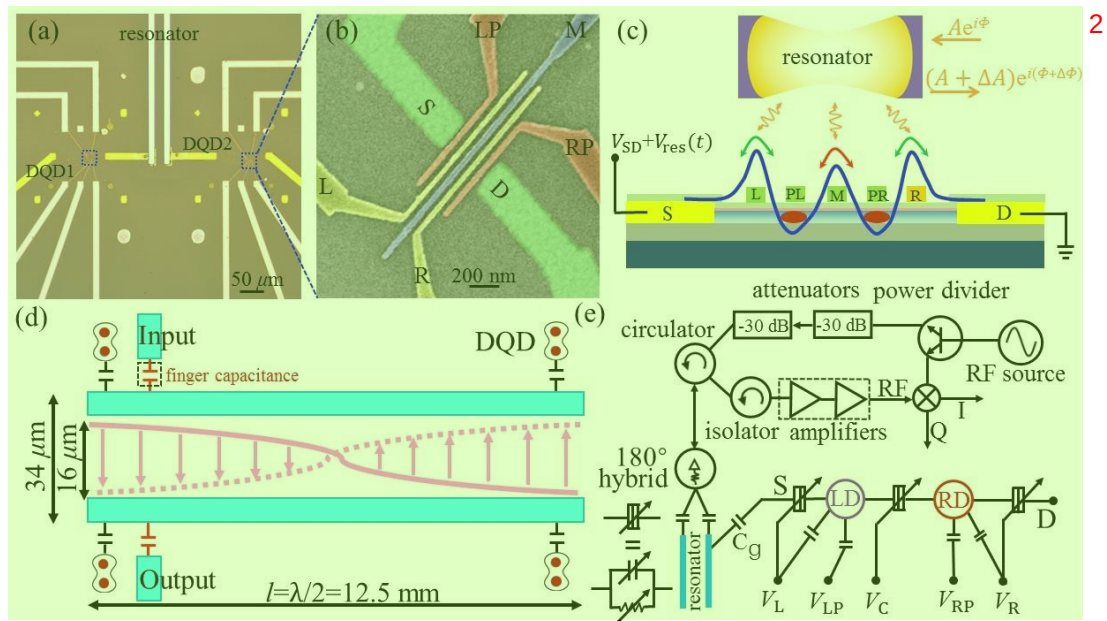
图 6.2 (a) 双量子点和谐振腔的复合结构的光学显微镜照片。双量子点通过源电极和谐振腔耦合到一起。(b-c) 双量子点的扫描电子显微镜照片和横截面示意图。扫描电子显微镜照片经过颜色处理, 其中绿色为源电极和漏电极, 红色为势垒电极、黄色为 plunger 电极、蓝色为中间电极。空穴在左点和右点之间隧穿或者量子点和电极之间隧穿都会影响到谐振腔的反射信号。(d) 谐振腔的设计结构图。腔的两根超导传输线通过指电容和微波的输入和输出端相连。施加在两根传输线上幅值相同、相位相反的微波信号构建了稳定的电磁场。(e) 双量子点的等效电路图以及复合结构的测量系统。
