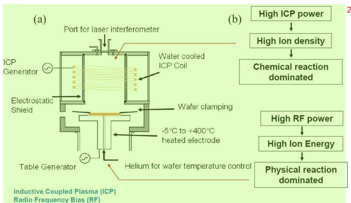
图 2.8 电感耦合刻蚀机结构示意图。(b) 刻蚀反应过程。图片来源于 Oxford 公司培训材料。3
