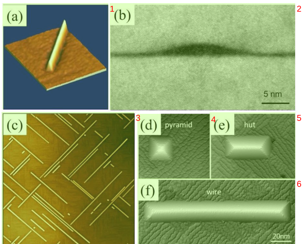
图 1.8 锗硅自组织纳米线的 (a) 原子力显微镜图 (b) 投射电子显微镜图片。(c) 纳米线沿 (100) 或者 (010) 方向生长。(d-f) 不同生长条件下得到的金字塔型锗硅纳米晶 (d)、棚顶型团簇 (e) 和棚顶型纳米线 (f)。图片引用自[65]。
