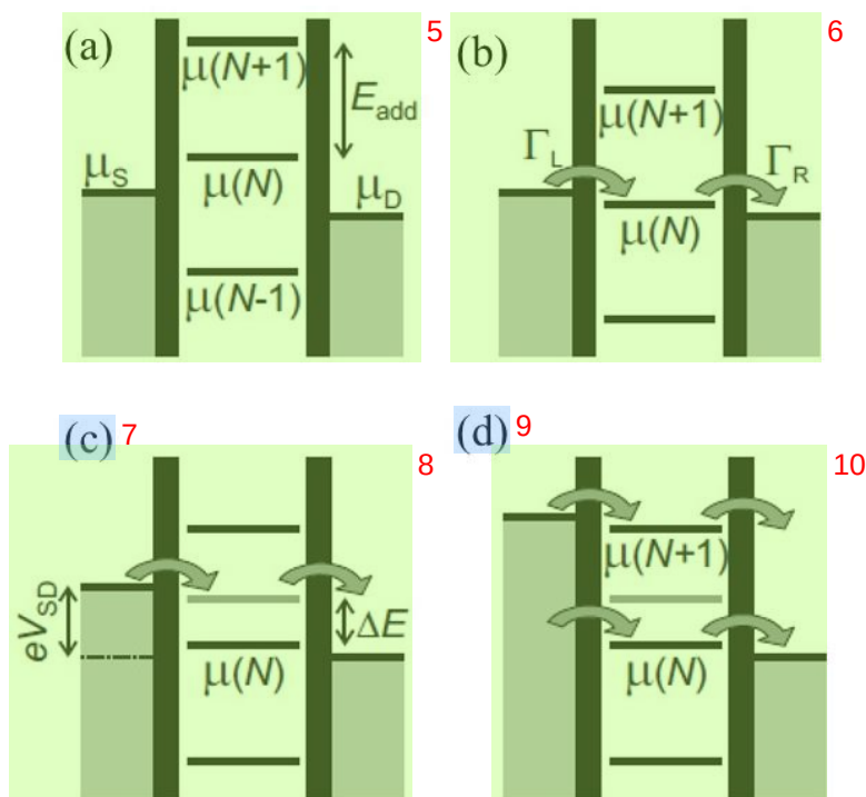
图 3.5 (a) 库仑阻塞区域，量子点中的任何一个化学势都没有落入偏压窗口之内，没有输运发生。(b) 库仑谐振区域，第 N 个空穴的化学势落入源漏偏压窗口中，发生输运发生。(c) 改变偏压窗口的大小，第 N 个空穴的基态和激发态都落入窗口内，空穴可以在两个路径之
