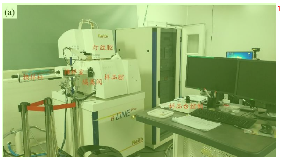
图 2.4 (a) E-line+E-line plus 模块，包括样品腔、灯丝腔、隔离阀、换样室、换样杆、样品台控制等组件。
