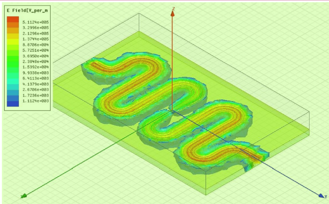
图 4.3 反射式超导微波谐振腔谐振器部分设计和仿真。利用 HFSS 软件对谐振器的电磁场模拟。可以看出电磁场主要集中在两根超导传输线之间。在波腹的位置电磁场的强度最大，在波结的位置电磁场强度几乎为零。
