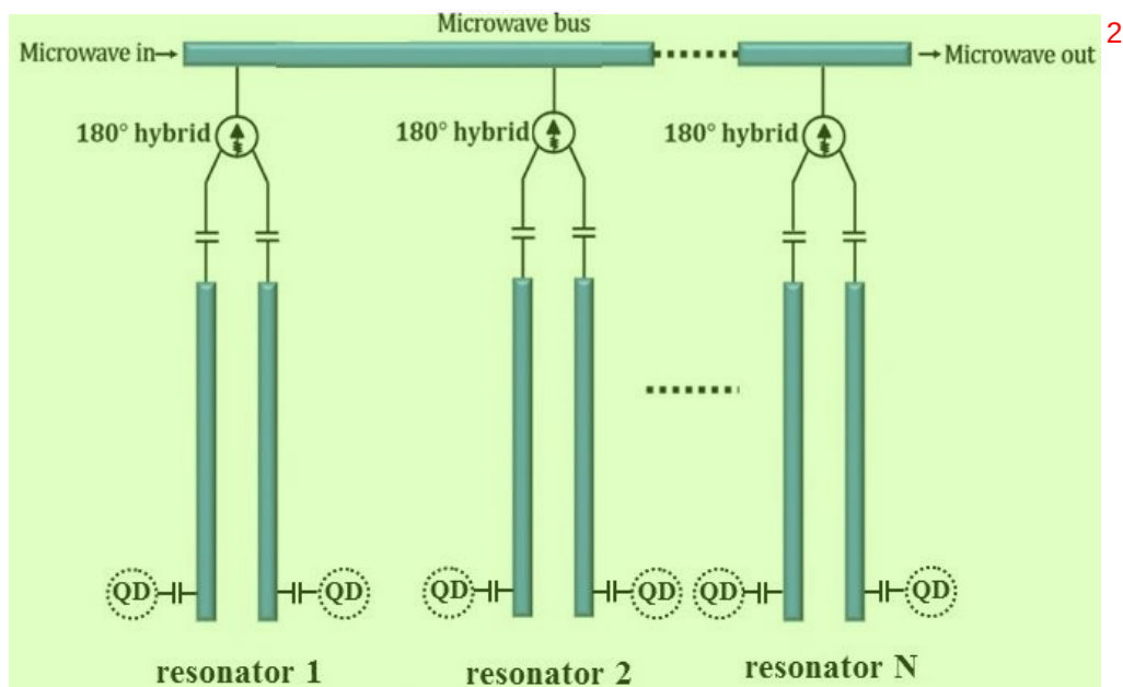
图 7.3 一个超导微波谐振腔作为将多个谐振腔串联在一起，每一个谐振腔作为量子总线耦 合到有限个量子比特。 3
