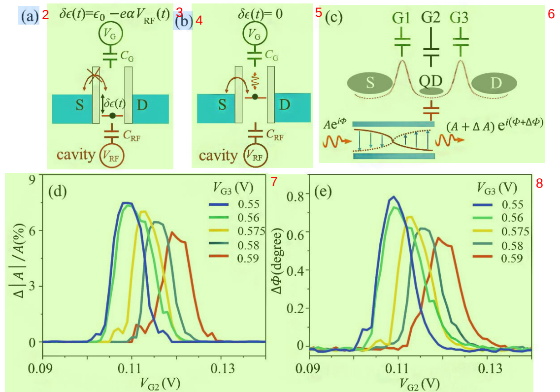
图5.4（a）谐振腔的传输线之间电磁场会在量子点的源漏偏置电压上产生电势震荡 V_{\text{RF}}(t) ，也随之影响量子点和源漏电极之间的电势能差 \delta\epsilon(t) = \epsilon_0 - e\alpha V_{\text{RF}}(t) 。（b）在库仑谐振区域， \delta\epsilon(t)=0 ，空穴在量子点和源电极/漏电极之间隧穿。（c）在固定 G_2 时，调节 G_1 和 G_3 会改变空穴的隧穿。谐振腔的幅值和相位信号对于隧穿率的变化有灵敏的反应。（d-e）调节势垒电极的电压 V_{G3} ，从而调节隧穿率时，对应的相位和幅值变化的库仑峰。
