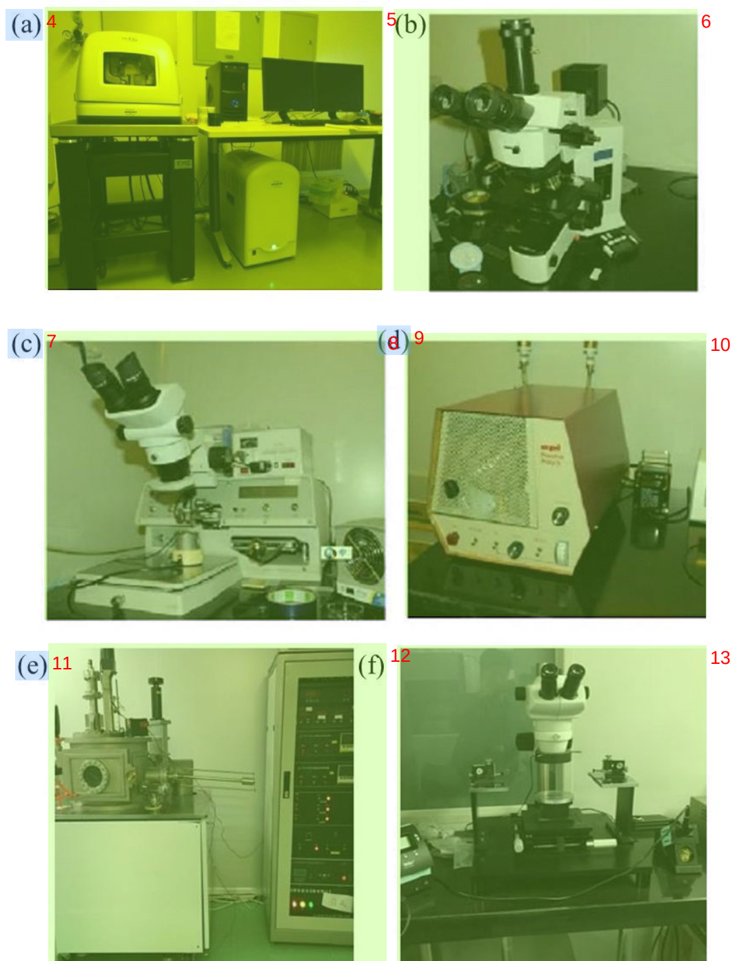
图 2.11 (a) 原子力显微镜。(b) 光学显微镜。(c) 键合机。(d) 等离子体清洗机。 14 (e) 退火炉。(f) 探针台。
