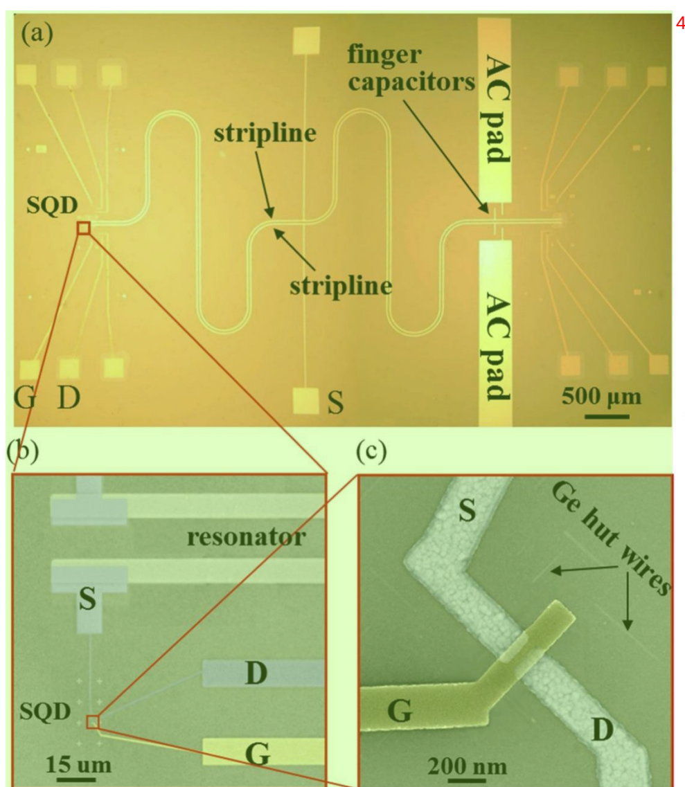
图 4.1 (a) 微波谐振腔和四个量子点的复合结构的光学显微镜照片。红色矩形是其中的一个 4 单量子点所在区域。(b) 量子点通过源电极与微波腔耦合的扫描电镜照片。(c) 单量子点结构的扫描电子显微镜照片。 5
