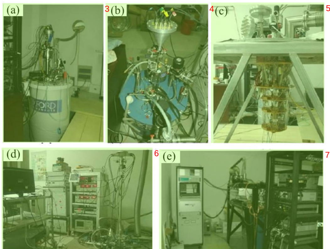
图 2.12 (a-b) 传统 He3 稀释制冷机。(c) 带自冷凝杜瓦 He3 稀释制冷机 (d) 插杆式稀释制冷机。(e) He3/He4 混合器稀释制冷机。
