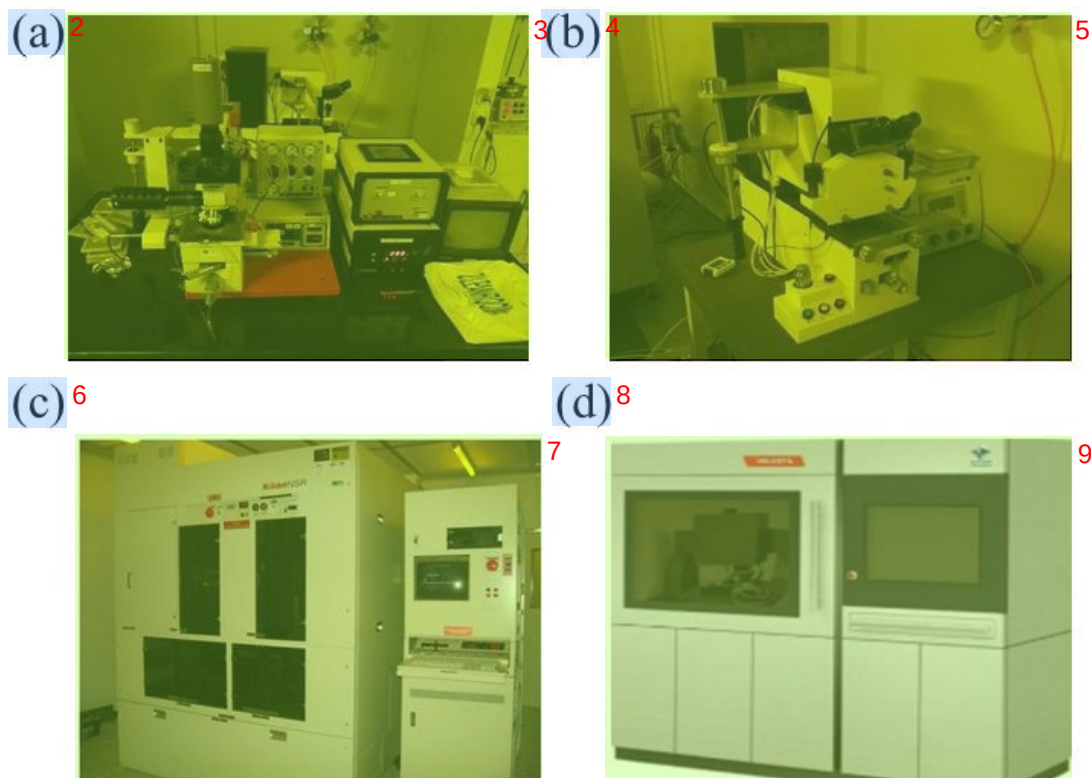
图 2.1 (a) SUSS 公司的接触式光刻机 MJB3。(b) 中国电子集团公司 45 所的接近式光刻 机 BG-401A。(c) 尼康公司的步进式光刻机 NSR i9。(d) Advantool 公司的 ATD 1500 激光 直写。
