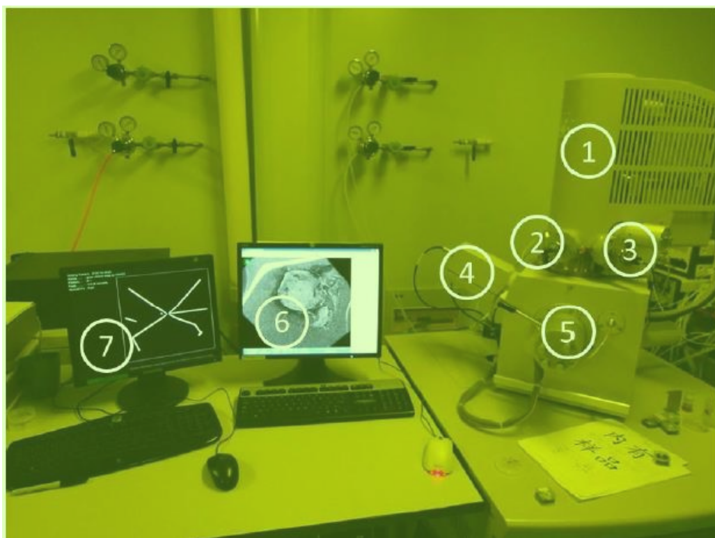
图 2.3 Inspect F50+NPGS 的构成。(1)高电压电子发射源；(2)光阑；(3)NPGS 控制系统； 8 (4)CCD 探头；(5)样品台方向调节旋钮；(6)SEM 控制电脑；(7)NPGS 控制电脑。
