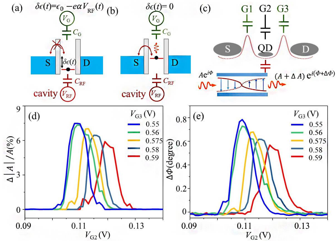
图5.4 (a) 谐振腔的传输线之间电磁场会在量子点的源漏偏置电压上产生电势震荡 V_{\text{RF}}(t) , 也随之影响量子点和源漏电极之间的电势能差 \delta\epsilon(t) = \epsilon_0 - e\alpha V_{\text{RF}}(t) 。 (b) 在库仑谐振区域, \delta\epsilon(t)=0 , 空穴在量子点和源电极/漏电极之间隧穿。 (c) 在固定 G_2 时, 调节 G_1 和 G_3 会改变空穴的隧穿。谐振腔的幅值和相位信号对于隧穿率的变化有灵敏的反应。 (d-e) 调节势垒电极的电压 V_{G3} , 从而调节隧穿率时, 对应的相位和幅值变化的库仑峰。
