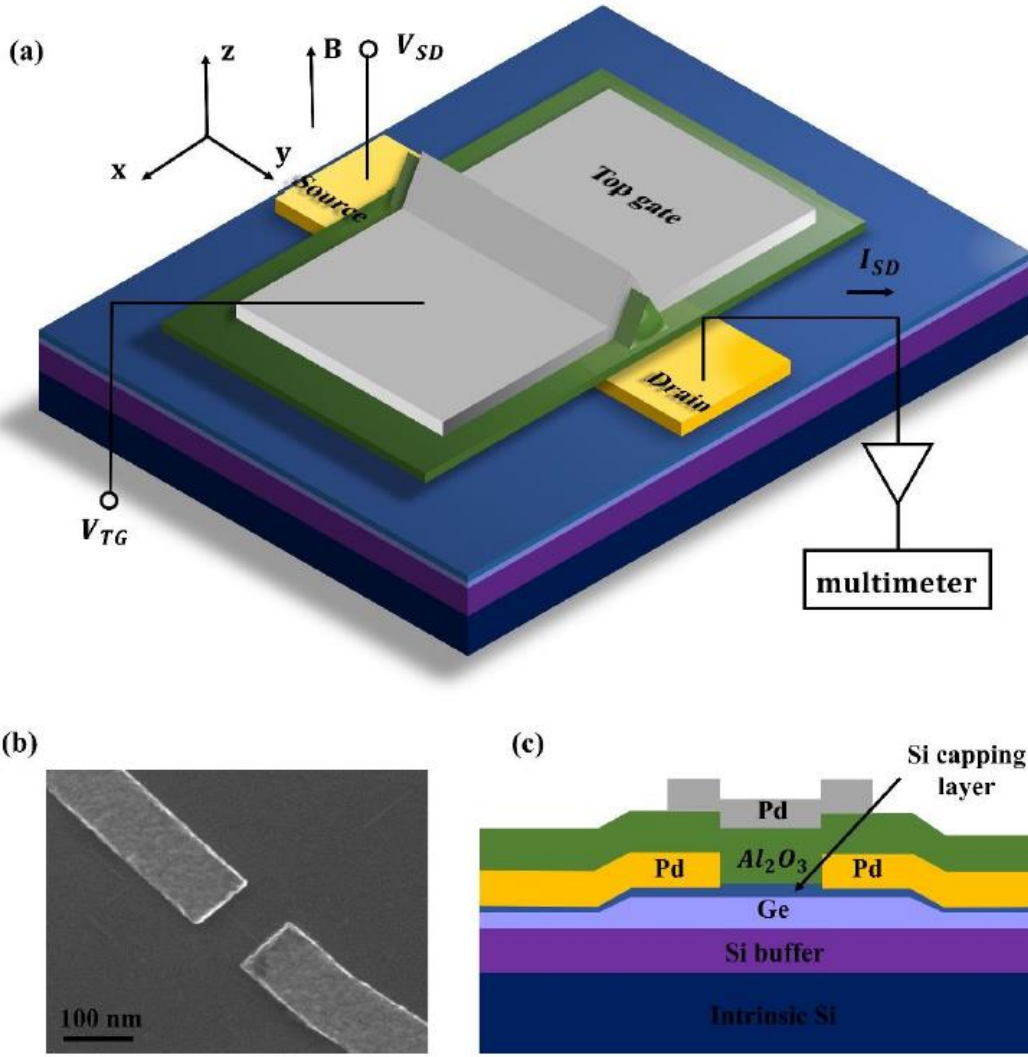
图 3.1 (a) 锗硅自组织纳米线的基片以及量子点的电极三维示意图。(b) 自组织纳米线和源漏电极的扫描电子显微镜照片。(c) 基片和量子点电极的横截面图。自下而上分别是本征硅，硅缓冲层，锗层和硅包覆层以及硅自然氧化层。
