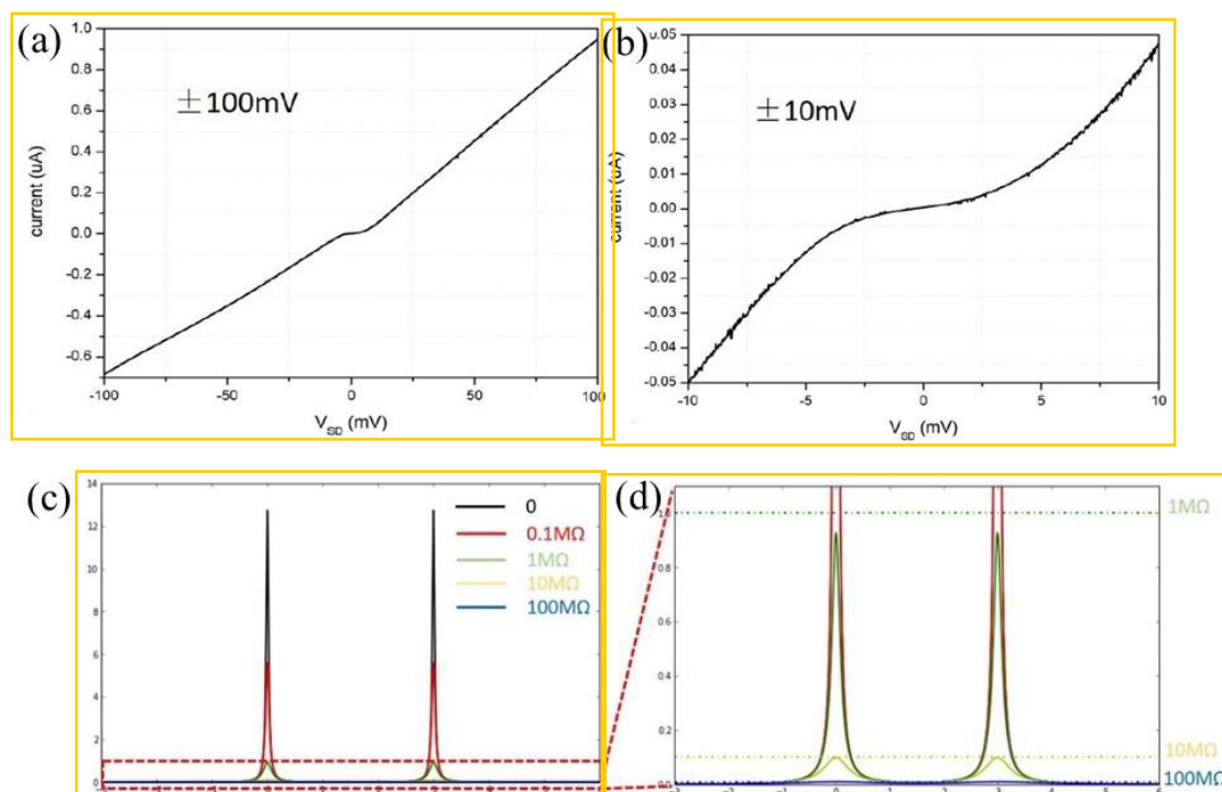
图 3.4 (a) 在 4.2\text{ K} 液氮温度下， -100\text{ mV} 到 100\text{ mV} 的 I-V 特性曲线。在大的偏置电压下，进入源漏电极费米面能级差窗口量子点能级很多，导电通道很多，I-V 特性曲线近似线性。(b) -10\text{ mV} 到 10\text{ mV} 的 I-V 特性曲线。参与导电的量子点能级变小，电导也变小，I-V 特性曲线变得平缓。在更低的温度下，电流呈现台阶状变化，量子特性显现。(c) 在量子点上
