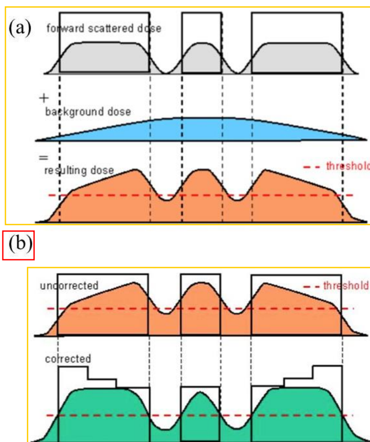
图 2.6 (a) 曝光图案以相同的曝光剂量进行曝光产生邻近效应, 纳米级图案出现变形。(b) 进行邻近效应修正后, 曝光图案的修正剂量。
