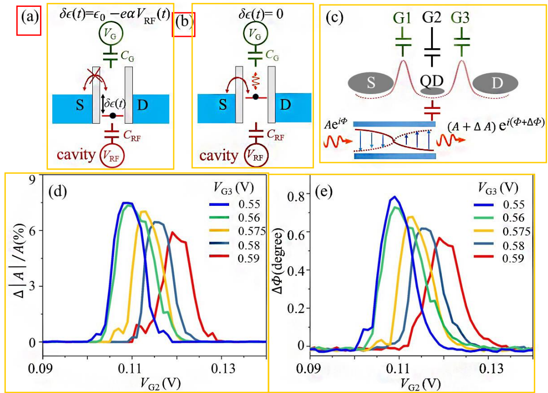
图5.4 (a) 谐振腔的传输线之间电磁场会在量子点的源漏偏置电压上产生电势震荡 V_{\text{RF}}(t) , 也随之影响量子点和源漏电极之间的电势能差 \delta\epsilon(t) = \epsilon_0 - e\alpha V_{\text{RF}}(t) 。 (b) 在库仑谐振区域 \delta\epsilon(t)=0 , 空穴在量子点和源电极/漏电极之间隧穿。 (c) 在固定 G_2 时, 调节 G_1 和 G_3 会改变空穴的隧穿。谐振腔的幅值和相位信号对于隧穿率的变化有灵敏的反应。 (d-e) 调节势垒电极的电压 V_{G_3} , 从而调节隧穿率时, 对应的相位和幅值变化的库仑峰。
