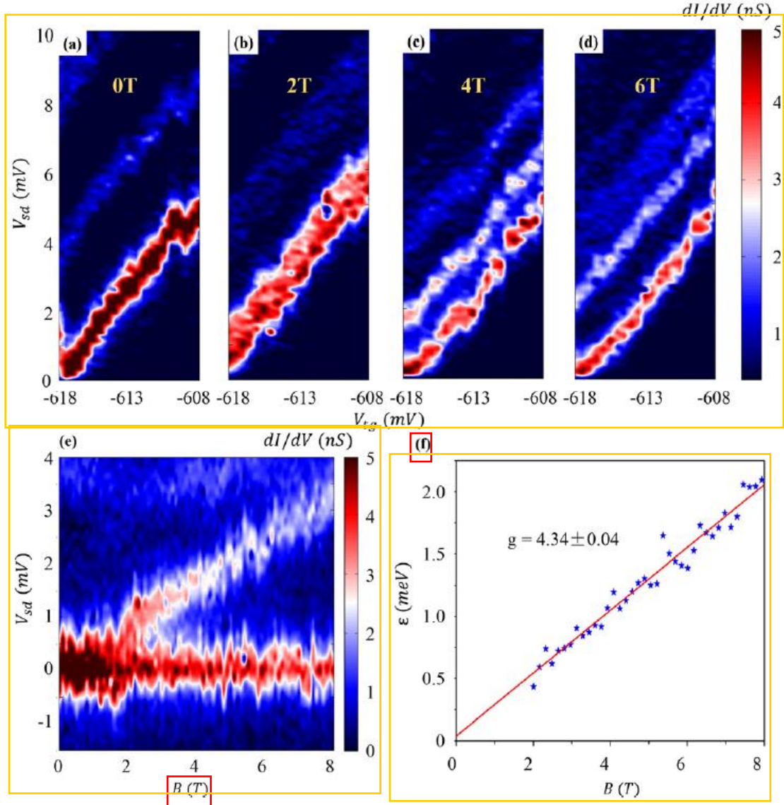
图 3.9 (a-d) 分别在 0T, 2T, 4T 和 6T 垂直磁场下，能级的塞曼劈裂。在垂直磁场下，能级分裂成两个能级。(e) 随着磁场强度的变大，分裂的能级间距逐渐变大。(f) 劈裂能级间距随着磁场的变化。
