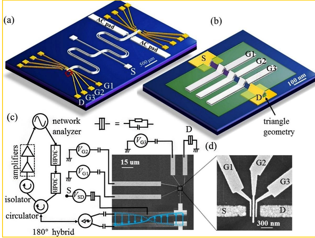
图5.1 (a) 量子点和谐振腔复合结构的三维示意图。谐振腔由两个超导传输线组成，并通过AC板连接到微波的输入和输出端口。一个量子点位于红色矩形框区域。(b) 锗硅自组织纳米线量子点的结构三维示意图，由源漏电极和三个顶栅极以及一层绝缘层构成。图中可以看出锗硅自组织纳米线的三角形横截面。(c) 复合结构的直流输运测量和微波测量电路系统。两个超导传输线上的差分微波信号构建了稳定的电磁场。(d) 单量子点的扫描电子显微镜照片。
