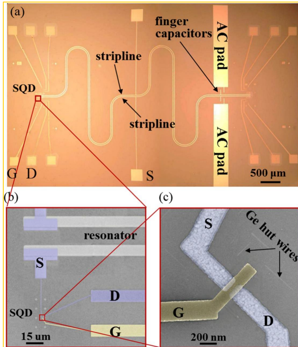
图 4.1 (a) 微波谐振腔和四个量子点的复合结构的光学显微镜照片。红色矩形是其中的一个单量子点所在区域。(b) 量子点通过源电极与微波腔耦合的扫描电镜照片。(c) 单量子点结构的扫描电镜照片。
