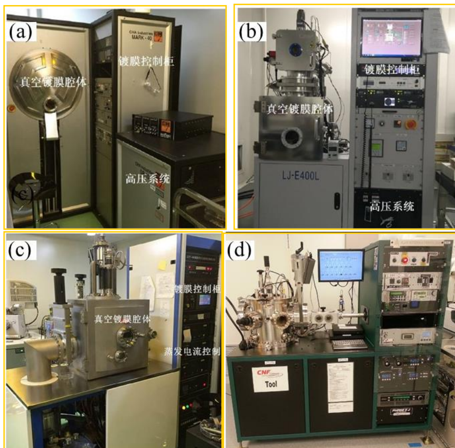
图 2.9 (a-b) 电子束蒸发镀膜机。(c) 热蒸发镀膜机。(d) 磁控溅射镀膜机。
