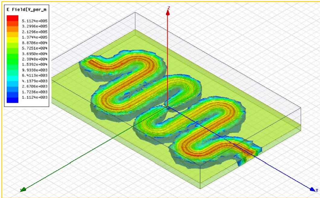
图 4.3 反射式超导微波谐振腔谐振器部分设计和仿真。利用 HESS 软件对谐振器的电磁场模拟。可以看出电磁场主要集中在两根超导传输线之间。在波腹的位置电磁场的强度最大，在波结的位置电磁场强度几乎为零。
