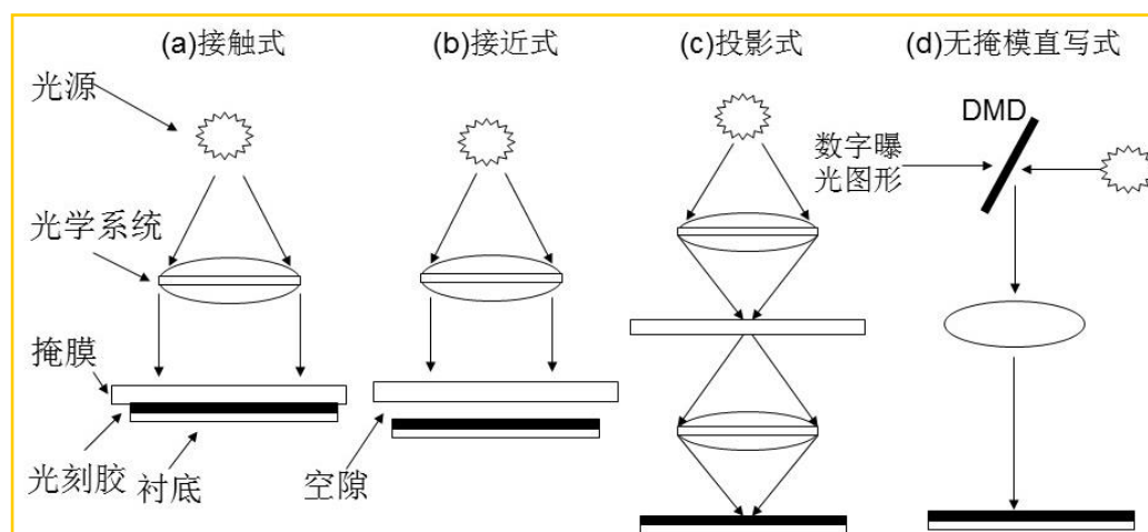
图 2.3 (a) 接触式光刻机。(b) 接近式光刻机。(c) 步进可重复式光刻机。(d) 无掩膜激光直写。图片来源于河北工业大学微电子研究所课件。
