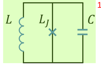
图 1.4 超导量子比特的一般等效电路模型。 2
