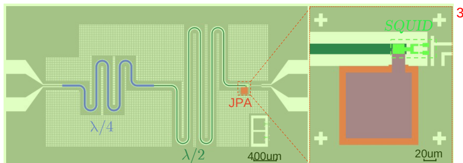
图 4.16 基于片上阻抗变换的 IMPA 的芯片设计版图。 4
