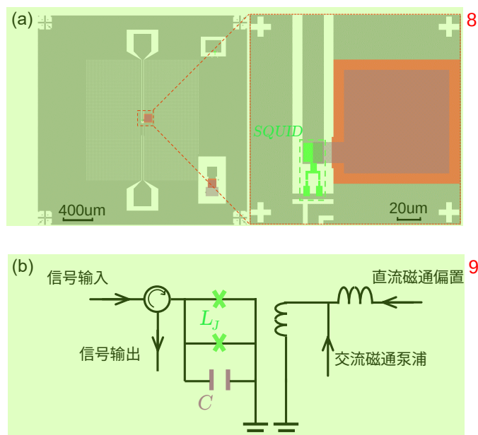
图 4.3 JPA 芯片设计版图 (a) 与它的等效电路图 (b)。版图中灰色代表第一层结构；红色 8 为第二层，代表电容介质层；紫色为第三层，代表电容上级板；绿色为第四层，代表 SQUID 环路（绿色虚线方框）。版图右上角和右下角分别有 SQUID 和电容测试结构，用于常温下的参数表征测试。 10
