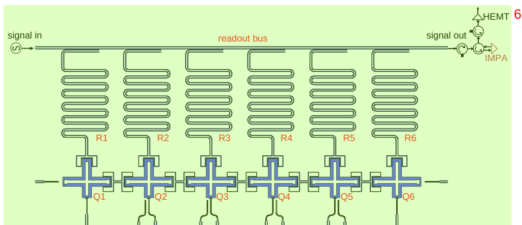
图 5.4 实验中使用的六比特芯片的核心结构的设计版图以及读取电路的关键部分示意图。
