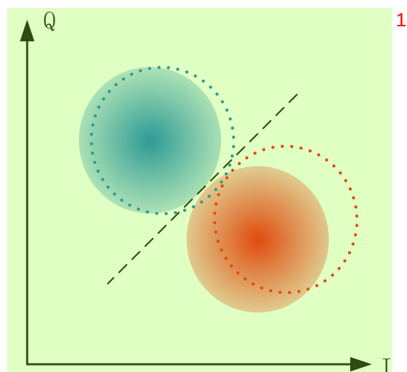
图 5.5 一个两比特体系中 IQ 圆斑偏移的示意图。两个实心圆表示 Q_3 处在 |0\rangle 态时 Q_4 的两个 IQ 圆斑，蓝色代表 |0\rangle 态，红色则代表 |1\rangle 态。黑色虚线表示此时的最佳二分类直线。两个虚线圆表示 Q_3 处在 |1\rangle 态时 Q_4 的两个 IQ 圆斑，由于与 Q_3 处在 |0\rangle 态时 Q_4 的两个 IQ 圆斑有明显的偏移，原来的最佳的分类线此时将不再适用。
