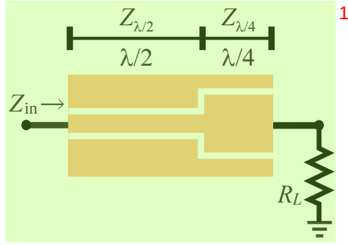
图 4.8 共面波导阻抗变换器示意图。
