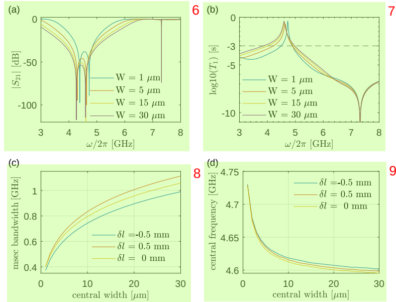
图 3.6 滤波器的中央导带线线宽 W 对结果的影响图。(a) W 取不同值时的 S_{21} 幅值谱。(b) W 取不同值时根据仿真结果计算的量子比特 T_1 ，其中虚线表示 T_1 = 1 \text{ ms} 。(c) \delta l 取不同值时分别扫描 W 得到的毫秒带宽与 W 的变化关系，纵轴毫秒带宽表示从图 (b) 中提取的 T_1 \geq 1 \text{ ms} 时的带宽。(d) 滤波器中心保护频率与 W 的变化关系。
