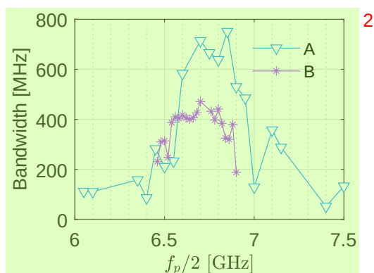
图 4.22 实验观测到的 IMPA 工作频率的可调性。样品 A 和 B 分别代表片上和片外阻抗变换方案下的 IMPA。
