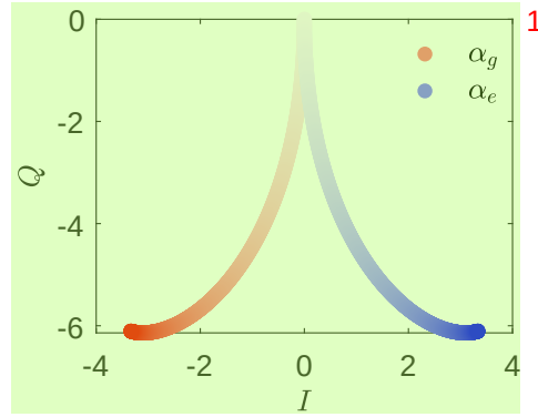
图 2.6 典型的腔光场在 I-Q 平面的演化轨迹图，线条颜色深度的增加代表演化时间的增加。
