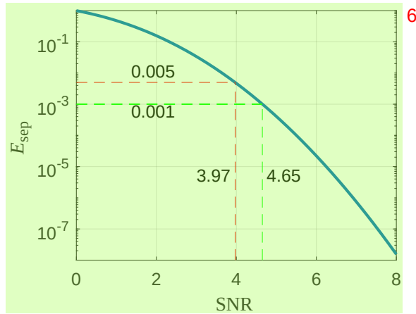
图 2.5 态分离错误率随信噪比的变化关系。图中红色和绿色虚线分别指示 E_{sep} 为 0.005 和 0.001 时对应的 SNR 的大小。
