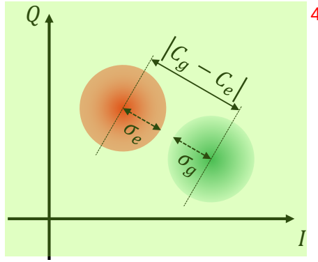
图 2.4 理想情况比特处于基态和激发态下对应的读取信号的两个高斯圆斑示意图。 5
