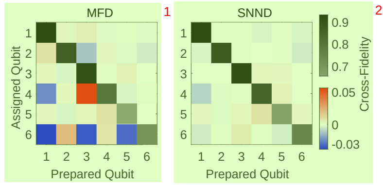
图 5.11 MFD 的交叉保真度矩阵以及 SNND 的交叉保真度矩阵。 3
