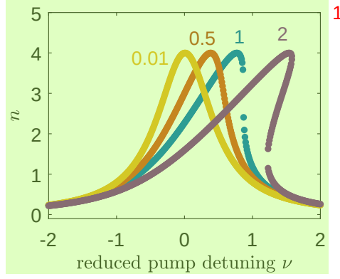
图 4.2 约化后的稳态光子数与约化后的泵浦失谐 \nu 以及实际驱动强度相关的量 \xi 之间的关系。 \xi/\xi_{\text{crit}} = 0.01, 0.5, 1, 2 分别对应黄色、红色、蓝色、紫色线。
