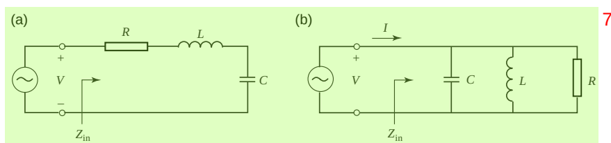
图 3.1 (a) 串联 RLC 电路。(b) 并联 RLC 电路。 8
