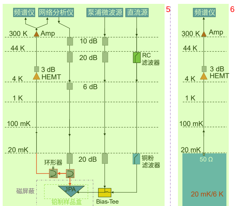
图 4.5 左侧：测量系统线路连接与配置图，JPA 的反射信号经过两级环形器之后先经低温 HEMT 放大再到室温经过室温放大器放大之后输入到频谱仪或网络分析仪。红色线路——包括两级环形器在内，表示 JPA 信号端口与 20 mK 冷盘之间存在一定的插损。右侧：冷 (20 mK) / 热 (6 K) 负载法测量低温 HEMT 噪声温度的线路连接图，HEMT 的负载为 20 mK 盘上连接的标准 50 \Omega 负载器。
