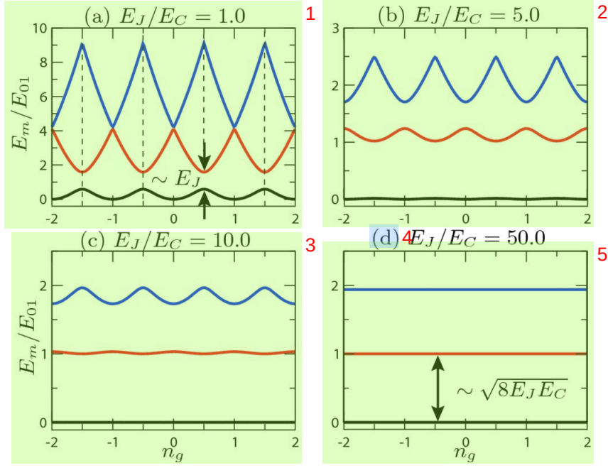
图 1.5 不同参数条件下的电荷量子比特的本征能级图，图片引自文献 [57] 。6
