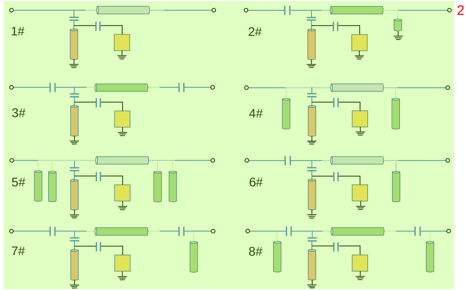
图 3.10 8 种不同设计的 Purcell 滤波器等效电路图，其中 1# 没有 Purcell 滤波器。图中橙色代表读取谐振腔，黄色代表量子比特，绿色代表 Purcell 滤波器。 3
