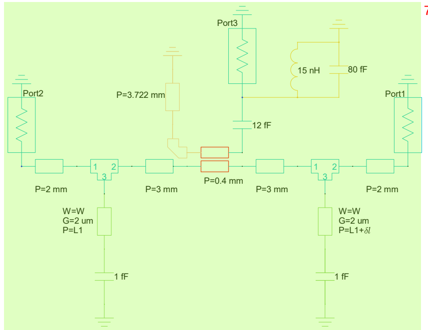
图 3.5 Purcell 滤波器的仿真电路图。黄色部分表示量子比特，橙色表示读取谐振腔，红色部分是谐振腔与读取总线的耦合部分，绿色部分表示滤波器。仿真使用的衬底为理想的本征硅，P 表示各段传输线的长度，G 表示传输线中央导带线距离地平面的距离，对于所有传输线 G=2 \mu\text{m} ，W 表示滤波器的中央导带线线宽，对于读取总线以及谐振腔，中央导带线线宽为 3.2 \mu\text{m} ，从而满足 50 \Omega 的阻抗匹配条件。
