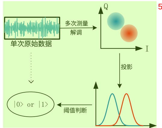
图 5.3 利用投影阈值法构建态分类器过程示意图。
