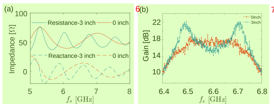
图 4.20 环形器端口到阻抗变换器之间的连接线长度对环境阻抗的影响 (a) 以及对 IMPA 增益的影响 (b)。测量 (a) 图时环形器的另外两个端口接标准 50 Ω 负载，因此阻抗曲线较为平滑。
