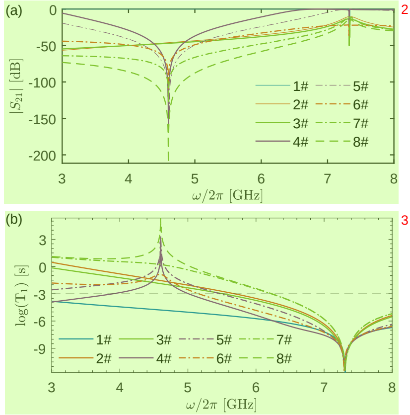
图 3.11 几种不同 Purcell 滤波器的设计仿真结果的对比。(a) 输入输出 |S_{21}| 幅值谱。(b) 根据 Purcell 耗散率计算的 T_1 上限随比特频率的变化关系。
