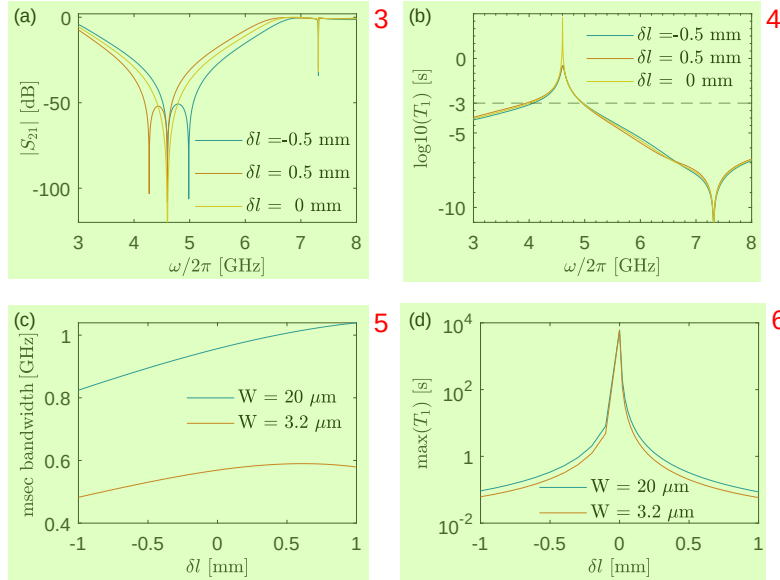
图 3.7 两个 \lambda/4 滤波器的长度差值 \delta l 对结果的影响图。(a) \delta l 取不同值时的 S_{21} 幅值谱。(b) \delta l 取不同值时根据仿真结果计算的量子比特 T_1 ，其中虚线表示 T_1 = 1 \text{ ms} 。(c) W 取不同值时分别扫描 \delta l 得到的毫秒带宽与 \delta l 的变化关系。(d) 滤波器中心保护频率出的 T_1 与 \delta l 的变化关系。
