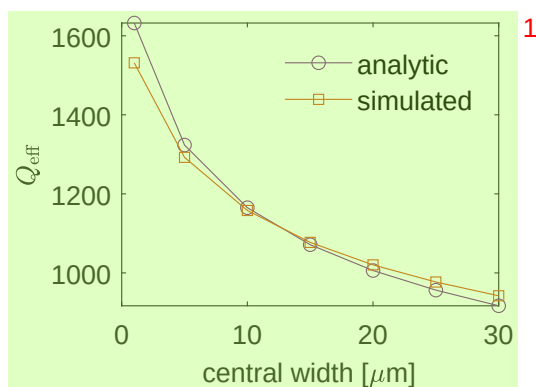
图 3.8 Purcell 滤波器对读取谐振腔的有效外部耦合 Q 值 Q_{\text{eff}} 的影响。 2
