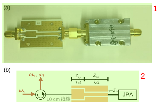
图 4.14 JPA 外接阻抗变换器样品图 (a) 及其等效电路和信号流图 (b)。阻抗变换器与环形器之间一般用约 10 cm 长的低温同轴电缆相连接。
