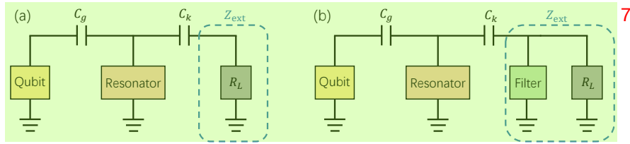
图 3.3 (a) 传统的不带滤波器的 CQED 等效电路图。(b) 带有 Purcell 滤波器的 CQED 7 等效电路图。两者的差别由蓝色虚线框内的外部阻抗 Z_{\text{ext}} 表示。 8
