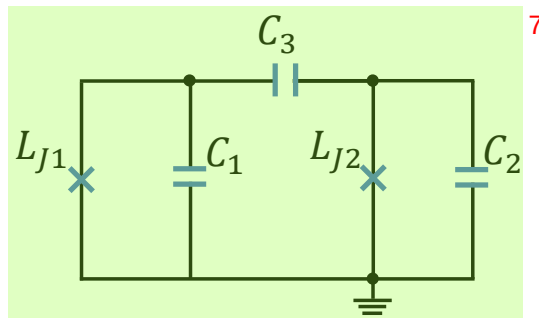
图 1.7 两个 transmon 量子比特通过电容耦合的等效电路图。
