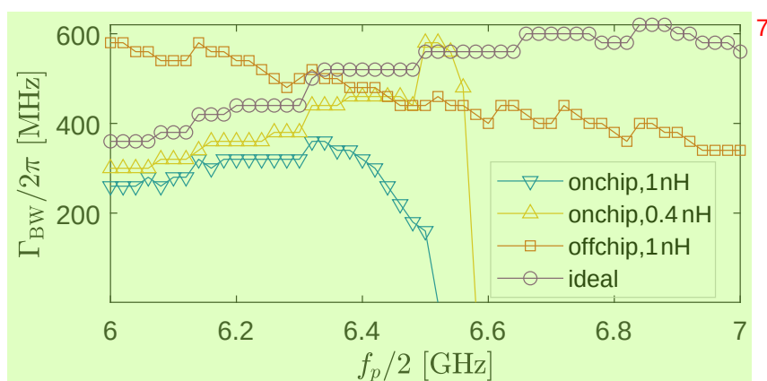
图 4.17 绑线电感对于片外和片上阻抗变换方案的影响。理想条件为环境阻抗 R_L = 50 \Omega ， 8 计算中采用的设计参数为 \omega_l/2\pi = 6.5 \text{ GHz} ， C = 3 \text{ pF} ， Z_{\lambda/2} = 60 \Omega ， Z_{\lambda/4} = 39.2 \Omega 。
