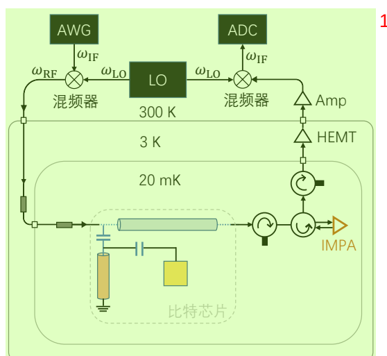
图 5.1 超导量子比特读取线路示意图。
