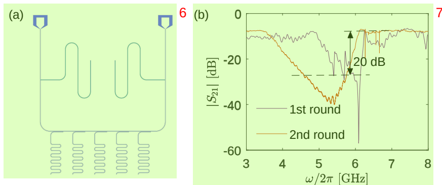
图 3.9 (a) Purcell 滤波器样品设计版图, 绿色部分表示开路 \lambda/4 滤波器。(b) 低温测量结果, 黑色箭头代表比特频率范围处与谐振腔频率范围处的隔离度, 20 dB 隔离度的带宽超过 1 GHz 以上。 8
