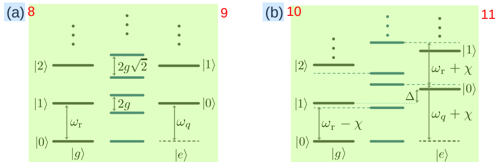
图 2.2 (a) JC 模型共振条件下的能级示意图。(b) JC 模型色散耦合条件下的能级示意图。黑线表示系统无耦合时的本征能级，蓝线表示系统耦合之后缀饰态本征能级。图片引自文献 [19] 。 12
