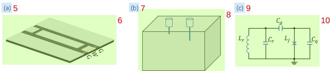
图 2.1 （a）平面共面波导谐振腔结构示意图。灰色为绝缘衬底，浅色为超导金属。中央导带线线宽为 W ，距离两边的地平面的距离为 G 。（b）3D 谐振腔示意图，微波信号通过一个端口耦合到谐振腔内部，通过另一个端口可以探测到谐振腔内部的光场信号。（c）谐振腔与超导量子比特通过电容耦合的等效电路图。 11
