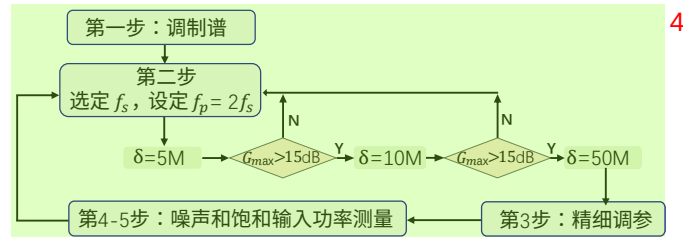
图 4.6 JPA 低温测试表征流程图。5
