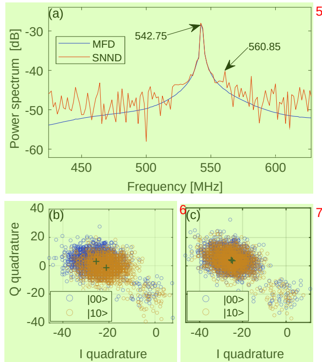
图 5.12 (a) 解调系数的功率谱，蓝线代表 MFD，在这条线上只有一个关于目标比特中频频率的信号峰。红色代表 SNND，可以看到，除了目标比特自身的频率信号峰之外，还有一个信号峰的频率刚好等于 Q3 的中频频率。(b) 使用 MFD 的解调系数获得的 IQ 圆斑以及 (c) 使用 SNND 的解调系数获得的 IQ 圆斑，其中的态表示 |Q3, Q4\rangle ，黑色的十字交叉记号代表每个圆斑的中心点，可以发现采用 MFD 方案时，随着 Q3 状态的改变，圆斑发生了偏移，而在 SNND 中则没有这种现象。 8
