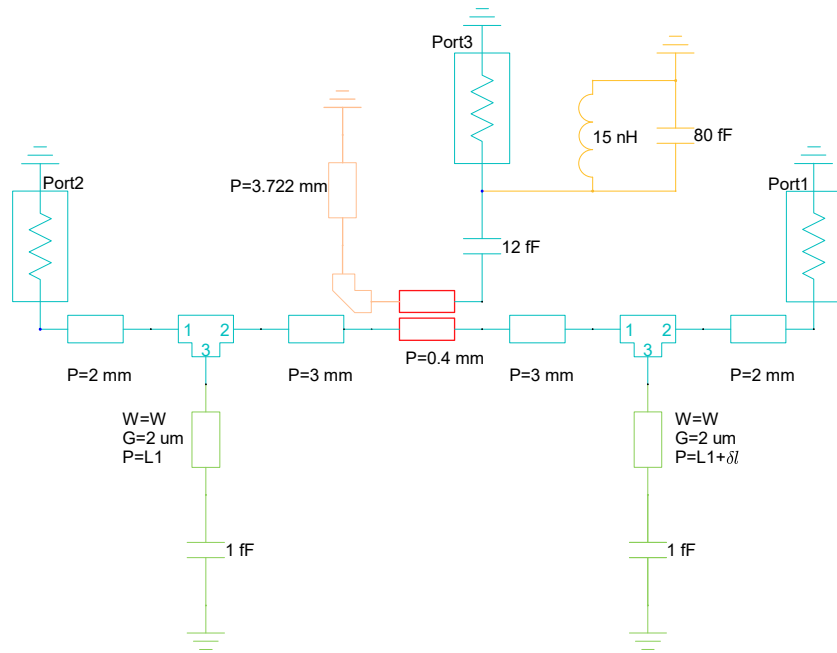
图 3.5 Purcell 滤波器的仿真电路图。黄色部分表示量子比特，橙色表示读取谐振腔，红色部分是谐振腔与读取总线的耦合部分，绿色部分表示滤波器。仿真使用的衬底为理想的本征硅， P 表示各段传输线的长度， G 表示传输线中央导带线距离地平面的距离，对于所有传输线 G=2\text{ }\mu\text{m} ， W 表示滤波器的中央导带线线宽，对于读取总线以及谐振腔，中央导带线线宽为 3.2\text{ }\mu\text{m} ，从而满足 50\text{ }\Omega 的阻抗匹配条件。
