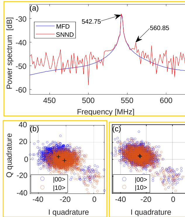
图 5.12 (a) 解调系数的功率谱，蓝线代表 MFD，在这条线上只有一个关于目标比特中频频率的信号峰。红色代表 SNND，可以看到，除了目标比特自身的频率信号峰之外，还有一个信号峰的频率刚好等于 Q3 的中频频率。(b) 使用 MFD 的解调系数获得的 IO 圆斑以及 (c) 使用 SNND 的解调系数获得的 IO 圆斑，其中的态表示 |Q3, Q4\rangle ，黑色的十字交叉记号代表每个圆斑的中心点，可以发现采用 MFD 方案时，随着 Q3 状态的改变，圆斑发生了偏移，而在 SNND 中则没有这种现象。
