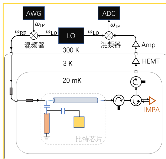
图 5.1 超导量子比特读取线路示意图。
