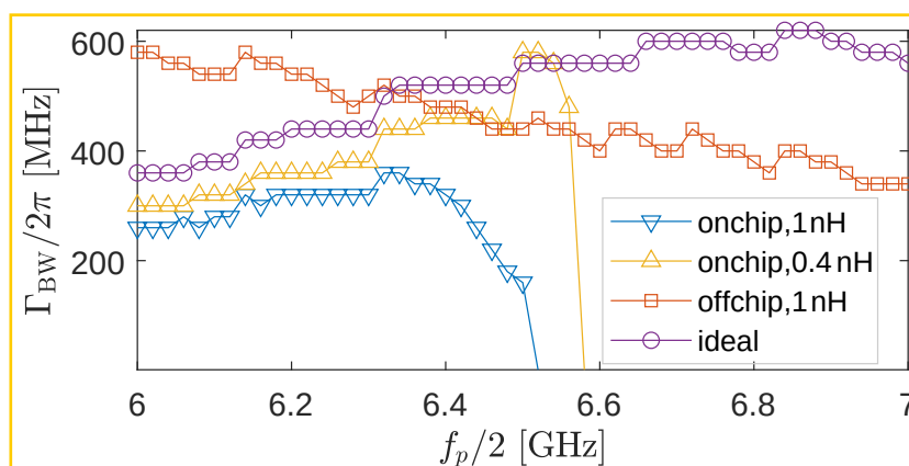
图 4.17 绑线电感对于片外和片上阻抗变换方案的影响。理想条件为环境阻抗 R_f = 50 \Omega ，计算中采用的设计参数为 \omega_p/2\pi = 6.5 \text{ GHz} ， C = 3 \text{ pF} ， Z_{\lambda/2} = 60 \Omega ， Z_{\lambda/4} = 39.2 \Omega 。
