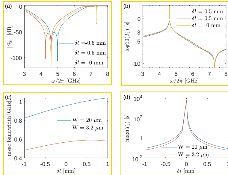
图 3.7 两个 \lambda/4 滤波器的长度差值 \delta l 对结果的影响图。(a) \delta l 取不同值时的 |S_{21}| 幅值谱。(b) \delta l 取不同值时根据仿真结果计算的量子比特 T_1 ，其中虚线表示 T_1 = 1 \text{ ms} 。(c) W 取不同值时分别扫描 \delta l 得到的毫秒带宽与 \delta l 的变化关系。(d) 滤波器中心保护频率出的 T_1 与 \delta l 的变化关系。
