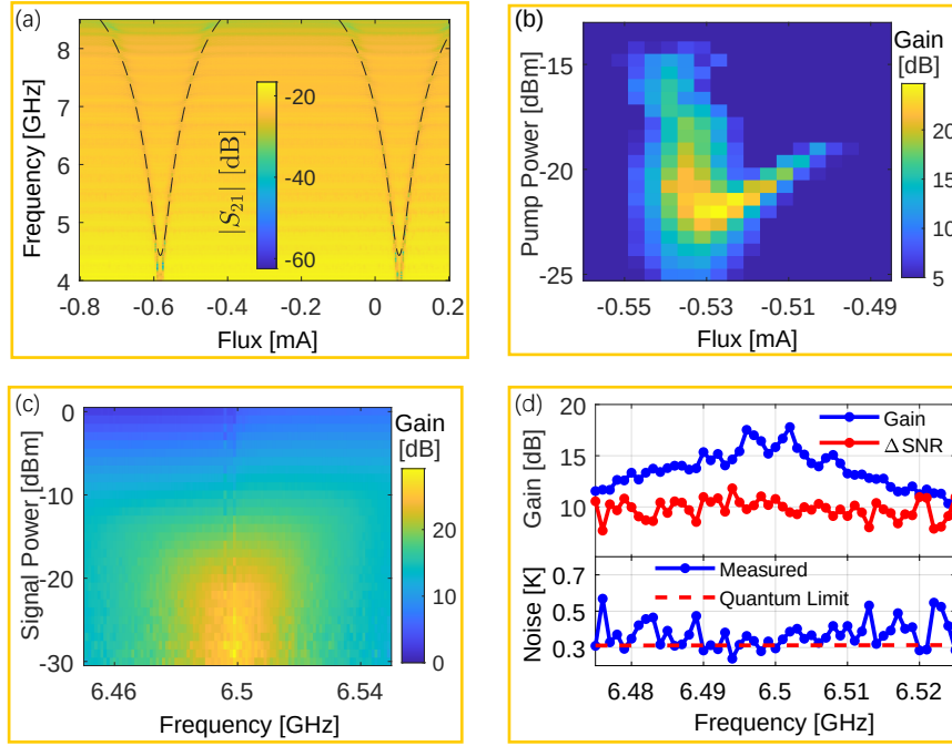
图 4.7 JPA 实验测量结果图。(a) JPA 的直流调制谱图，谐振频率随着直流偏置磁通周期性变化，且可调范围大于 4 GHz~8 GHz。图中黑色虚线为拟合曲线。(b) \delta = 10 MHz 时的信号增益与泵浦功率和直流偏置磁通的变化关系。(c) 信号增益随信号输入功率的变化关系，随着输入功率增大，增益逐渐减小，输入线上的总衰减量为 -101 dB。(d) \Delta SNR 法测到的系统噪声温度。
