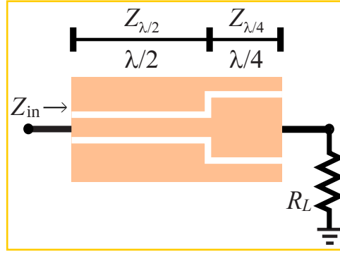
图 4.8 共面波导阻抗变换器示意图。
