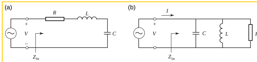
图 3.1 (a) 串联 RLC 电路。(b) 并联 RLC 电路。
