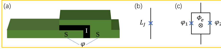
图 1.3 (a) 三明治结构的约瑟夫森结结构示意图。(b) 约瑟夫森结的电路符号。(c) 两个约瑟夫森结并联构成超导量子干涉仪 (SQUID)。
