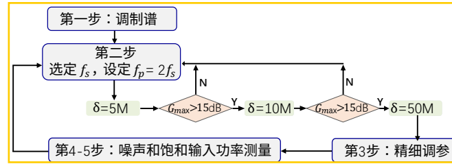
图 4.6 JPA 低温测试表征流程图。
