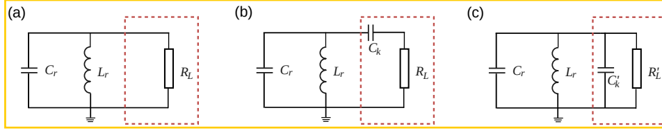
图 3.2 (a) 并联式谐振电路与环境直接耦合。(b) 并联式谐振电路与环境通过电容耦合。(c) 图 (b) 的等效电路。红色虚线框表示耦合电路部分， R_L 为环境阻抗， C_k 为耦合电容。
