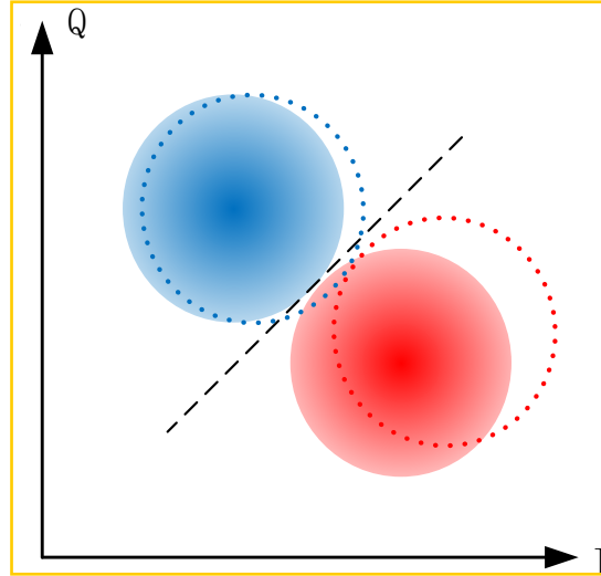
图 5.5 一个两比特体系中 IO 圆斑偏移的示意图。两个实心圆表示 Q3 处在 |0\rangle 态时 Q4 的两个 IO 圆斑，蓝色代表 |0\rangle 态，红色则代表 |1\rangle 态。黑色虚线表示此时的最佳二分类直线。两个虚线圆表示 Q3 处在 |1\rangle 态时 Q4 的两个 IO 圆斑，由于与 Q3 处在 |0\rangle 态时 Q4 的两个 IO 圆斑有明显的偏移，原来的最佳的分类线此时将不再适用。
