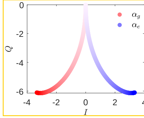
图 2.6 典型的腔光场在 I-O 平面的演化轨迹图，线条颜色深度的增加代表演化时间的增加。
