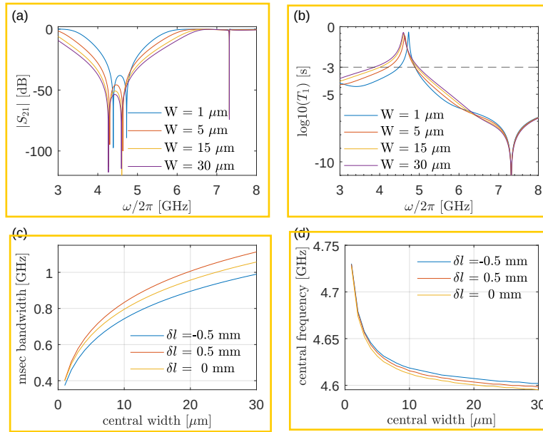
图 3.6 滤波器的中央导带线宽 W 对结果的影响图。(a) W 取不同值时的 |S_{21}| 幅值谱。(b) W 取不同值时根据仿真结果计算的量子比特 T_1 ，其中虚线表示 T_1 = 1 \text{ ms} 。(c) \delta l 取不同值时分别扫描 W 得到的毫秒带宽与 W 的变化关系，纵轴毫秒带宽表示从图 (b) 中提取的 T_1 \geq 1 \text{ ms} 时的带宽。(d) 滤波器中心保护频率与 W 的变化关系。
