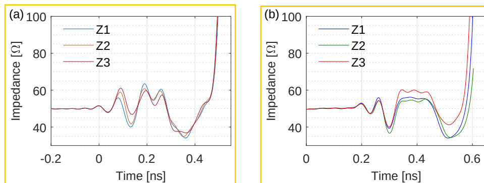
图 4.15 两种使用不同基底制备的片外阻抗变换器的特征阻抗时域测量结果。(a) 第一类基底，其介电常数 \epsilon_r = 3.48 ，0.2 ns 附近为半波长阻抗变换线的阻抗，之后的低谷对应四分之一波长阻抗变换线的特征阻抗。(b) 第二类基底，其介电常数 \epsilon_r = 10.2 ，0.4 ns 附近为半波长阻抗变换线的阻抗，之后的低谷对应四分之一波长阻抗变换线的特征阻抗。Z1、Z2、Z3 代表阻抗参数的不同设计组合编号。
