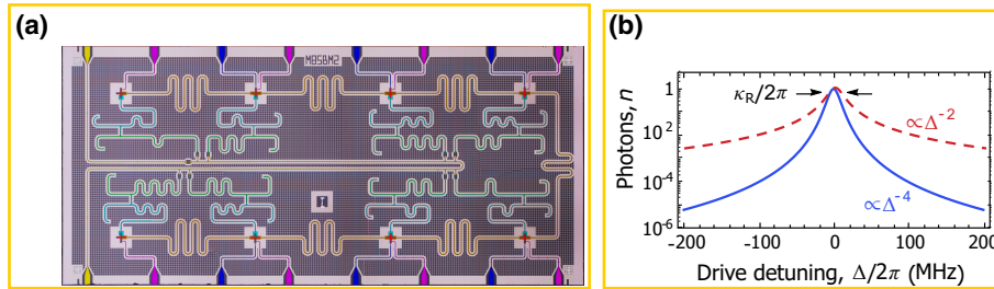
图 5.6 每个读取腔设置独立的 Purcell 滤波器可以有效抑制读取串扰。(a) 样品结构图。(b) 红色虚线表示没有 Purcell 滤波器时谐振腔的激发光子数与驱动频率失谐量的关系，而蓝色实线表示有了独立的 Purcell 滤波器之后的情形。图片引自文献 [6] 。
