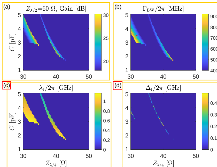
图 4.13 固定 Z_{\lambda/2} = 60\ \Omega ，计算 C 和 Z_{\lambda/4} 对增益和带宽的影响。(a) 满足设计条件前提下计算出来的增益大小。(b) 满足设计条件前提下计算出来的带宽大小，红色小圆点表示正文中提到的设计参数，在这个参数条件下，横向和纵向都有较大的冗余度。(c) 工作点的泵浦强度，决定磁通泵浦的功率大小。(d) 工作点的泵浦失谐，决定 JPA 的谐振频率。由于在满足设计条件的前提下，工作点参数仍然有一定的可调范围，图 (c) 和 (d) 是按照正文中的最大带宽策略计算的工作点泵浦强度和失谐量。
