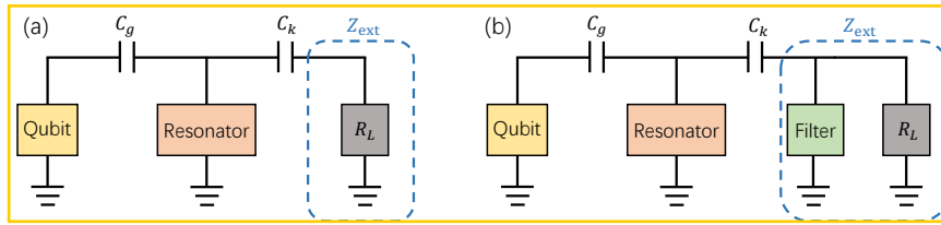
图 3.3 (a) 传统的不带滤波器的 CQED 等效电路图。(b) 带有 Purcell 滤波器的 CQED 等效电路图。两者的差别由蓝色虚线框内的外部阻抗 Z_{\text{ext}} 表示。
